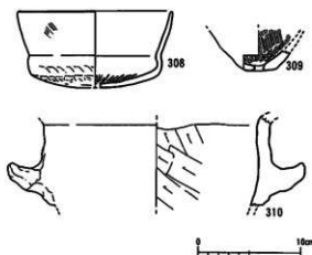
第45図 7号住居跡出土遺物実測図
