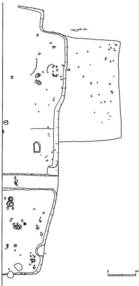
第41图 5・6号住居跡実測图
