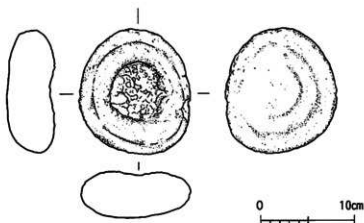
第85図 2号土坑出土遺物実測図②
