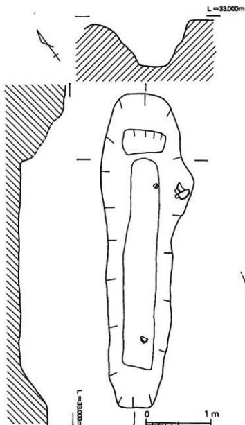
第50図 3号土坑実測図
