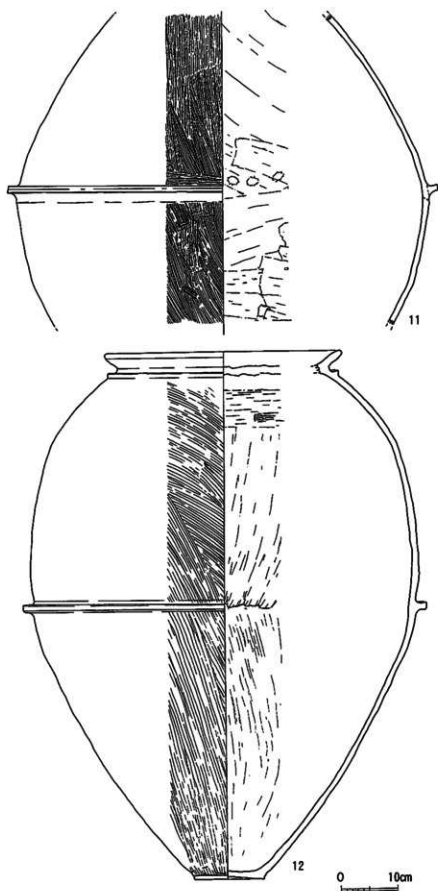
第18图 4号墓棺冥测图（上·下）
