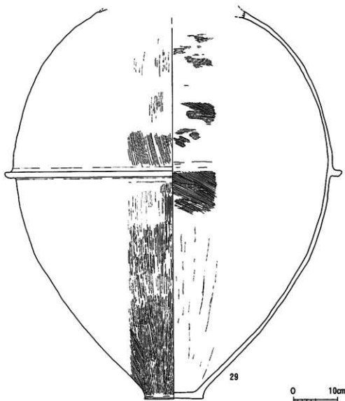
第40図 13号壟下壘実測図
