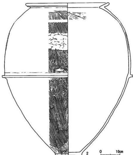
第15図 3号壺棺実測図
