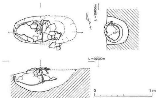
第30図 10号墓棺出土状況実測図
