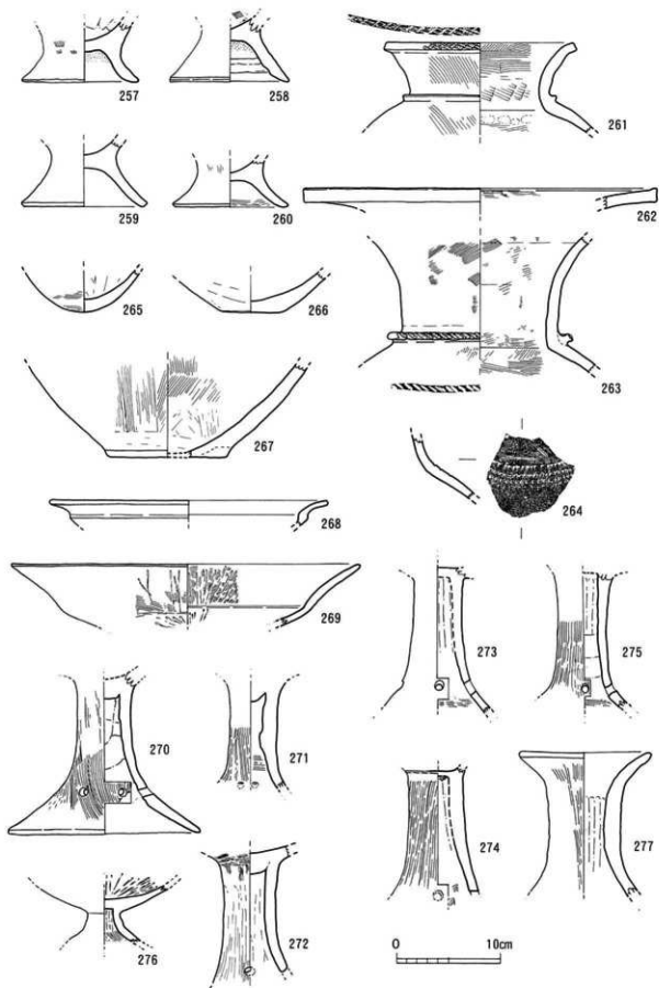
第84图 2号土坑出土遗物实测图①
