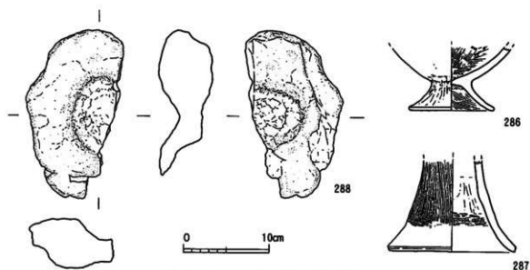
第89图 4号土坑出土文物实测图
