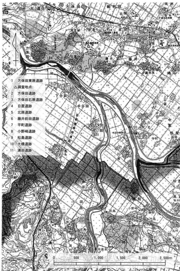
第8図 弥生時代遺跡分布図
