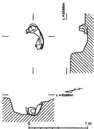
第12図 2号壙棺出土状況実測図
