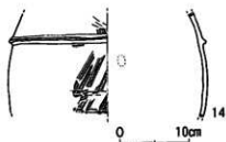
第21図 5号甕棺上甕実測図
