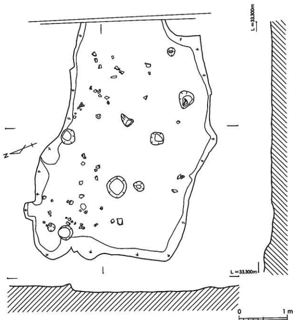
第48図 2号土坑実測図
