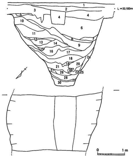
第57図 2号溝実測図 (C-5区) ④
