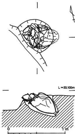
第20図 5号壺棺出土状況実測図
