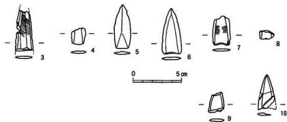
第16图 3号墓出土文物实测图
