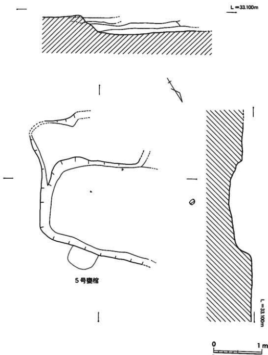
第44図 3号住居跡実測図
