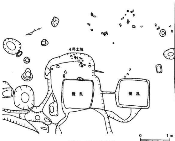
第88图 4号土坑实测图
