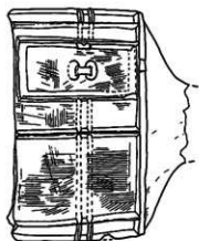
第76图 家形土器实测图
