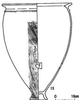
第22図 5号甕棺下甕実測図
