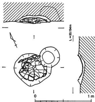
第27図 8号壺棺出土状況実測図
