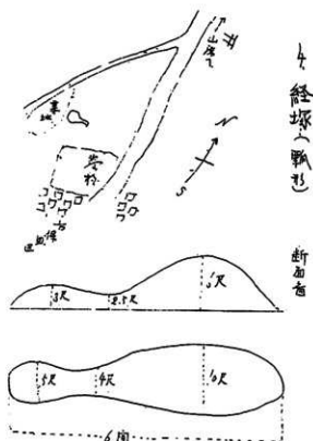
第7図 経塚古墳見取図
