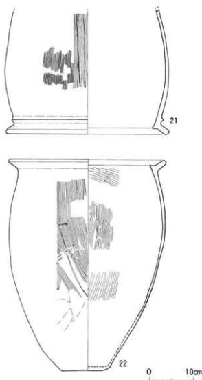
第31図 10号墓棺実測図(上・下)
