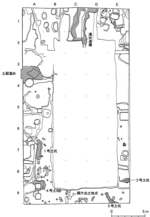
第71図 遺構配置図
