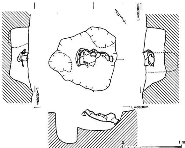
第25図 7号墓出土状況実測図
