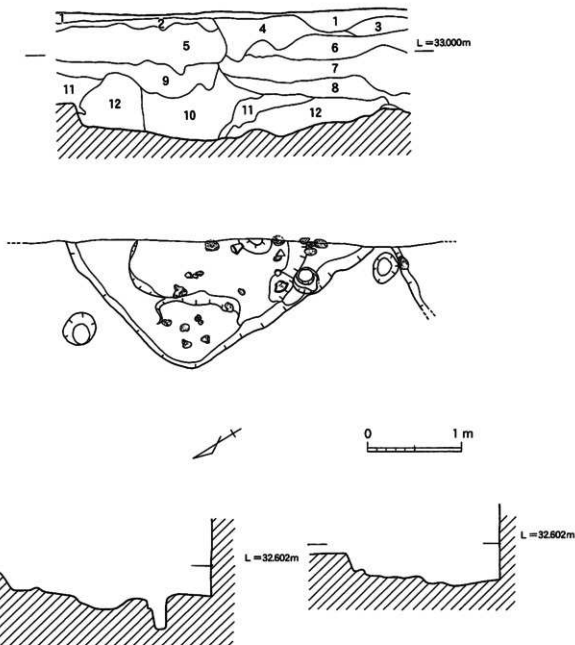
第42図 1号住居跡実測図
