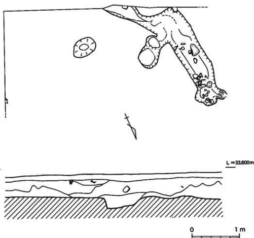
第83图 2号土坑下層・断面实测图
