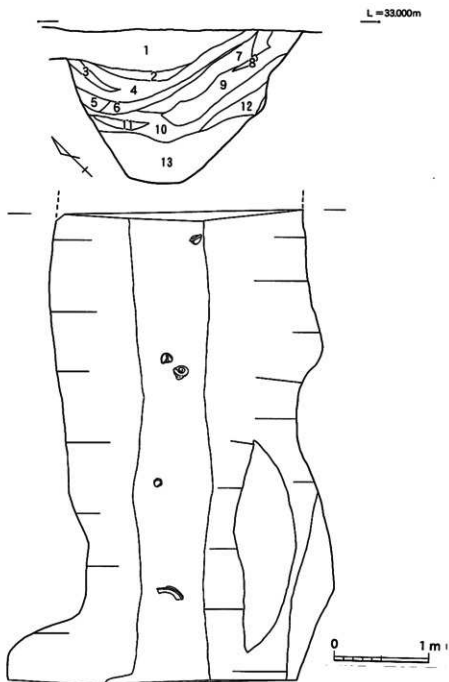
第58図 2号溝実測図 (D・E-4区) ⑤
