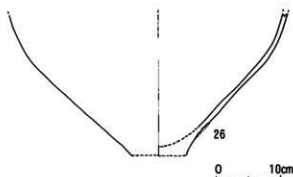
第37図 12号墓実測図
