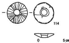
第63図 遺構に伴わない遺物実測図③
