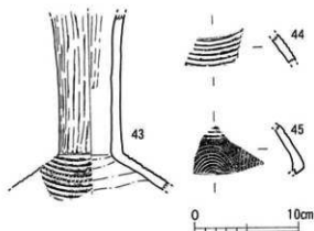
第47図 1号土坑出土遺物実測図
