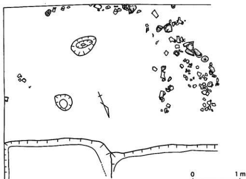
第82图 2号土坑上层实测图
