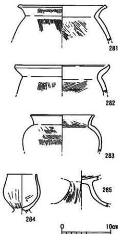
第87図 3号土坑出土遺物実測図
