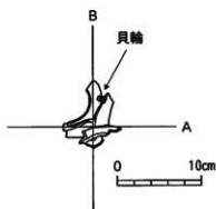
第33図 11号墓棺内貝輪出土状況実測図
