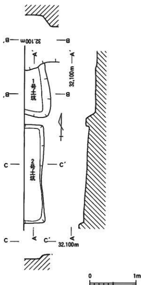
第415图 1号土坑·2号土坑 实测图 (S=1/40)
