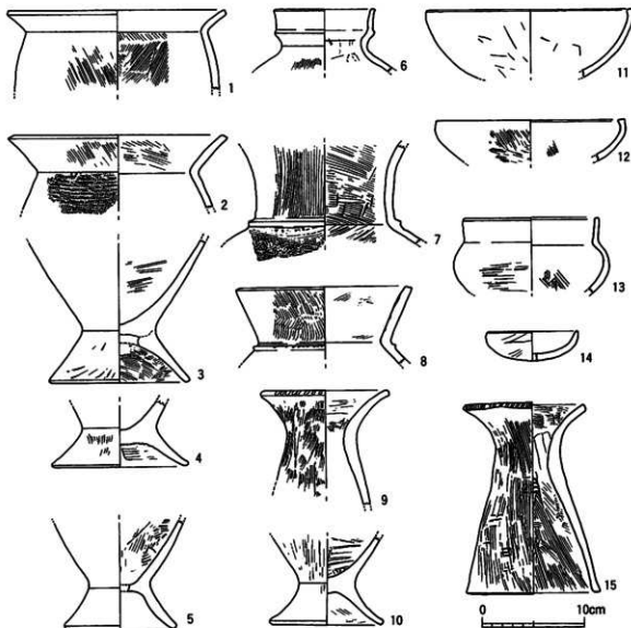
第365図 第2トレンチ 2号溝出土土器実測図
