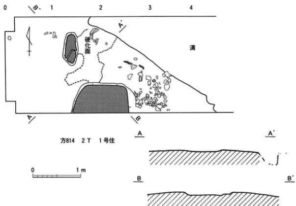
第266図 1号住居跡実測図
