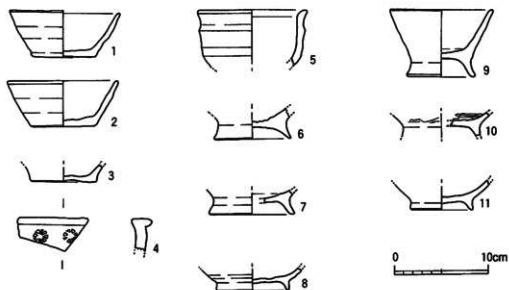
第362図 第1トレンチ土坑出土土器実測図
