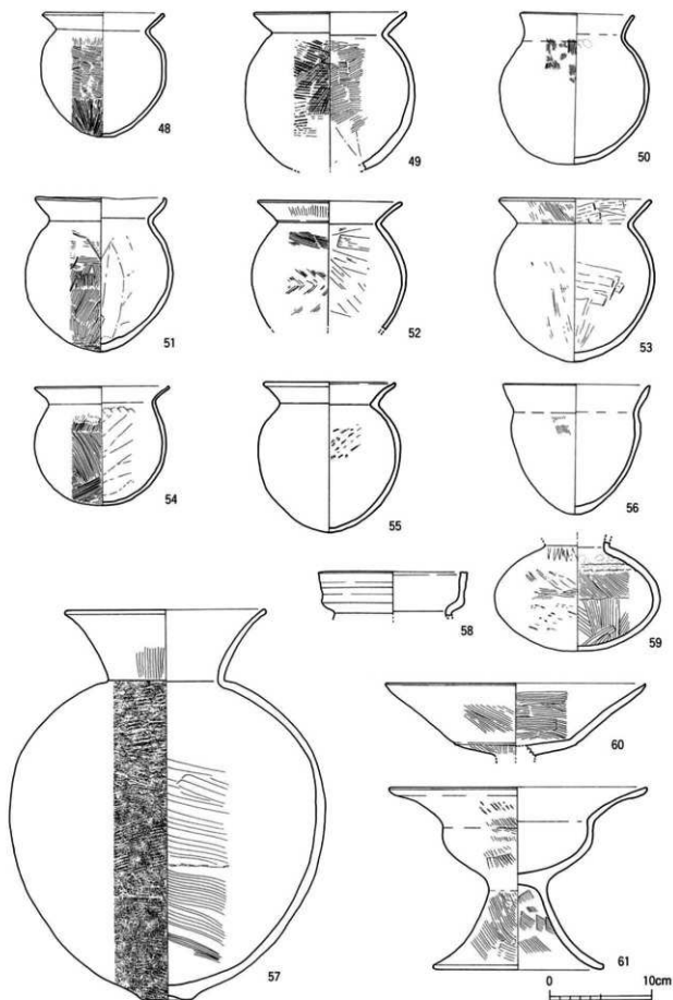
第19图 满(上層)出土土器 実測図② (S=1/4)
