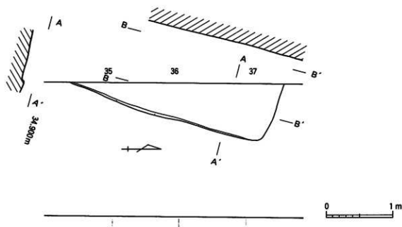
第245図 南北1 T 3号住居跡実測図
