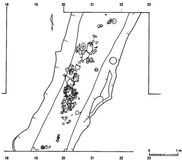
第255図 方268 南北2 T・東西1 T (1号溝) 1号溝実測図
