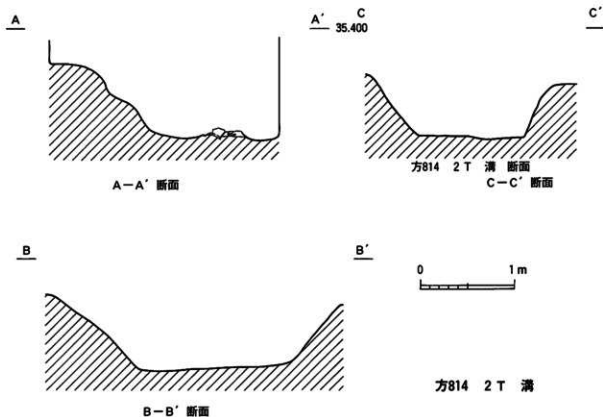
第270図 1・2号溝断面図
