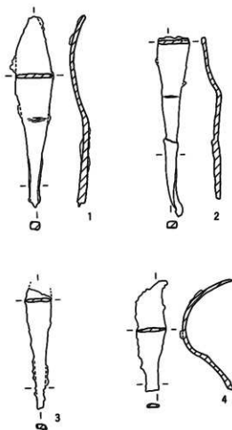
方保田813番地出土鉄器実測図 (S=1/2)
