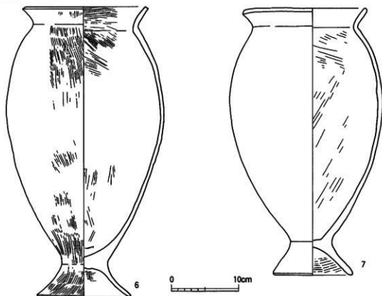
第368図 第2トレンチ3号溝出土土器実測図②(2層)
