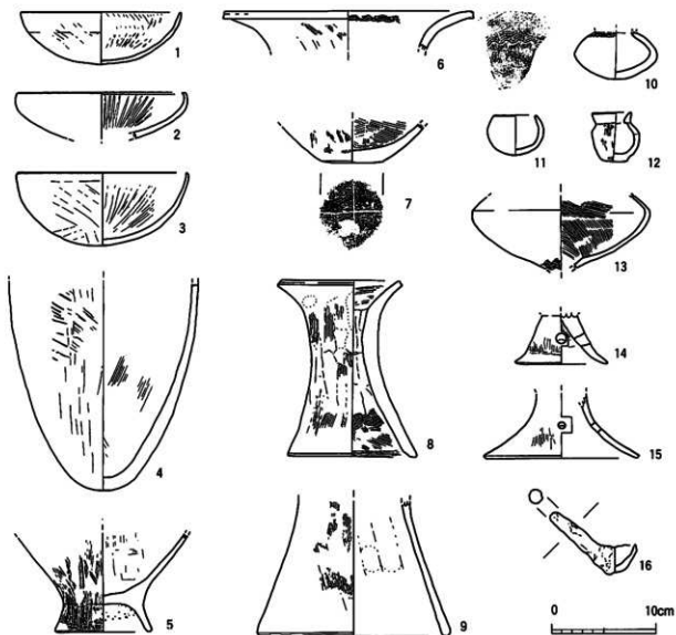
第423図 遺構に伴わない遺物実測図 (S=1/4)
