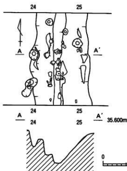
第323図 溝実測図
