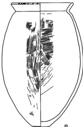
第273図 2号溝出土・遺構に伴わない遺物実測図
