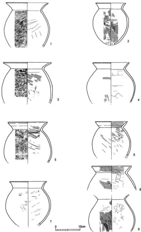
第42图 7号住居跡出土土器実測図①
