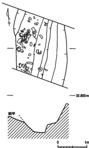
第364図 第2トレンチ 2号溝 実測図 (S=1/40)
