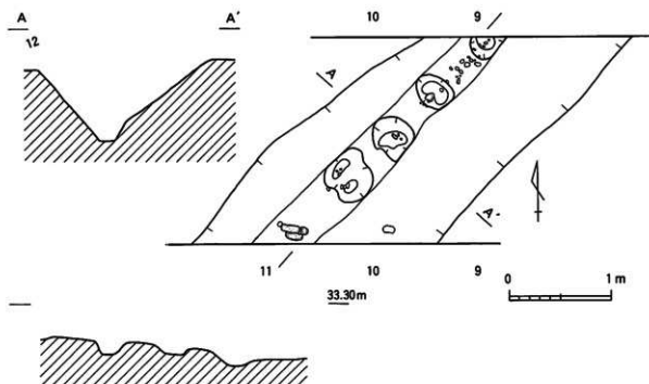
第232図 方268 東西4 T 2号道路実測図
