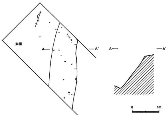
第363図 第2トレンチ 1号溝実測図（S=1/40）
