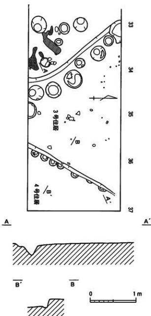
第281図 3・4号住居跡実測図
