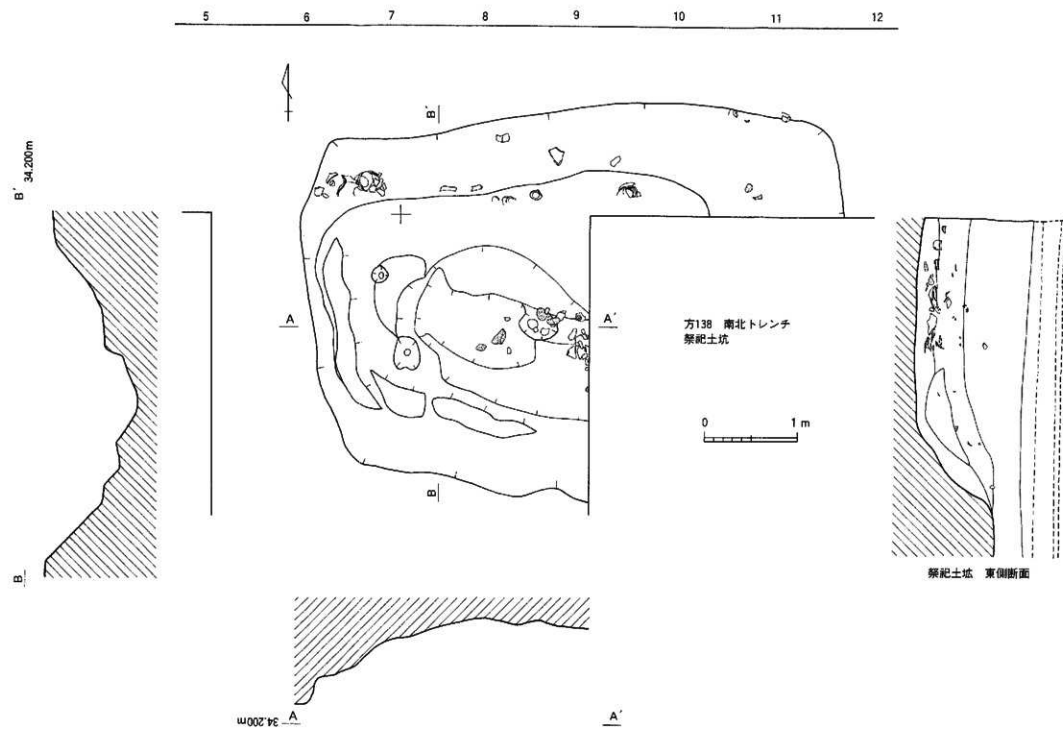
第144図 138番地 南北丁 祭祀土坑実測図
