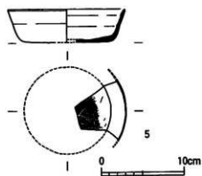
第293图 2号住居跡出土物実測図
