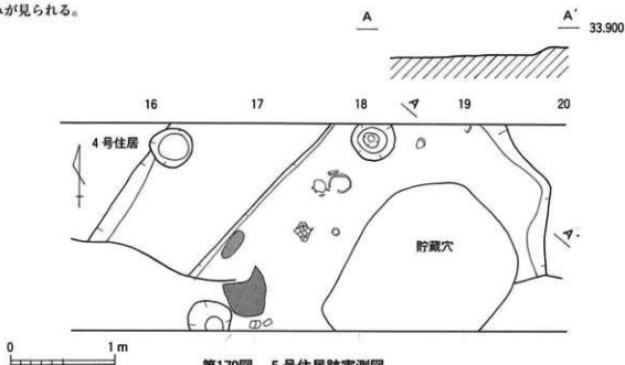
第179図 5号住居跡実測図
