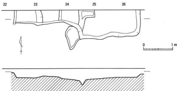
第296図 4号住居跡実測図
