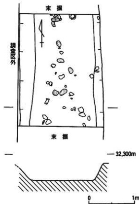
第390図 2号溝（掘下部分）実測図 (S=1/40)
