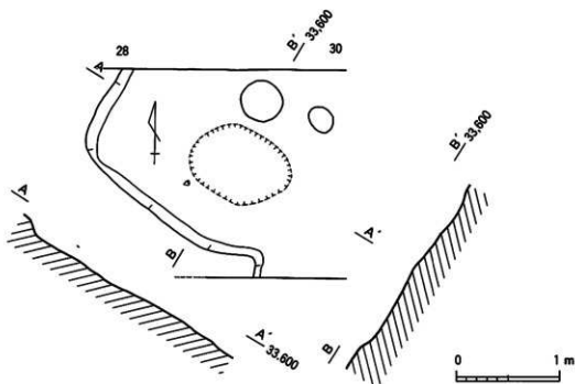
第161图 1号住居跡実測図
