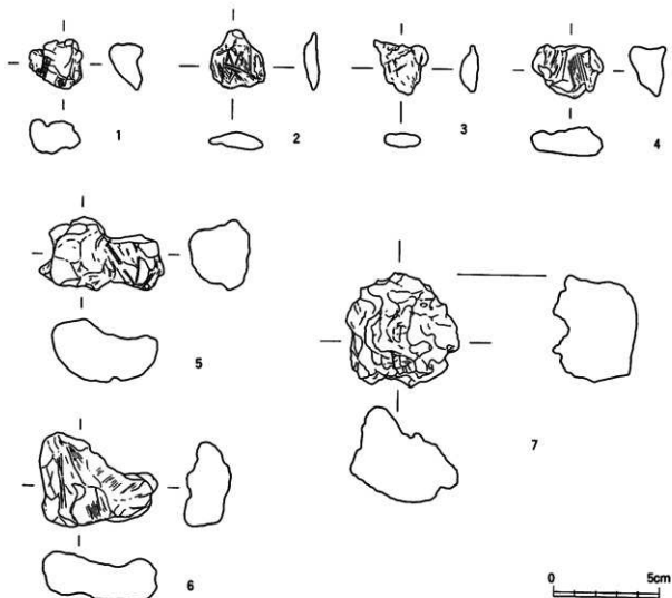
第432図 焼成粘土塊 実測図（S=1/2）
