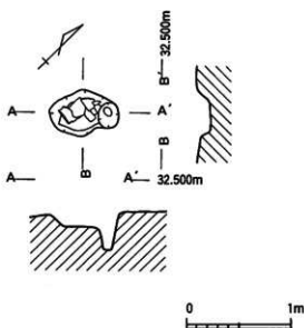
第420図 6号土坑 実測図 (S=1/40)
