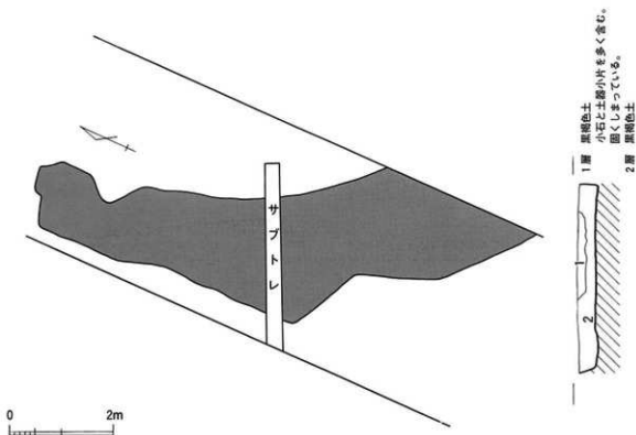
第434図 道路状遺構 実測図 (S = 1 / 80)
