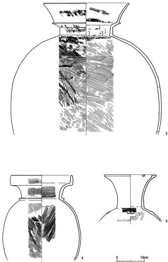
第93图 1号溝出土遺物実測図
