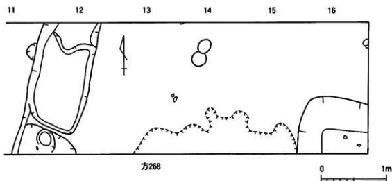
第229図 東西第3 T 住居跡実測図
