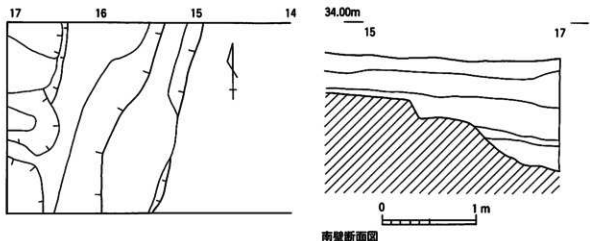
第231図 東西第4トレンチ 6号溝実測図
