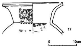
第441図 遺構に伴わない遺物実測図② (S=1/4)
