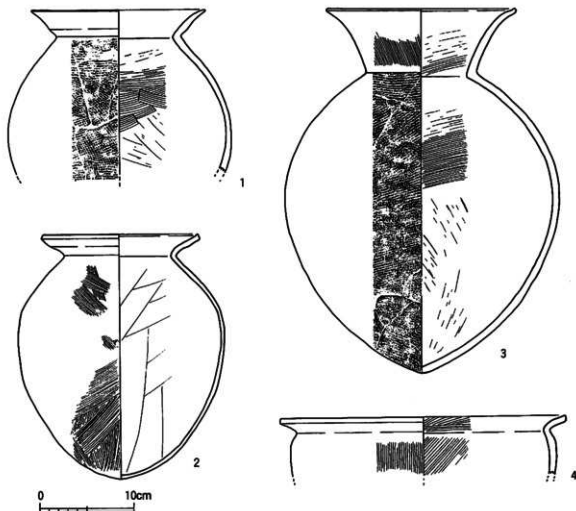
第51図 10号住居跡出土土器実測図
