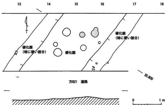
第315図 道路状遺構実測図
