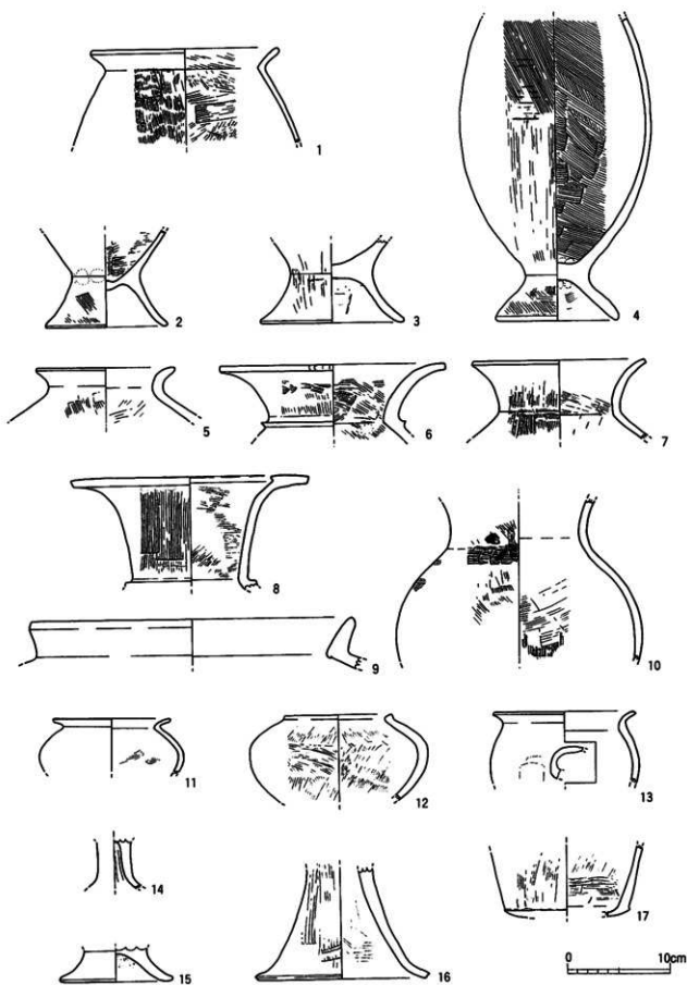
第402图 4号溝(上層)出土土器実測図(S=1/4)
