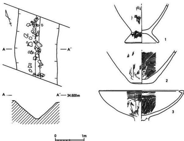
第337图 831番地4号溝 実測図 (S=1/40)
