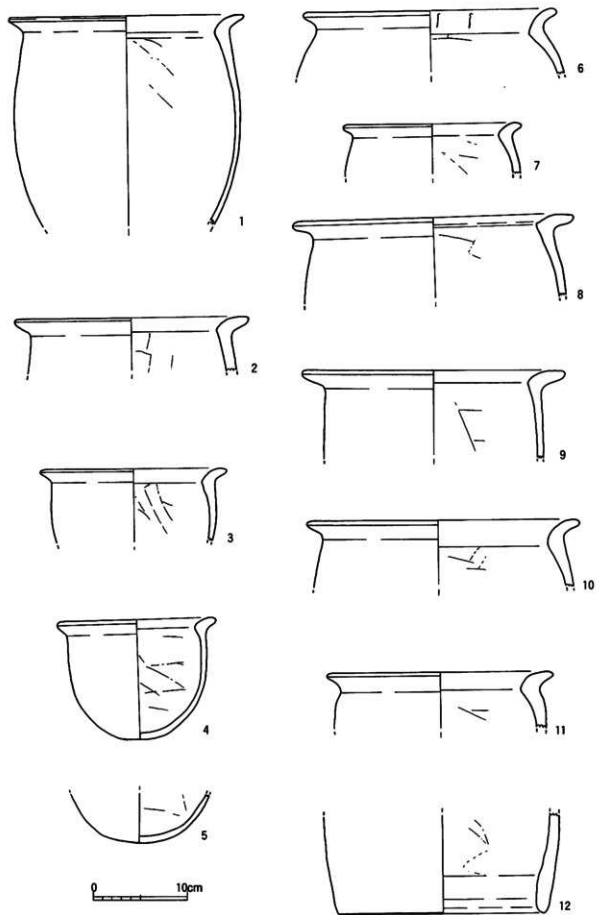
第443圖 焼土出土土器実測図 (S=1/4)
