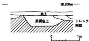
第333図 831番地 2号溝実測図 (S=1/40)
