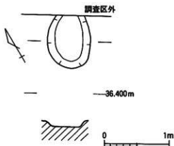
第351図 932-2番地 1号土坑実測図 (S=1/40)
