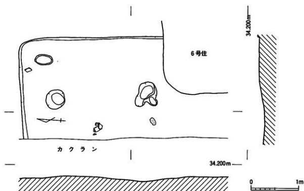
第37図 4号住居跡 実測図 (S=1/40)
