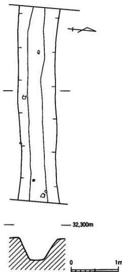
第388図 1号溝 実測図 (S=1/40)
