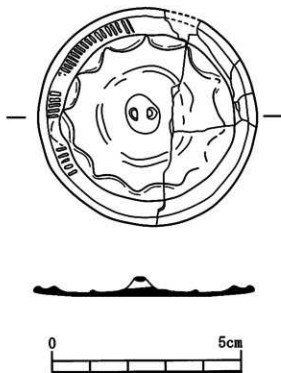
第46図 7号住居跡出土小型仿製鏡実測図(S=1/1)
