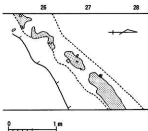
第251図 南北1T 2号道路実測図
