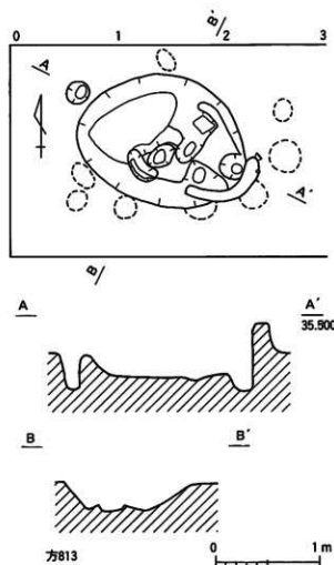
第262図 1号土坑実測図
