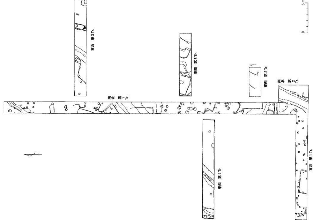
第215図 方保田268基地 遺構配置図 (S=1/250)
