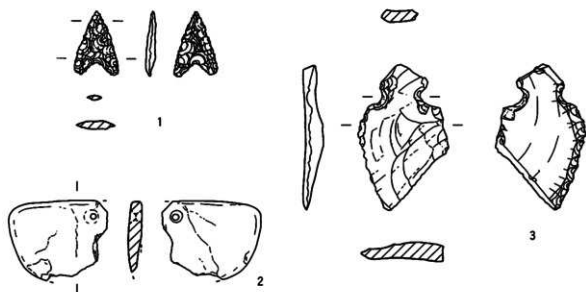
第439図 石器実測図 (1はS=1/1、2・3はS=1/2)
