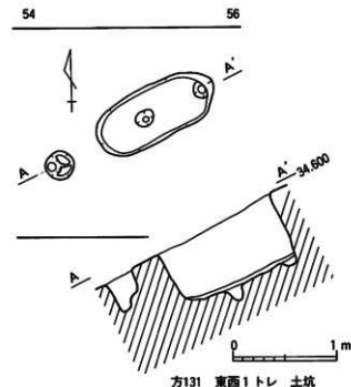
第107図 2号土坑実測図
