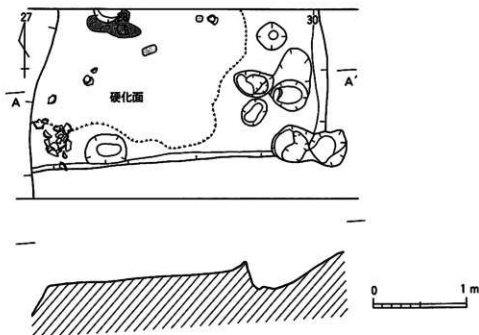
第128図 3号住居跡 実測図
