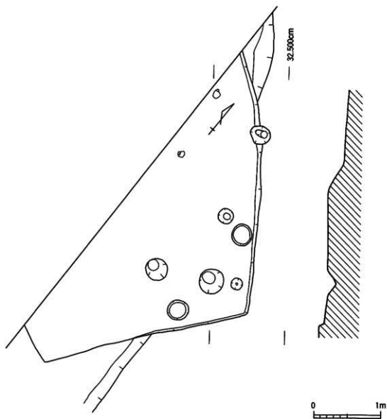
第413図 3号住居跡 実測図 (S=1/40)
