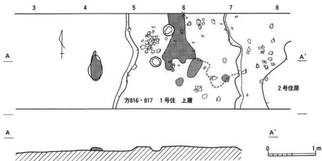
第289図 1号住居跡実測図
