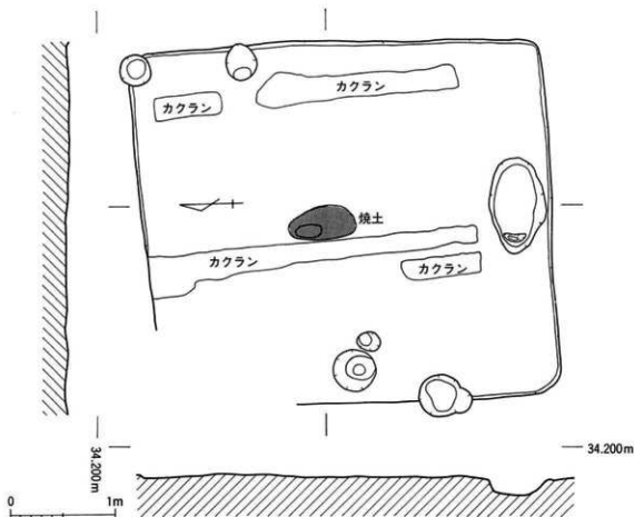
第47図 8号住居跡 実測図 (S=1/40)
