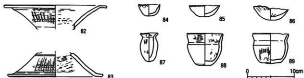
第21図 溝(上層)出土土器 実測図④ (S=1/4)
