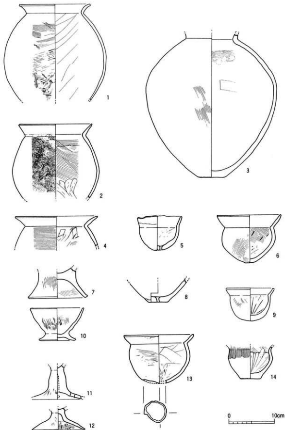
第60图 15号住居跡出土土器実測図
