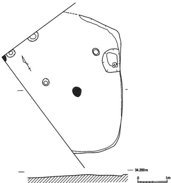
第32图 1号住居跡 実測図 (S=1/40)
