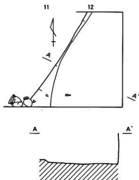
第240図 5号住居跡実測図
