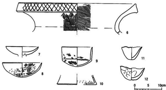
第94図 1号溝出土遺物実測図
