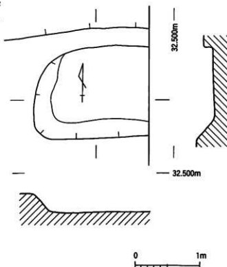
第426図 3号土坑 実測図 (S=1/40)
