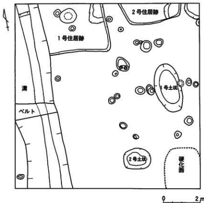
第3図 方保田84-2番地 遺構配置図 (S=1/100)
