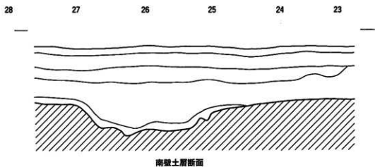
第130图 1号沟实测图
