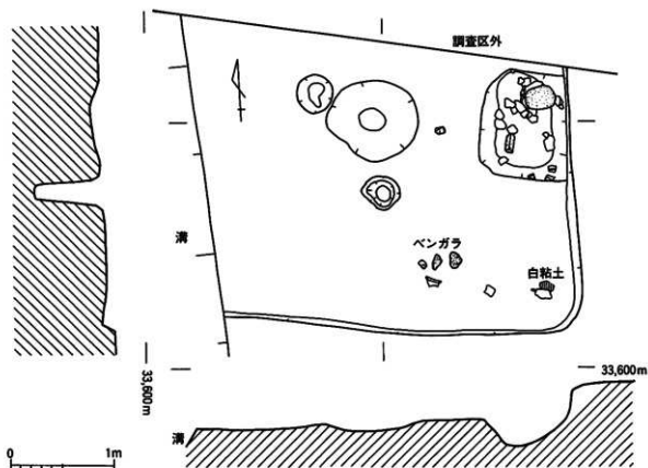
第5図 1号住居跡 実測図 (S=1/40)
