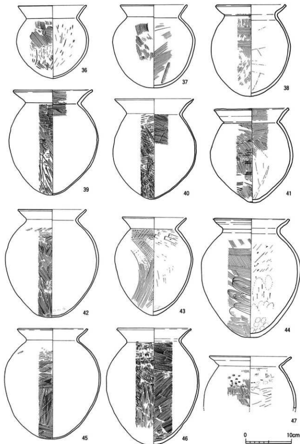
第18图 满(上層)出土土器 实测图① (S=1/4)
