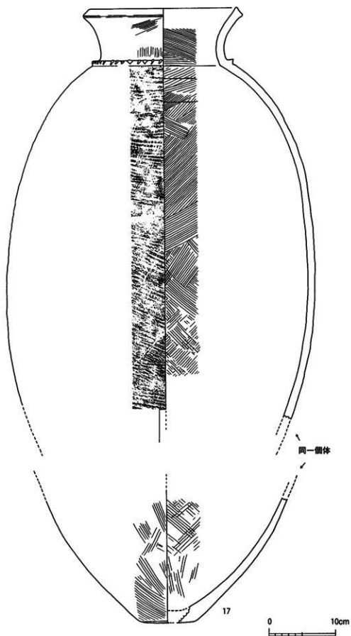
第371図 第2トレンチ3号溝出土土器実測図⑤(2層)
