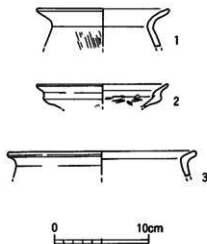
第416图 2号土坑出土土器实测图 (S=1/4)
