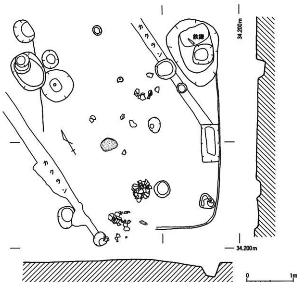
第50図 10号住居跡 実測図 (S = 1/40)
