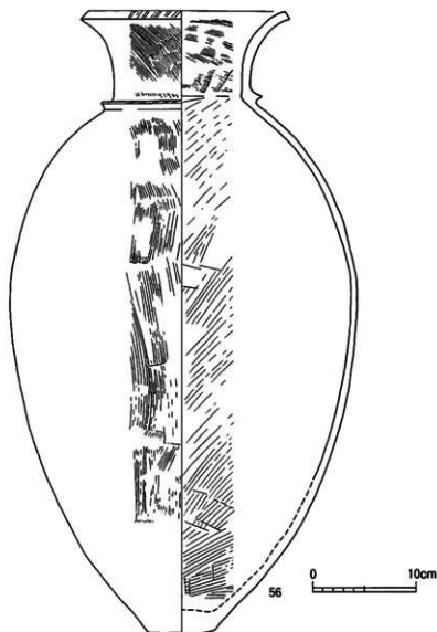
第381図 第2トレンチ3号溝出土土器実測図⑮（6層）
