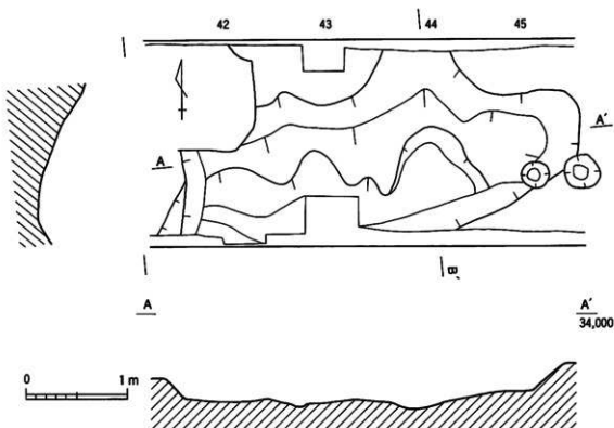
第304図 不整形土坑実測図
