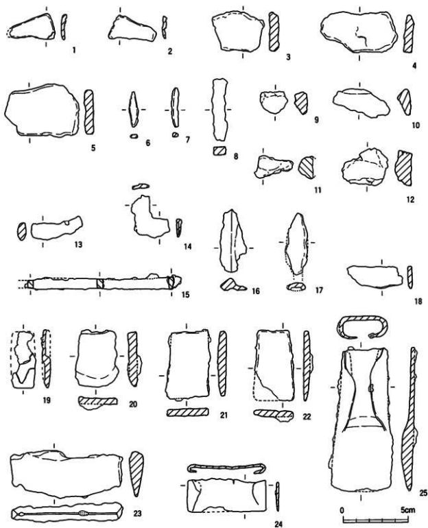
第27図 遺構に伴わない遺物（鉄器）実測図（S=1/2）
