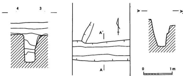
第246図 南北1 T 2号溝実測図
