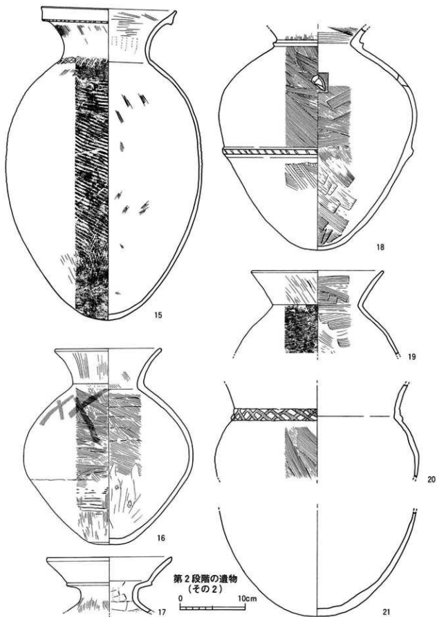
第148図 祭祀土坑出土遺物実測図②
