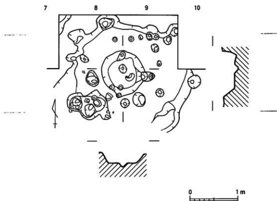
第327图 土坑实测图
