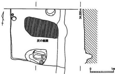
第34号 2号住居跡 実測図 (S=1/40)
