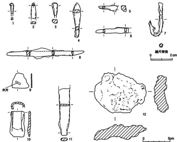
第422図 209番地出土鉄器実測図（S=1/2、7のみ等倍）
