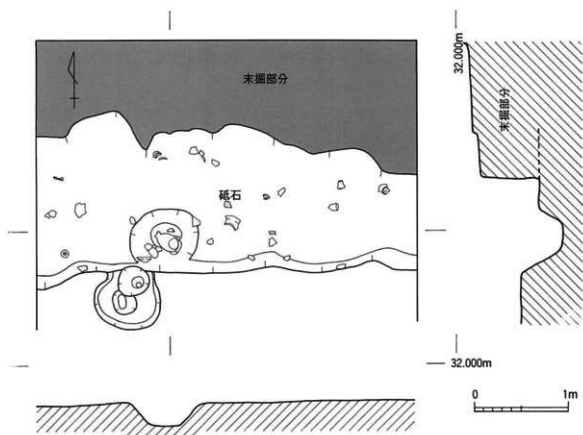
第411图 2号住居跡 実測図 (S=1/40)
