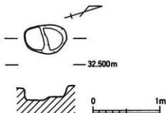
第419図 5号土坑 実測図 (S=1/40)
