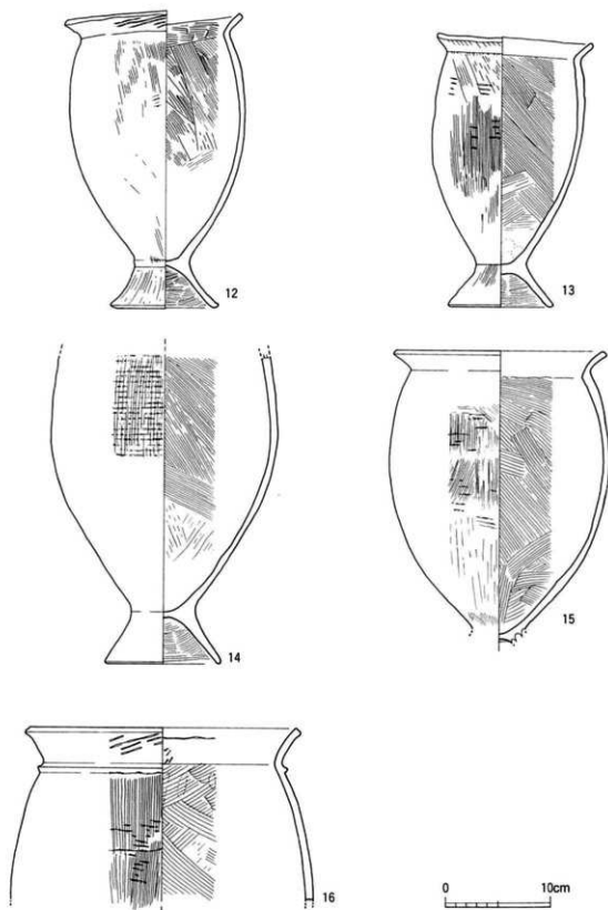
第370図 第2トレンチ3号溝出土土器実測図④(2層)
