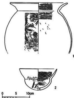
第209図 1号住居跡出土遺物実測図
