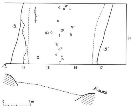
第122図 方136-1番地 第2トレンチ 溝実測図
