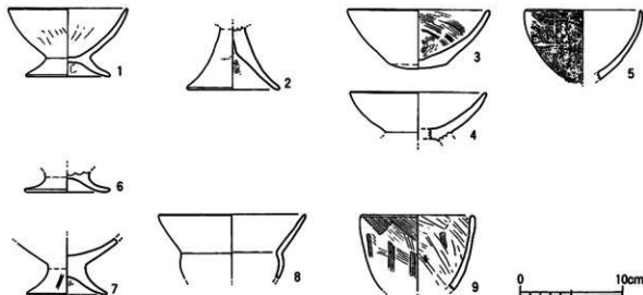
第72図 土坑出土土器実測図
