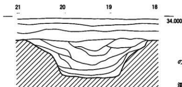
第219図 東西1 T 1号溝南側断面図
