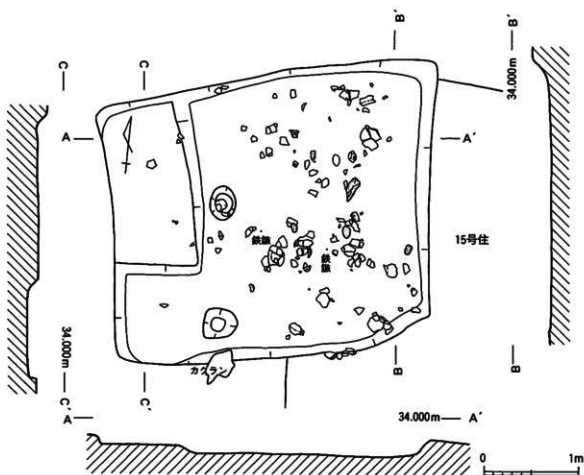
第57図 14号住居跡 実測図 (S=1/40)
