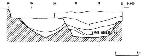
第254図 南北第1トレンチ自然災害遺構・第2トレンチ1号溝断面図
