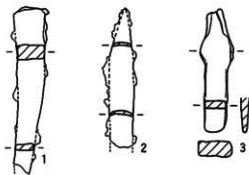
第340図 方保田831番地出土鉄実測図 (S=1/2)
