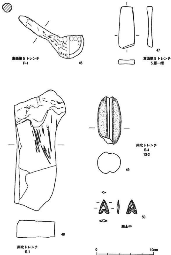
第452図 268番地出土の特殊な遺物実測図⑤
