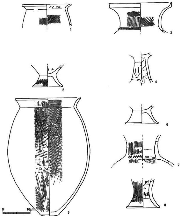
第228图 1号清出土文物实测图
