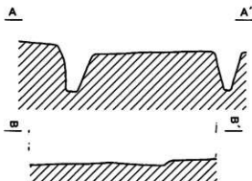
第313図 1号住居跡実測図
