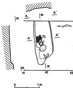
第252図 南北1T 土坑実測図
