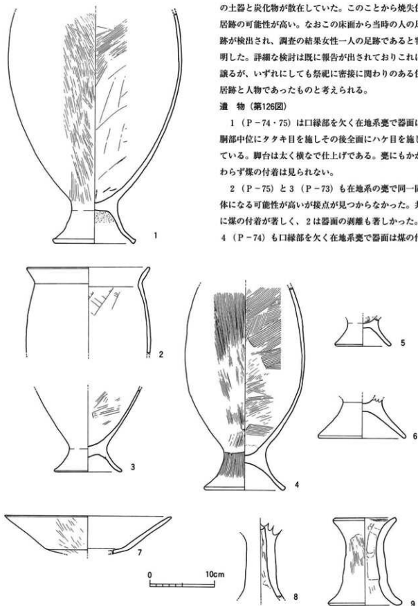
第126図 1号住居出土遺物実測図
