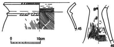
第401図 3号溝(下層)出土土器実測図 (S=1/4)
