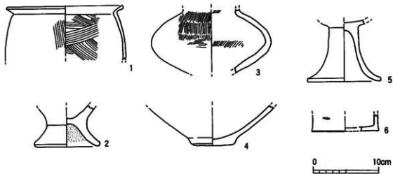
第261图 溝出土遺物実測圖
