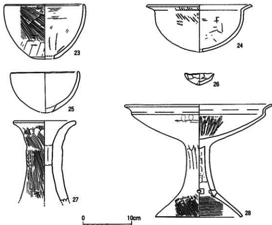
第373図 第2トレンチ3号溝出土土器実測図⑦（2層）
