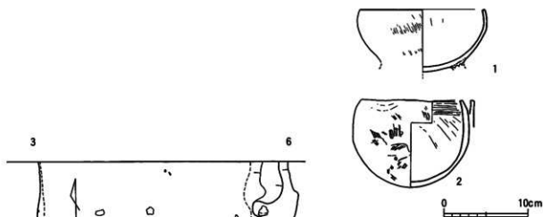
第162图 1号住居跡出土遺物実測図
