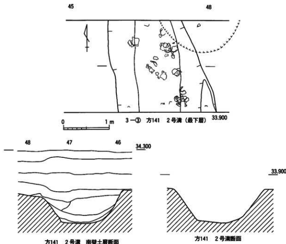
第190図 2号溝実測図
