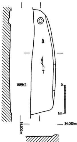
第61図 16号住居跡 実測図
