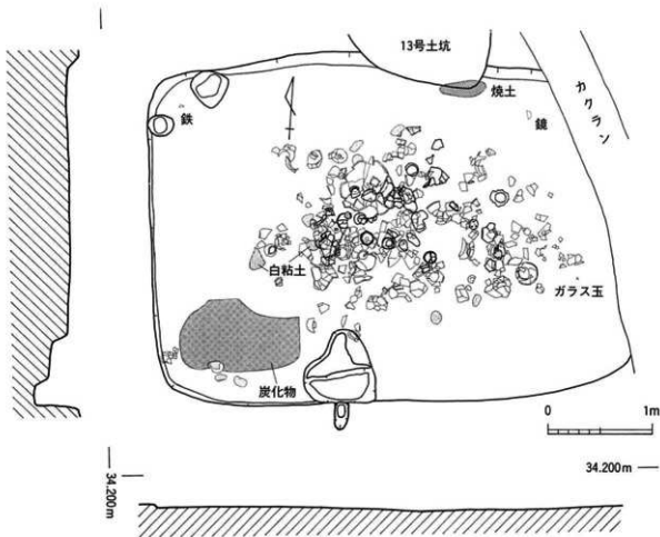
第41図 7号住居跡 実測図 (S=1/40) [淡色は上層]
