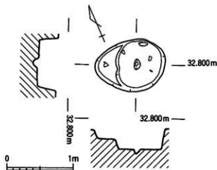
第382図 第2トレンチ1号土坑 実測図 (S=1/20)
