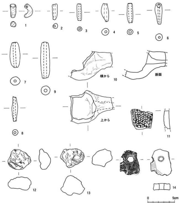
第343図 831番地出土その他の遺物実測図（土鍾など）（S=1/2）
