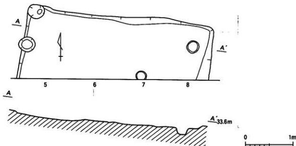
第217図 方268 東西1 T 1号住居実測図
