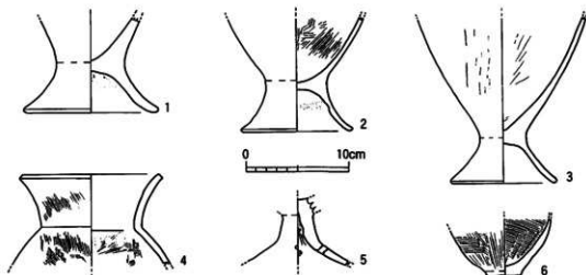
第324図 溝出土遺物実測図
