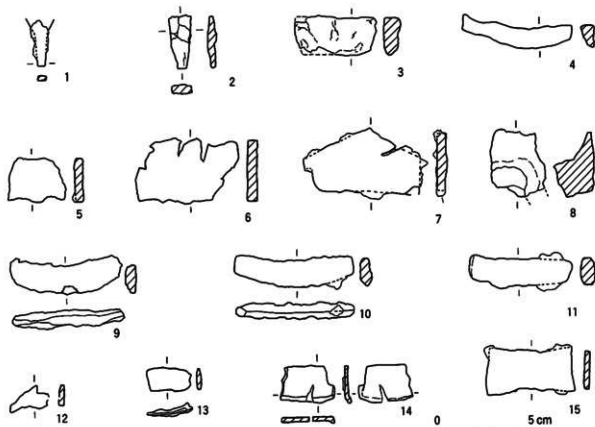
第10図 84-2番地 2号住居跡出土鉄器実測図 (S=1/2)
