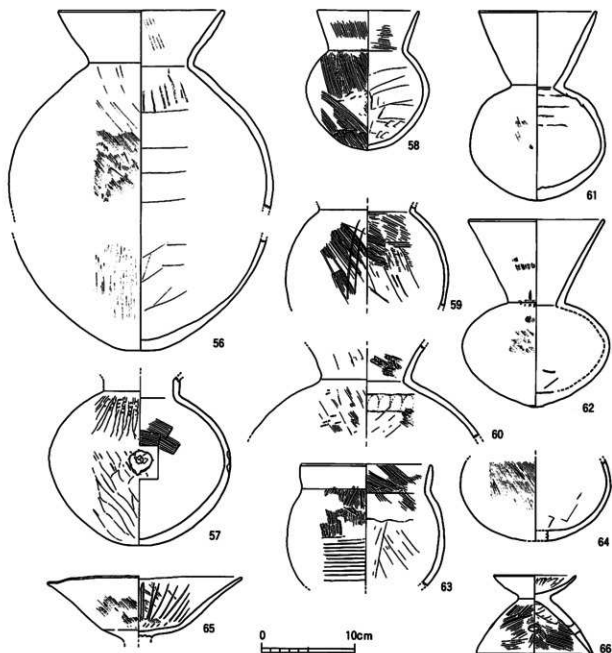
第153図 祭祀土坑出土遺物実測図④
