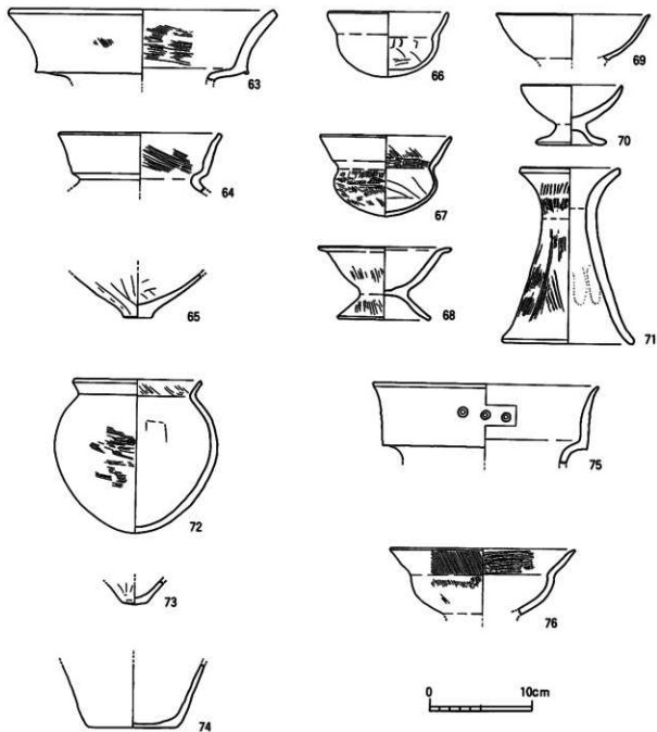
第204図 遺構に伴わない遺物実測図
