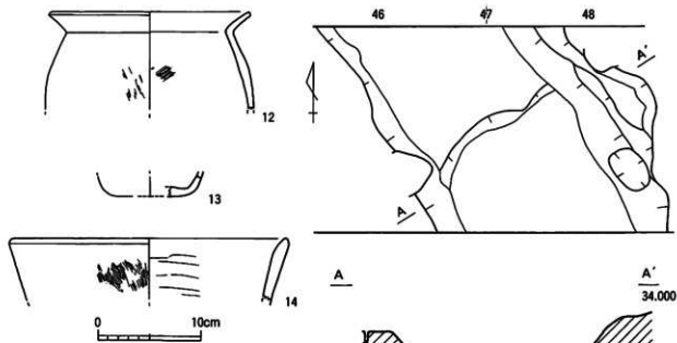
第301図 6号住居跡出土遺物実測図
