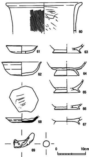
第142図 1号道路出土遺物実測図
