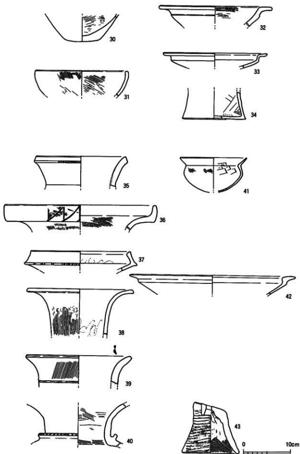
第117図 遺構に伴わない遺物実測図
