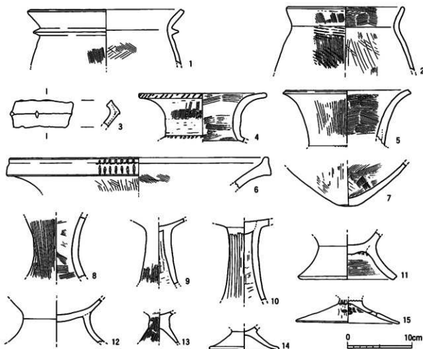
第391図 2号溝出土土器実測図 (S=1/4)
