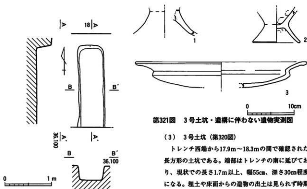
第320図 3号土坑実測図
