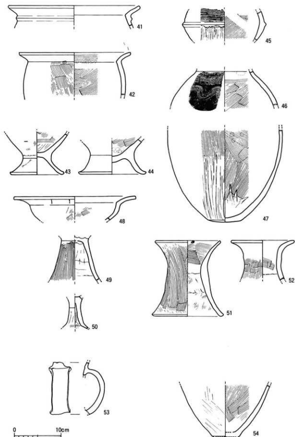
第138图 3号溝出土遺物実測図
