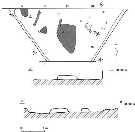
第110図 132番地 1号住居跡実測図
