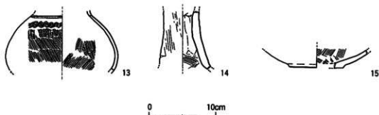
第95図 1号溝出土遺物実測図
