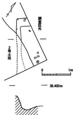
第353図 932-2番地 3号土坑実測図 (S = 1/40)
