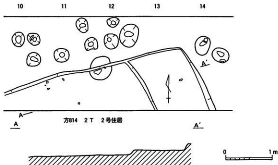
第268図 2号住居跡実測図
