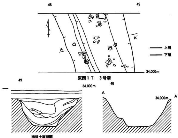
第137図 方138番地 東西1 T 3号溝実測図
