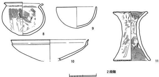
第223図 1号溝出土遺物実測図
