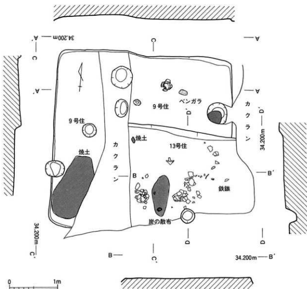
第48図 9号住居跡・13号住居跡 実測図 (S=1/40)
