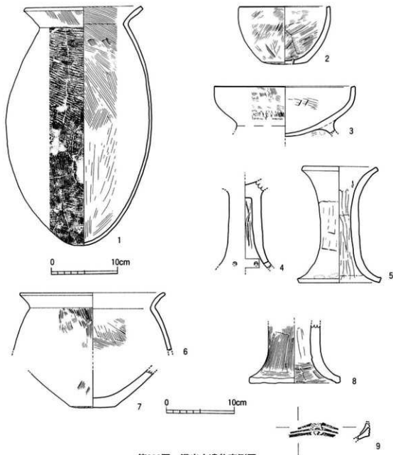
第309図 溝出土遺物実測図
