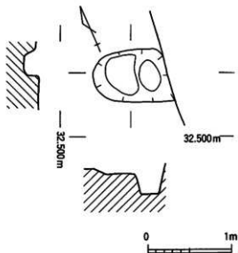
第417图 4号土坑 实测图 (S=1/40)
