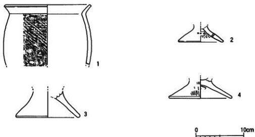
第33图 1号住居跡出土土器実測図① (S=1/4)
