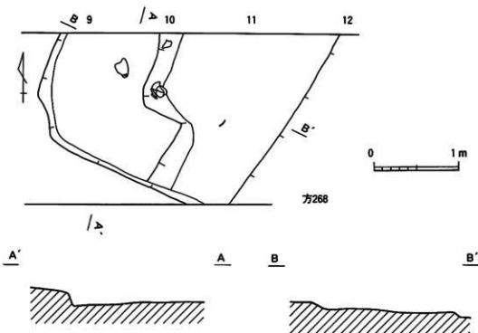
第237図 東西5 T 4号住居跡実測図
