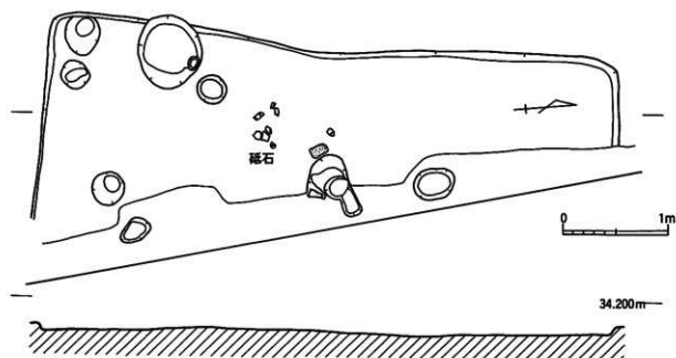
第38図 5号住居跡 実測図 (S=1/40)
