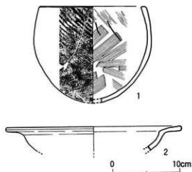
第54图 11号住居跡出土土器実測図
