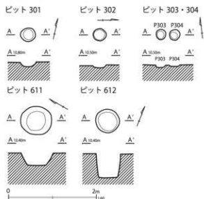
第225図 ビット
