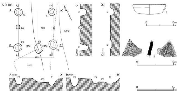
第131図 第105号掘立柱建物跡・出土遺物
