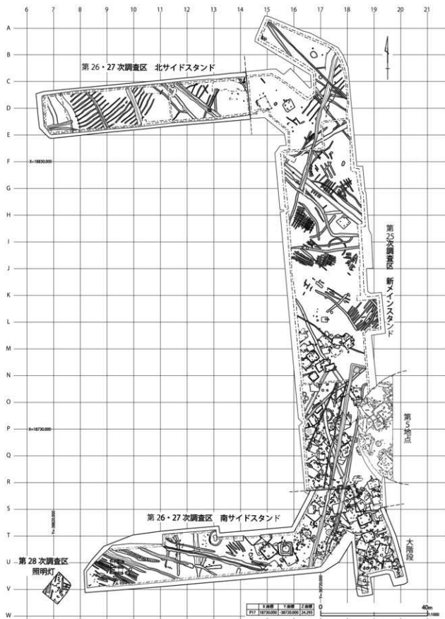
第8図 北島遺跡第26～28次全体図
