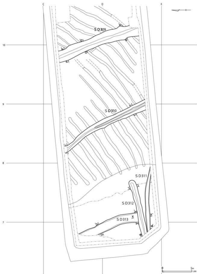
第146図 古代の溝跡全体図（5）
