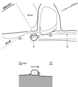
第22図 第120・121・150号住居跡・遺物出土状況
