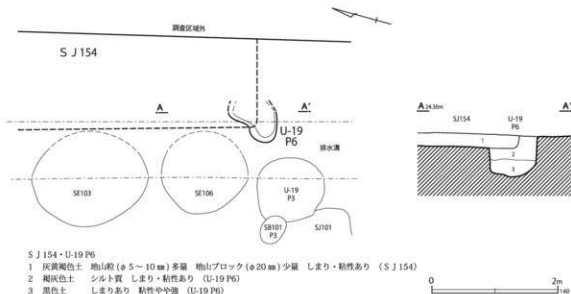
第57図 第154号住居跡
