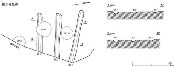
第177図 第5号畝跡
