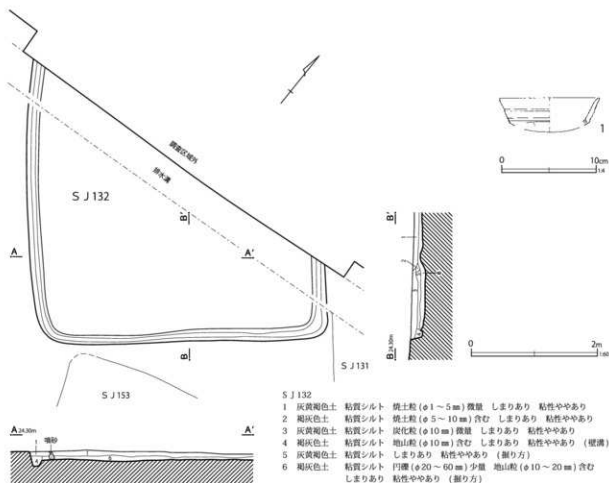
第40図 第132号住居跡・出土遺物
