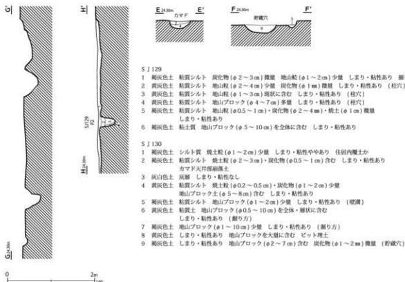
第35図 第129・130号住居跡（2）
