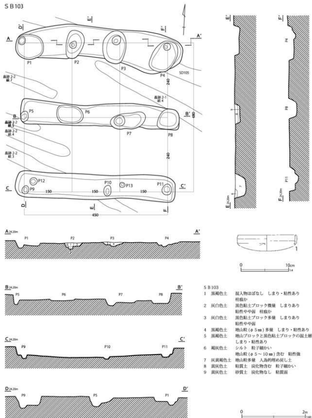
第63図 第103号掘立柱建物跡・出土遺物
