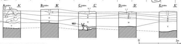
第26・27地点基本土層（南サイドスタンド）
