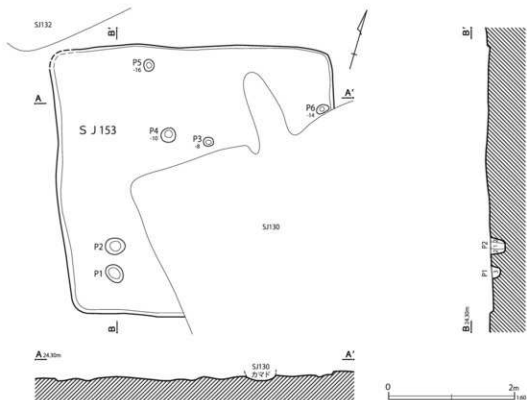
第56図 第153号住居跡
