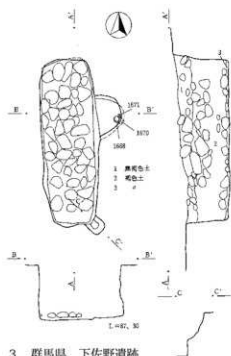
3 群馬県 下佐野遺跡 7区113号土坑
