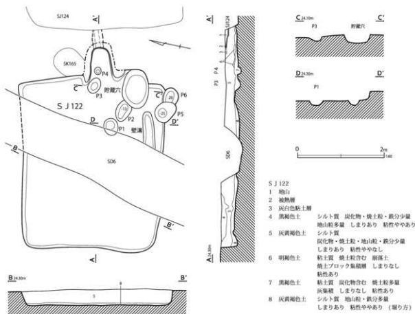
第105図 第122号住居跡
