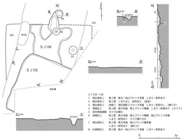
第43図 第134・135号住居跡
