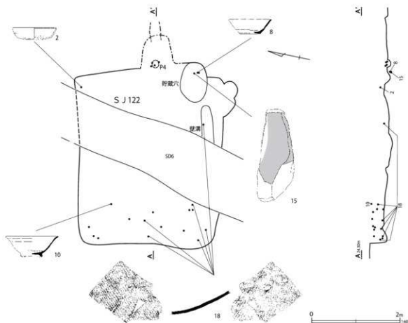
第106図 第122号住居跡遺物出土状況
