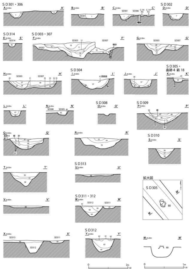
第147図 古代の溝跡土層図（2）
