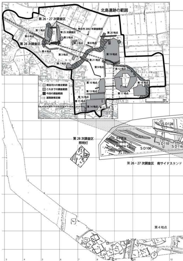
第192図 第101号道路跡、第3・4・6号溝跡位置図(1)
