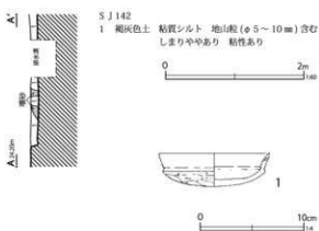
第54図 第142号住居跡・出土遺物
