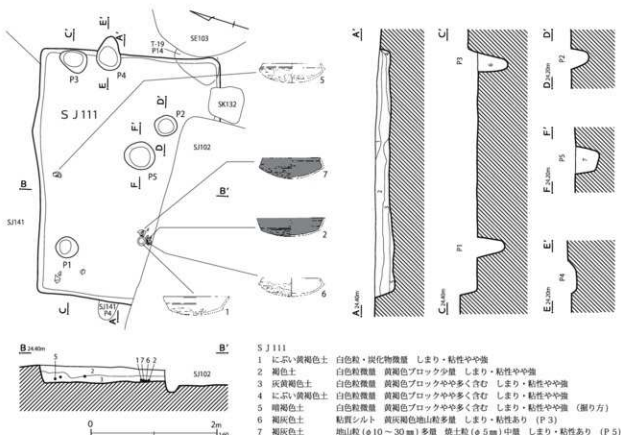
第18図 第111号住居跡・遺物出土状況
