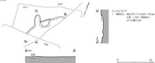
第55図 第151号住居跡
