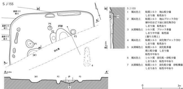
第58図 第155号住居跡・遺物出土状況
