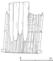
井桁立面図 (北側)
