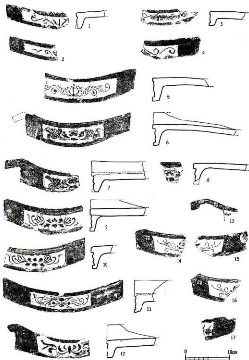
Fig. 15 瓦類実測図① (S=1/4)
