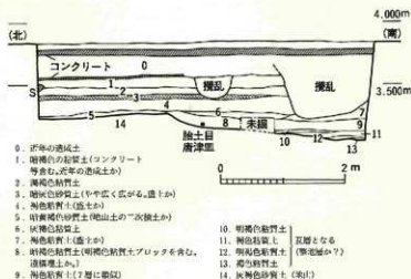
Fig. 5 調査区東壁土層図 (S=1/60)
