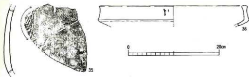
Fig.10 SK 1 出土遺物④ (S=1/4)
