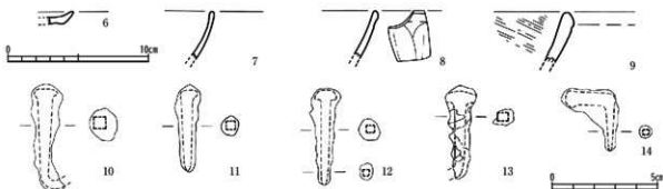
第14図 ST135出土遺物実測図（10～14は1/2、他1/3）
