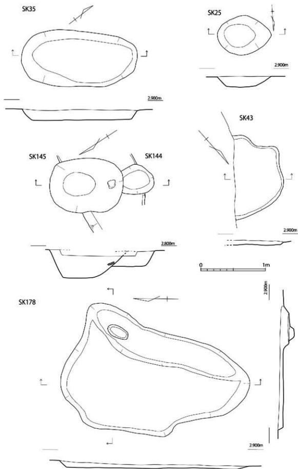
第15図 土坑実測図① (1/30)
