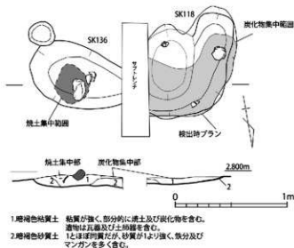
第17図 土坑実測図③ (1/30)
