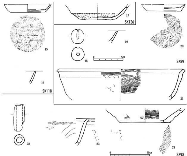
第18図 土坑出土遺物実測図 (18・22は1/2、他1/3)
