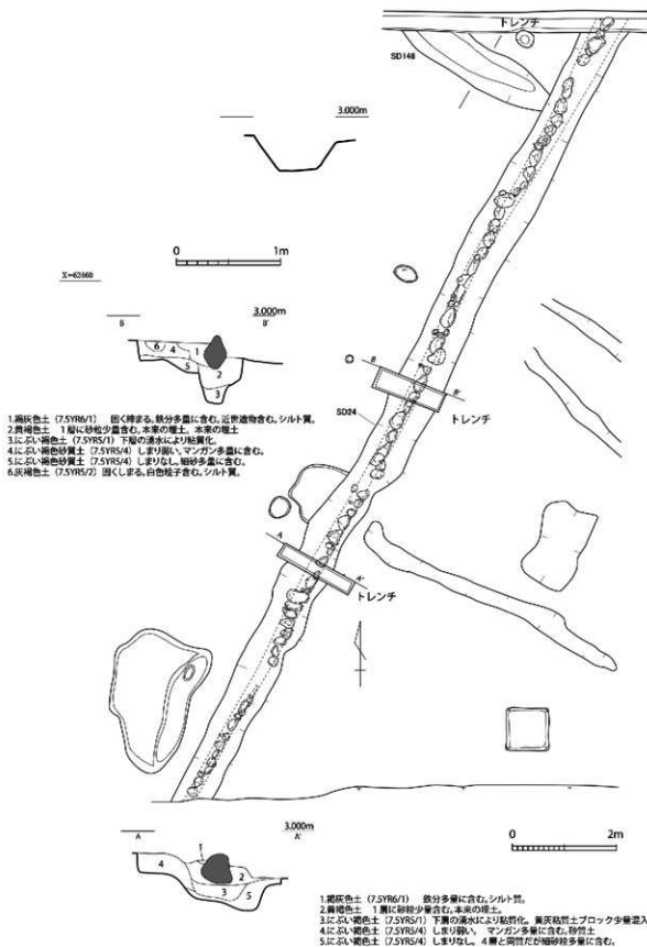
第20図 SD24・146実測図 (断面1/40・平面1/80)
