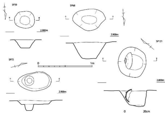
第24図 ピット実測図 (SP121は1/10、他1/20)
