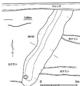
第21図 SD123実測図 (1/60)
