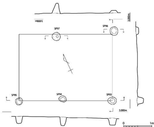
第9図 SB1実測図 (1/40)
