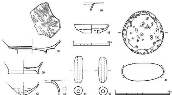
第26図 調査区出土遺物実測図 (44～46は1/2、他1/3)
