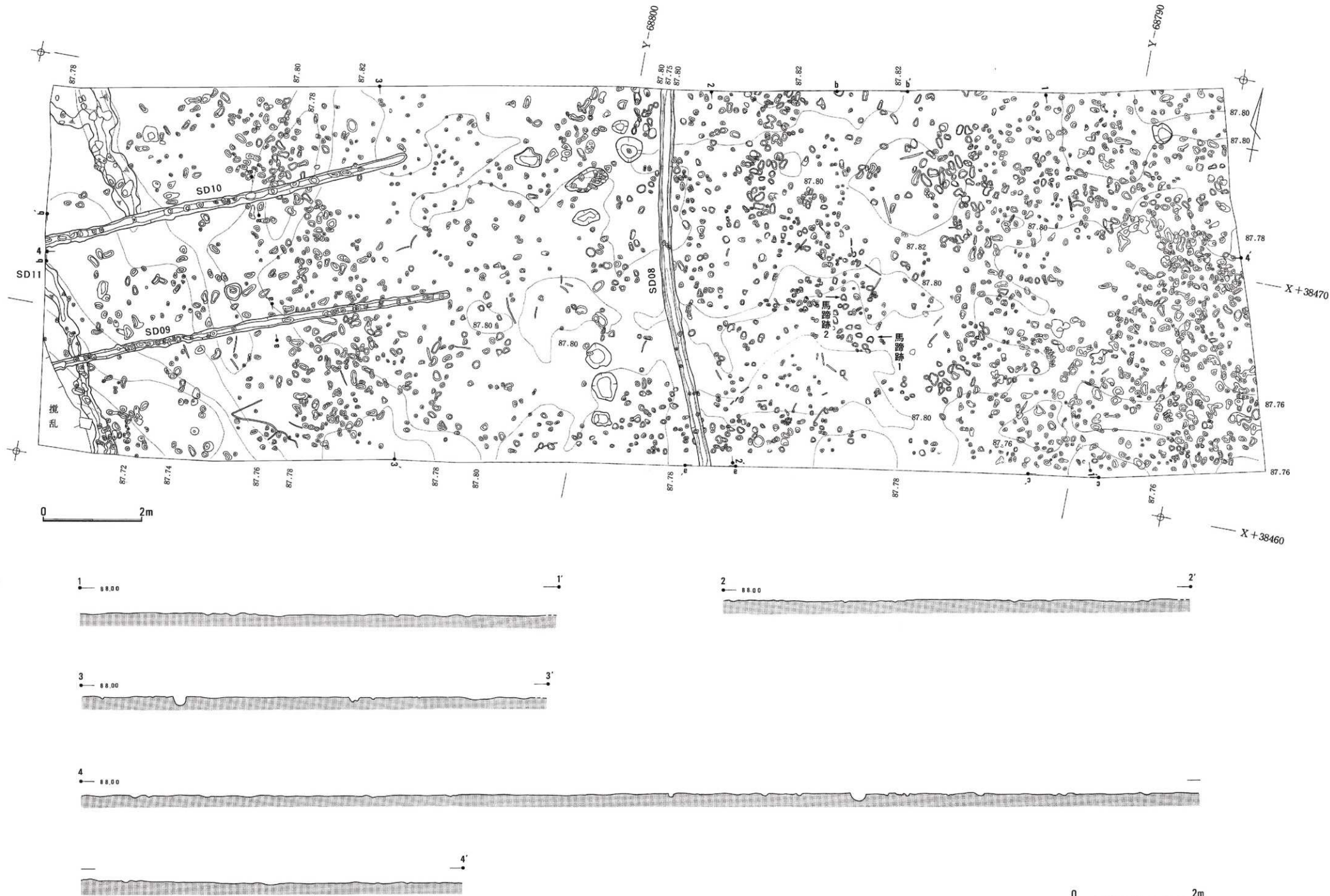
付図 京目杉ノ内・大沢大沢西遺跡 6区全測図
