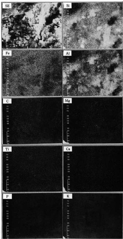
Photo. I 方保田東原遺跡出土、石胞丁形鉄器 (M-861) の特性X線像 (×1400)
