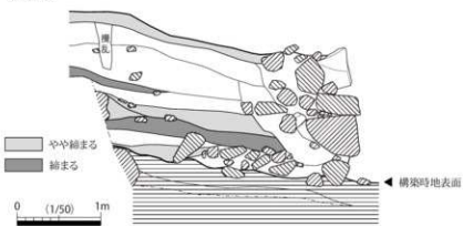
第18図 石垣構築状況模式図
