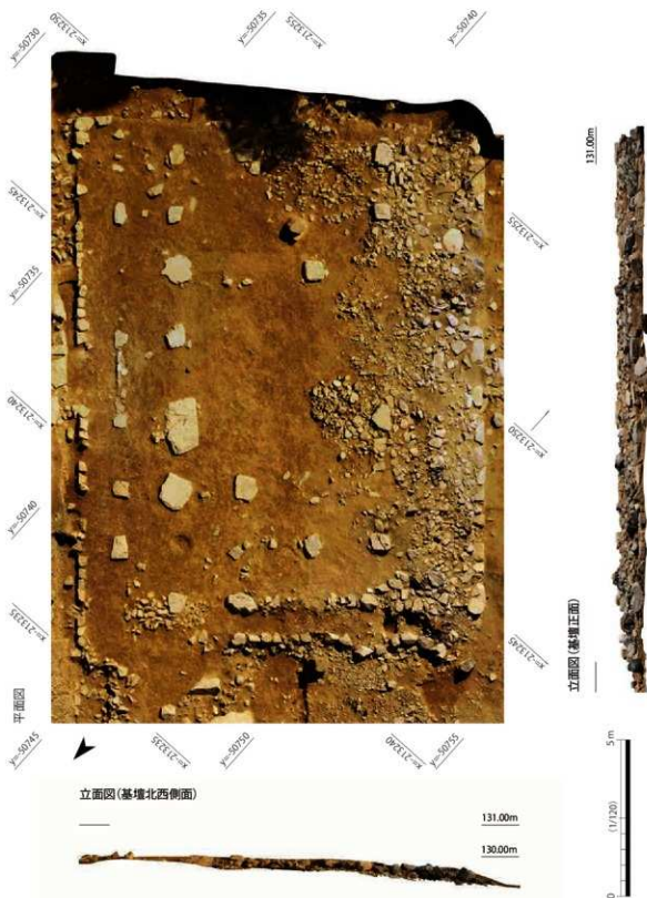
第61図 基壇をもつ礎石建物平面図・立面図 (オルソン画像)
