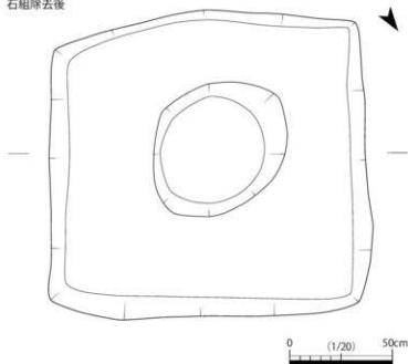
第33図 方形石組平面図（石組除去後）
