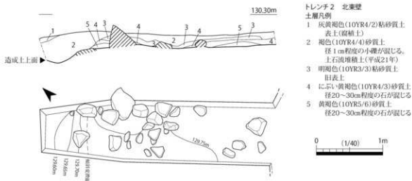
第8図 トレンチ1・2平面図・土層断面図
