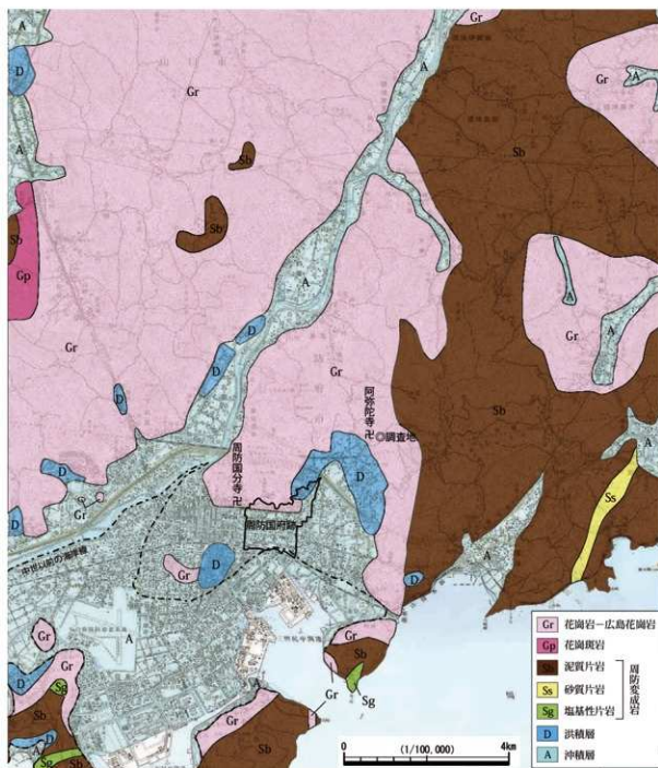
第2図 阿弥陀寺周辺の地質分布
