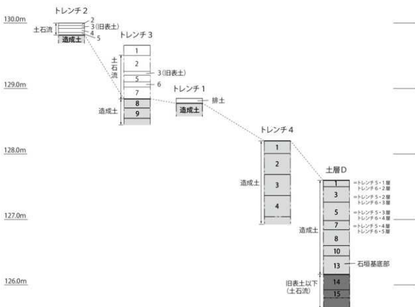
第14図 中段造成状況模式図
