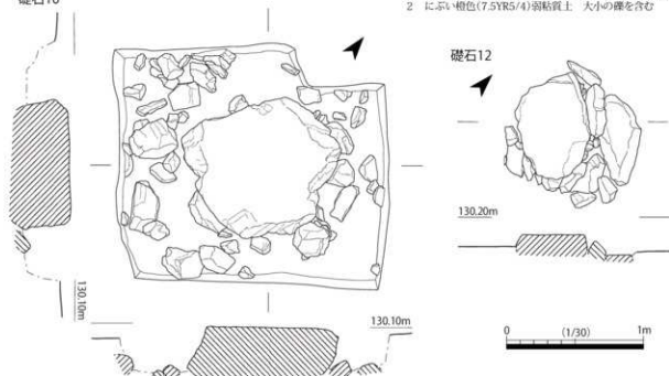
第27図 礎石及びその周辺平面図・土層断面図(1)
