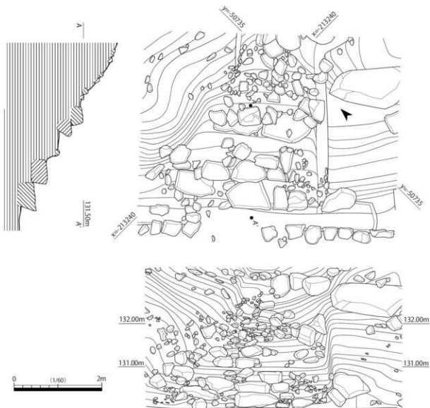
第 29 図 石段 2 平面図・立面図・断面図
