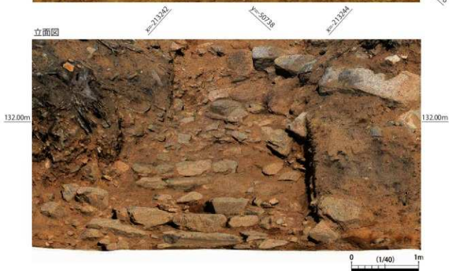
第 62 図 石段 2 平面図・立面図（オルソ画像）
