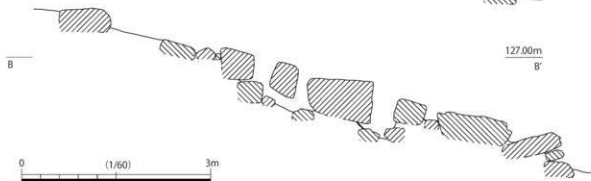
第 16 図 石段 1 立面（側面）図・断面図
