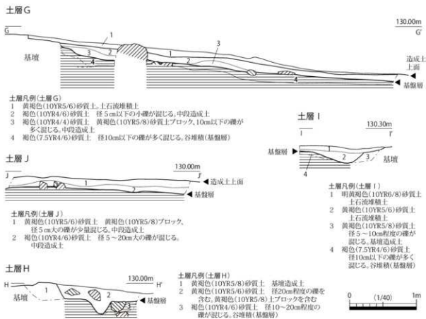
第 25 図 基壇及びその周辺土層断面図(2)
