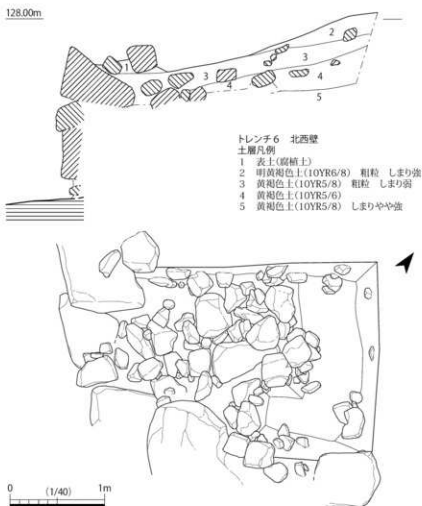
第12図 トレンチ6平面図・土層断面図
