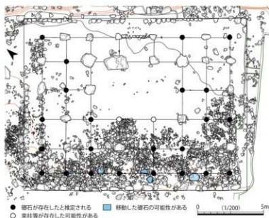
第40図 礎石建物の礎石配置平面図 (山岸氏の原案をもとに作成) 上: 礎石番付と礎石間隔、下: 礎石配置平面
