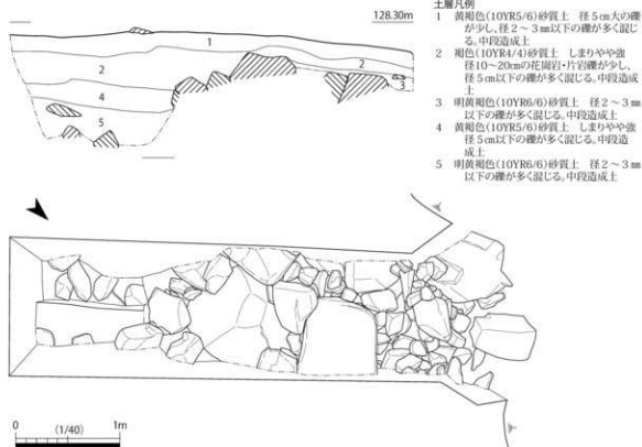
第10図 トレンチ4平面図・土層断面図
