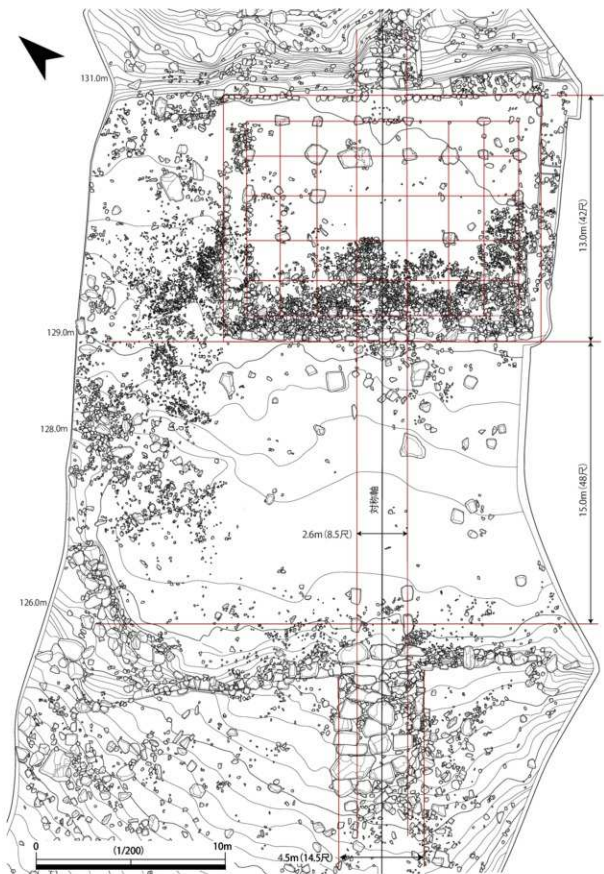
第 46 図 阿弥陀寺調査地の建築計画
