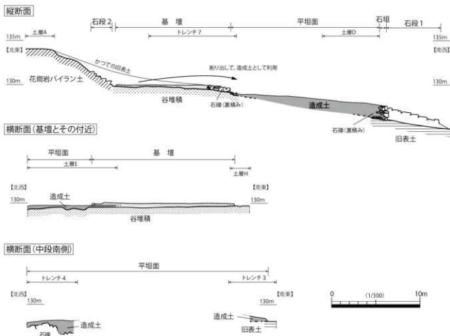
第 47 図 調査地の断面模式図
