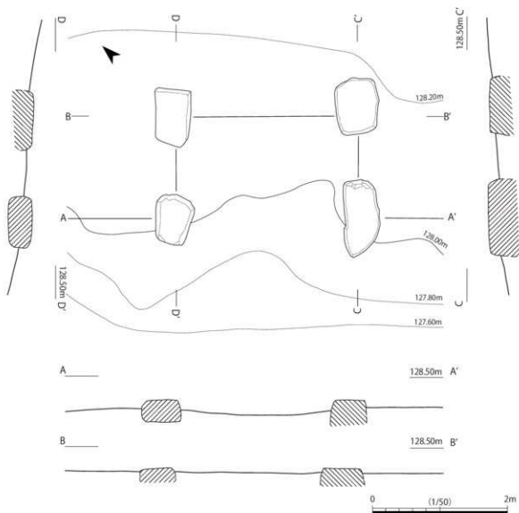
第19図 門礎石平面図・断面図
