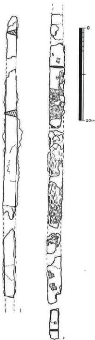
第10図 鉄剣・鉄刀実測図 (1/4)
