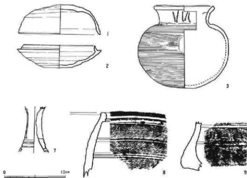
第11図 出土土器実測図 (1/3)
