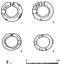
第8図 出土装身具実測図 (2/3)
