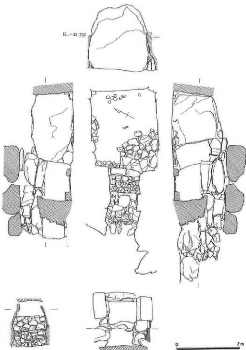
第6図 6号墳石室実測図 (1/80)
