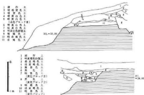
第4図 墳丘・版築状況実測図 (1/40)
