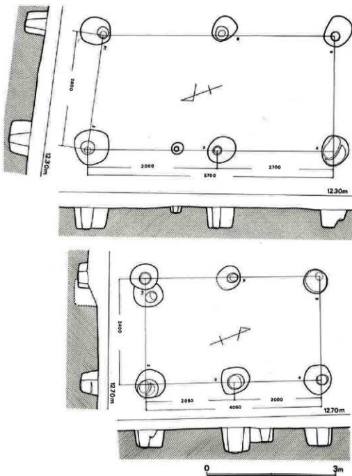
第8图 11号·12号掘立柱建物実測図 (1/60)
