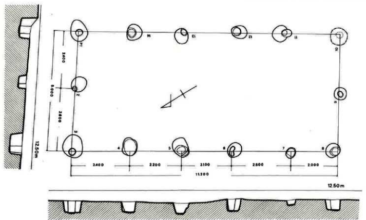
第6图 8号·13号榑立柱建筑物实测图 (1/80)
