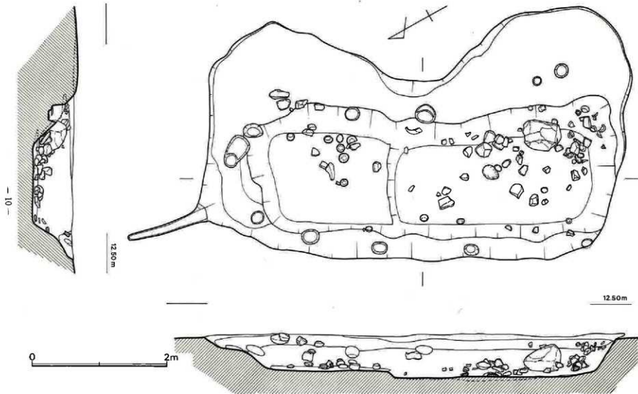
第9図 豎穴遺構実測図(1/40)
