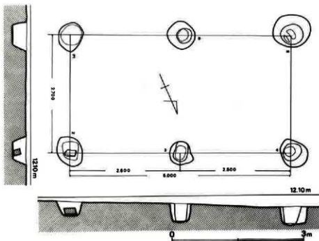
第7図 9号・10号掘立柱建物実測図（1/60）
