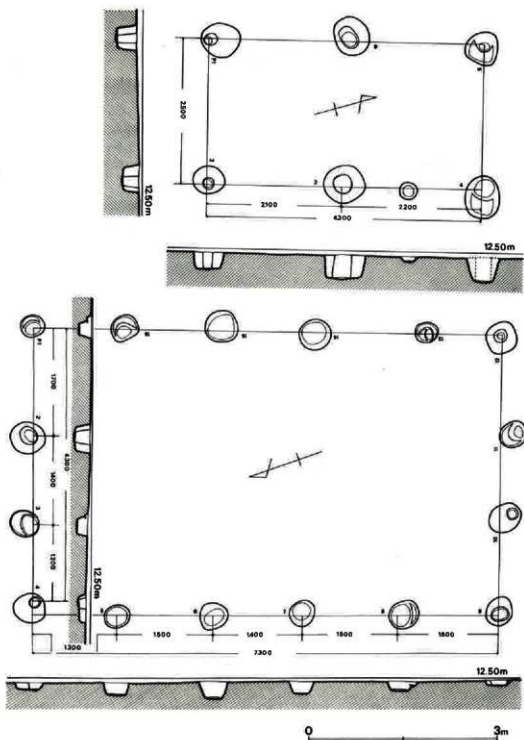
第4图 2号·3号孤立柱建物实测图(1/60)
