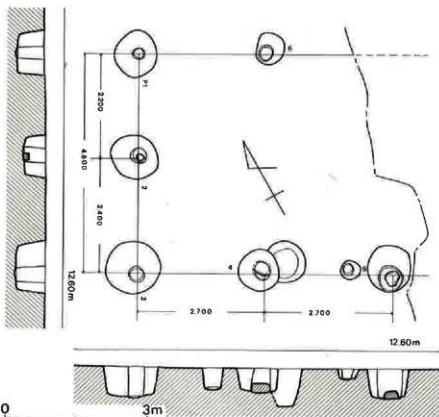
第5図 4号掘立柱建物実測図（1/80）
