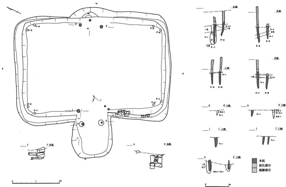
図面-4 炭焼窯跡1号
