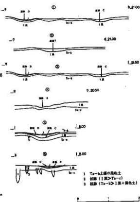
図Ⅵ-40 道跡位置図・断面図
