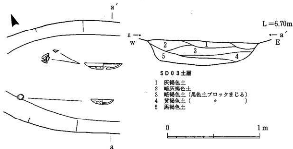
第7図 SD 03 (1:20)
