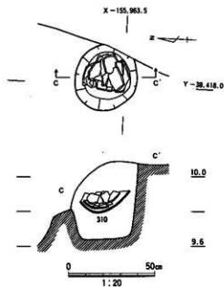
図83 I区SP701と出土遺物
