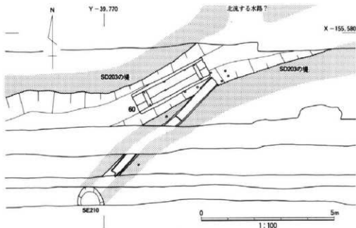
図35 Ⅷ区SD203と木樋
