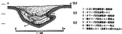
図75 I区SD801の断面
