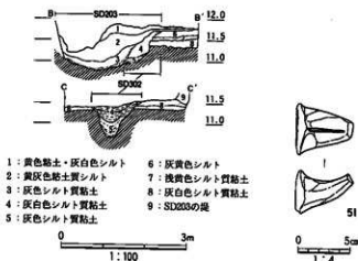
図31 Ⅶ区SD302と出土遺物
