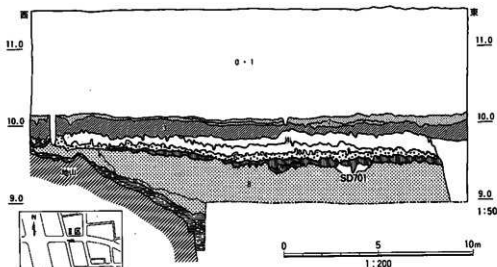
図52 II区地層断面
