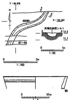
図30 Ⅲ区SD301と出土遺物
