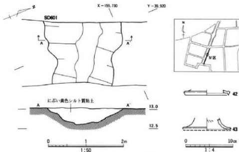
図17 N区SD601と出土遺物
