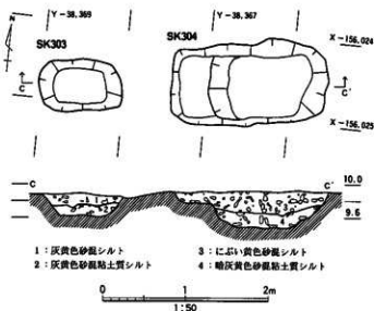
図89 I区SK303とSK304
