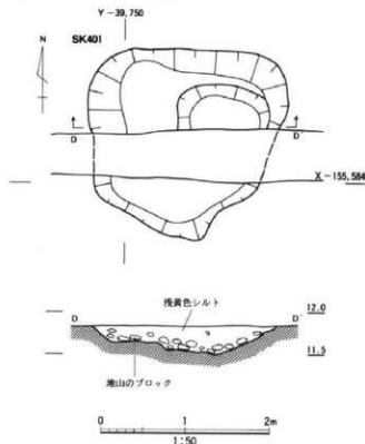
図21 V区SK401と出土遺物
