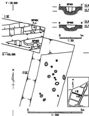
図19 I区SP401・402とⅡ区
