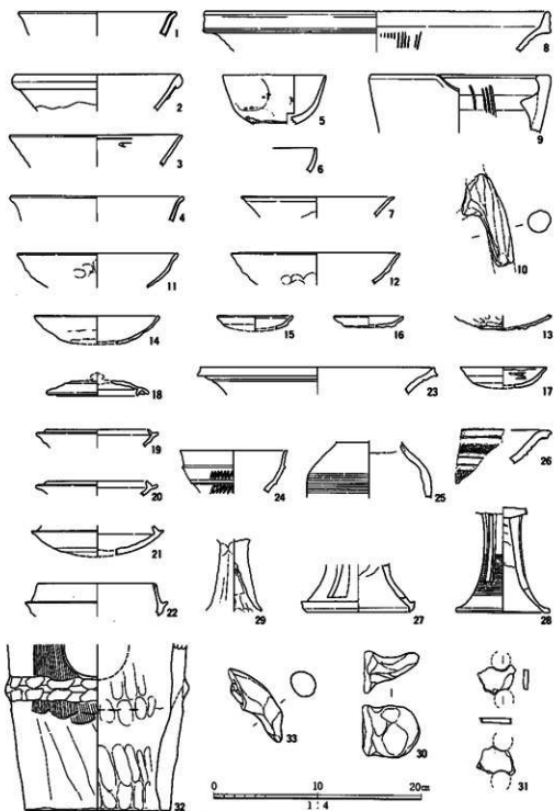
図10 各層出土の遺物(陶磁器・土器・埴輪)
