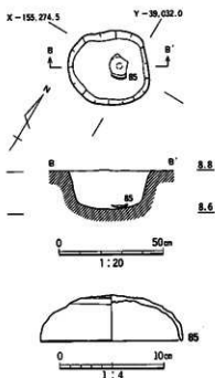
図45 I区SK701と出土遺物
