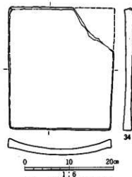
図11 各層出土の遺物(瓦)
