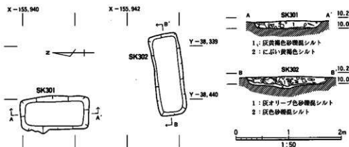
図88 I区SK301とSK302
