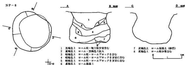
図III-14 NP-5・NP-7と出土遺物・NP-8
