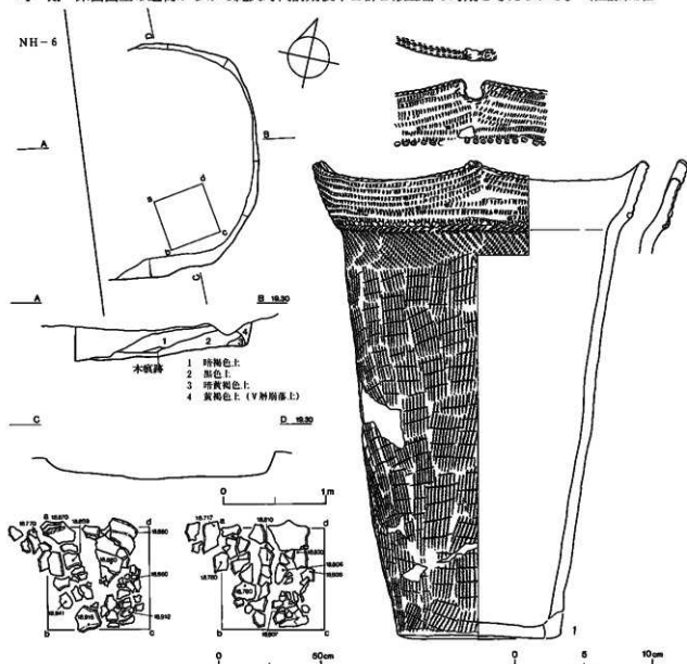
図Ⅲ-10 NH-6と出土遺物
