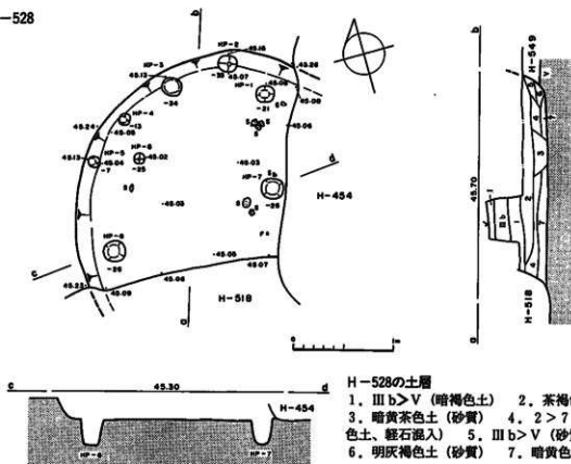
図Ⅲ-378 H-528実測図
