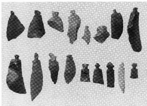
1 石匙
