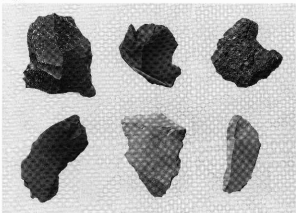
2 挟入石器
