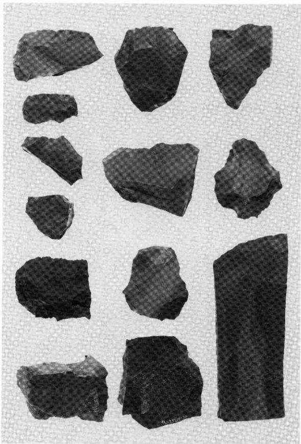
石核
