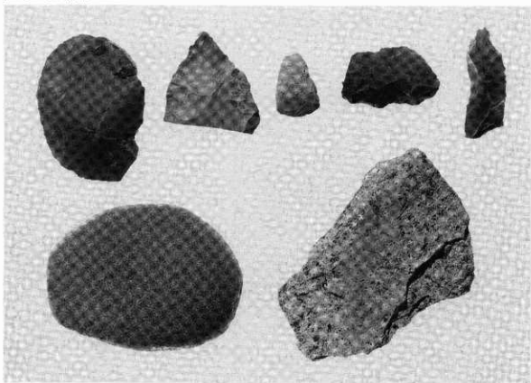
2 P-7の石器
