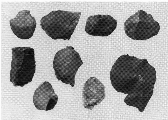
1 撿器
