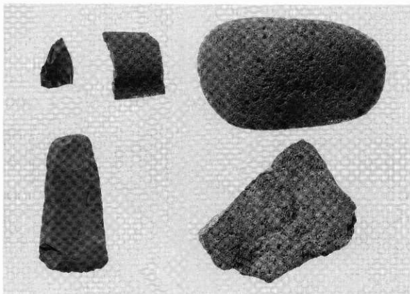
1 P-3の石器
