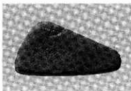
6 すり石④
