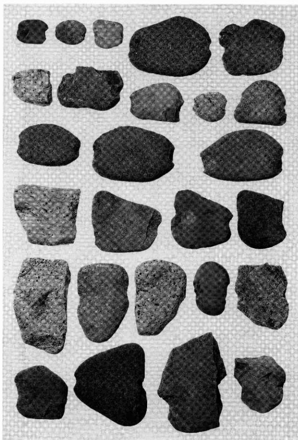
石錘
