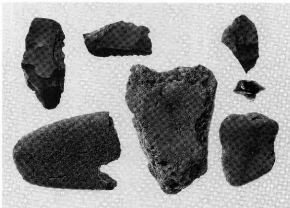
2 H-8の石器
