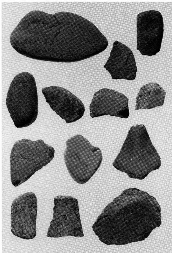
H-4の石器
