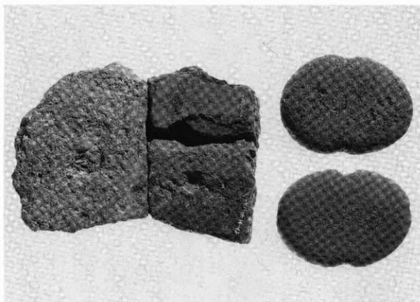
1 H-4の石器
