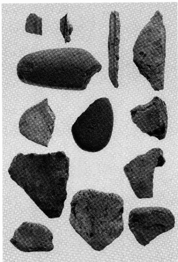
H-5の石器
