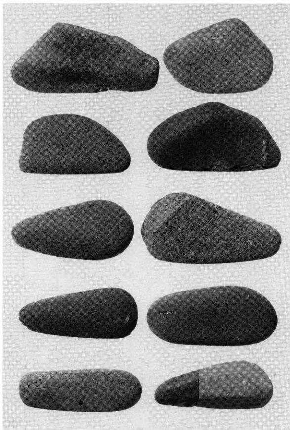
すり石
