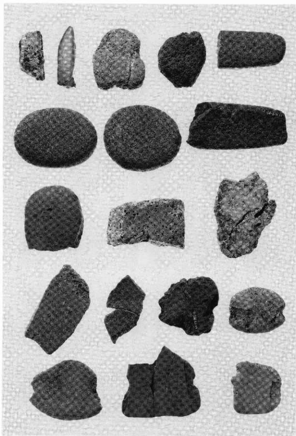
H-9の石器
