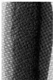
2 たたき石
