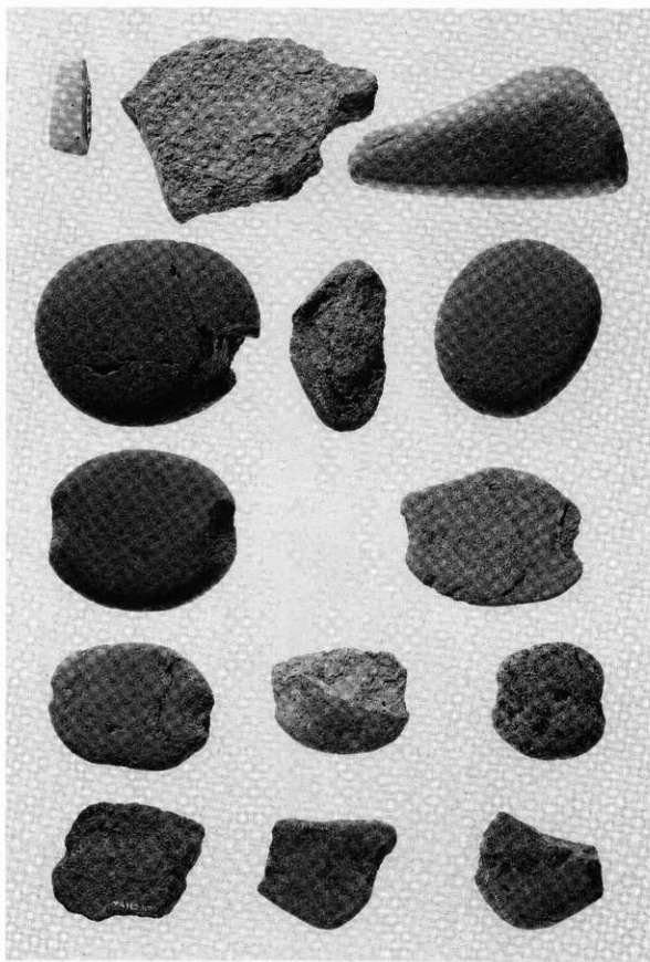
H-2の石器
