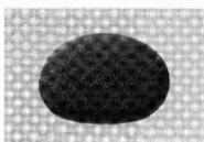
3 すり石①
