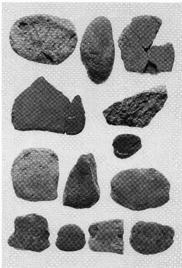
H-6の石器
