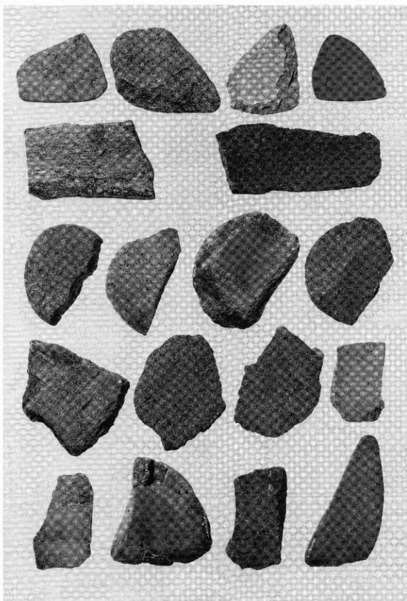
石鏃・砥石
