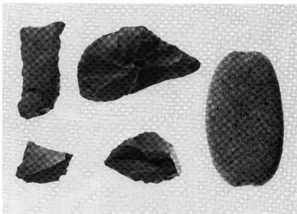
1 H-7の石器
