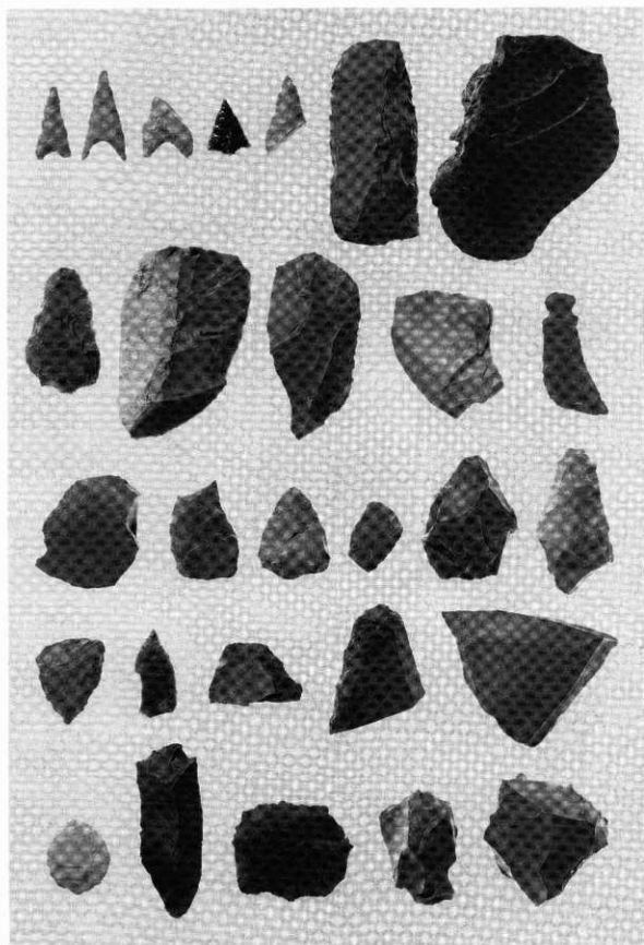
H-9の石器
