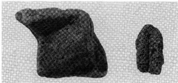
3 石製品②
