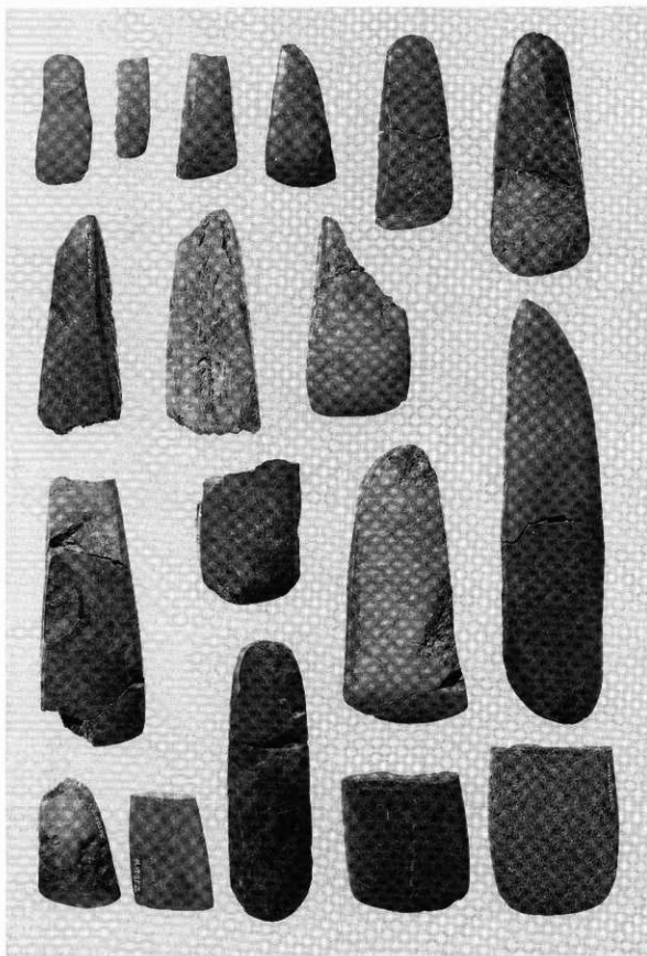
磨製石斧
