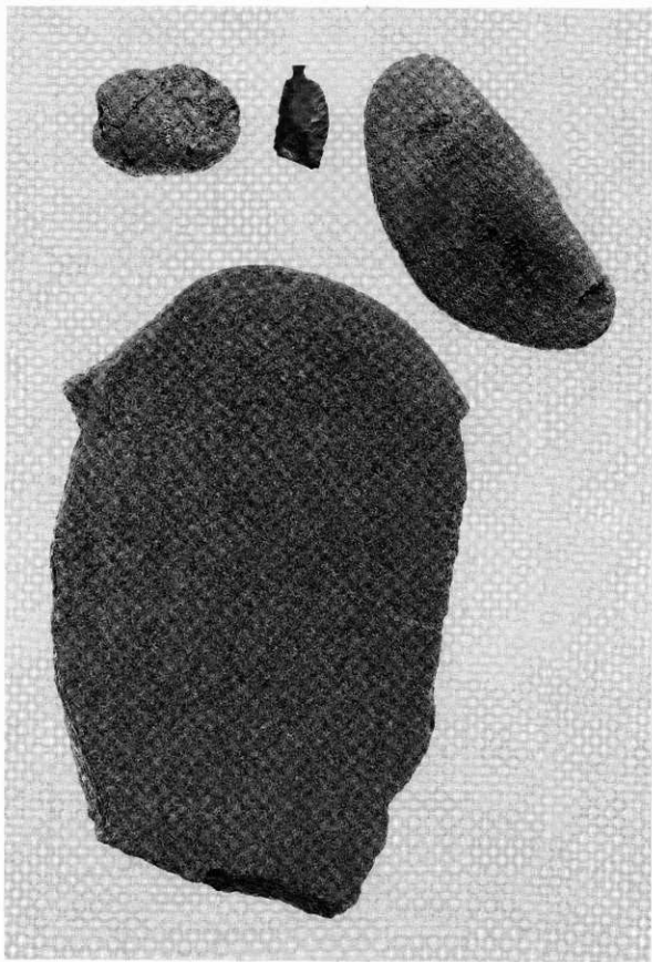
X-1の石器
