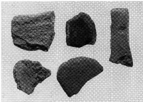
1 H-11の石器
