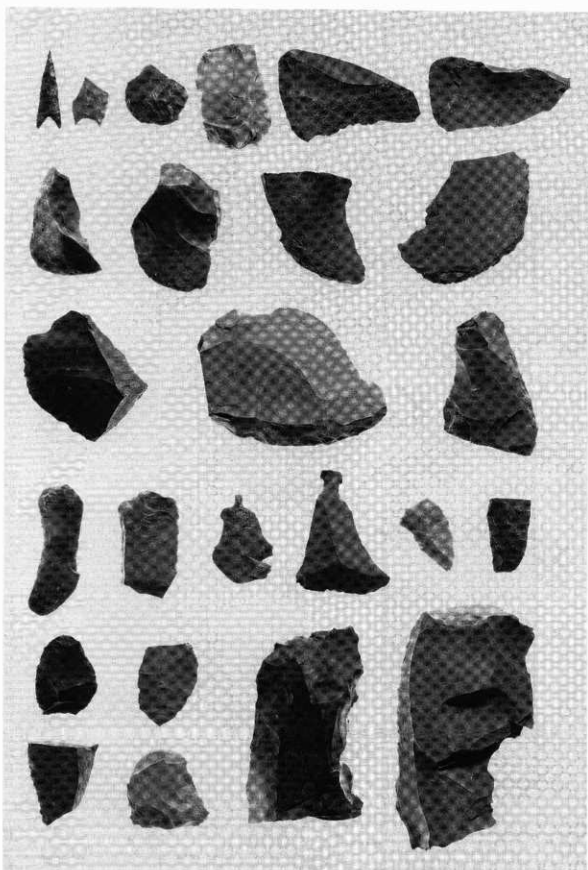
H-5の石器
