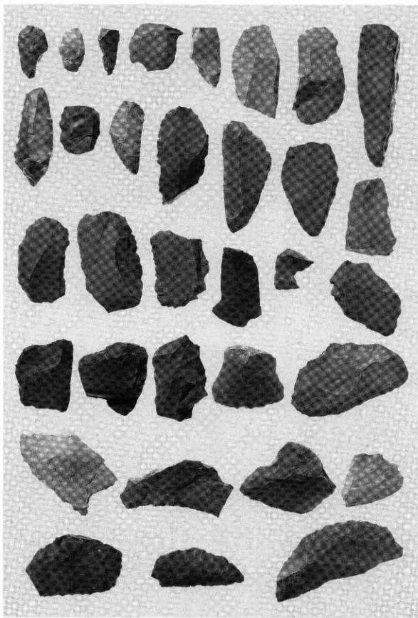
削器
