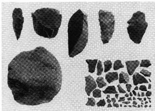
1 H-1の石器
