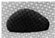
5 すり石③
