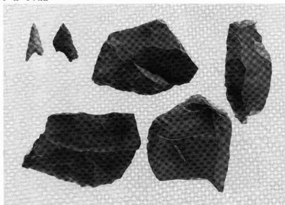
2 H-2の石器
