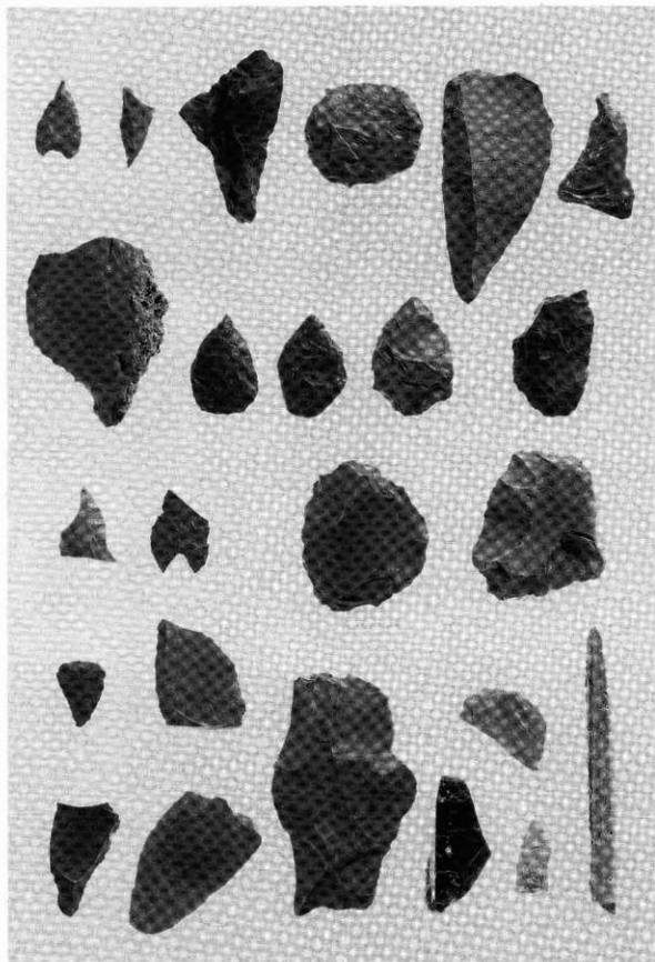
H-3の石器
