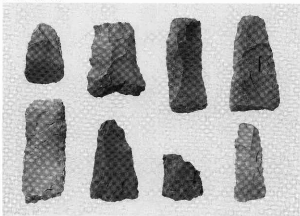
2 簞状石器
