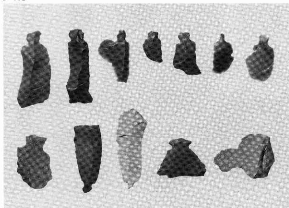
2 石匙形石器
