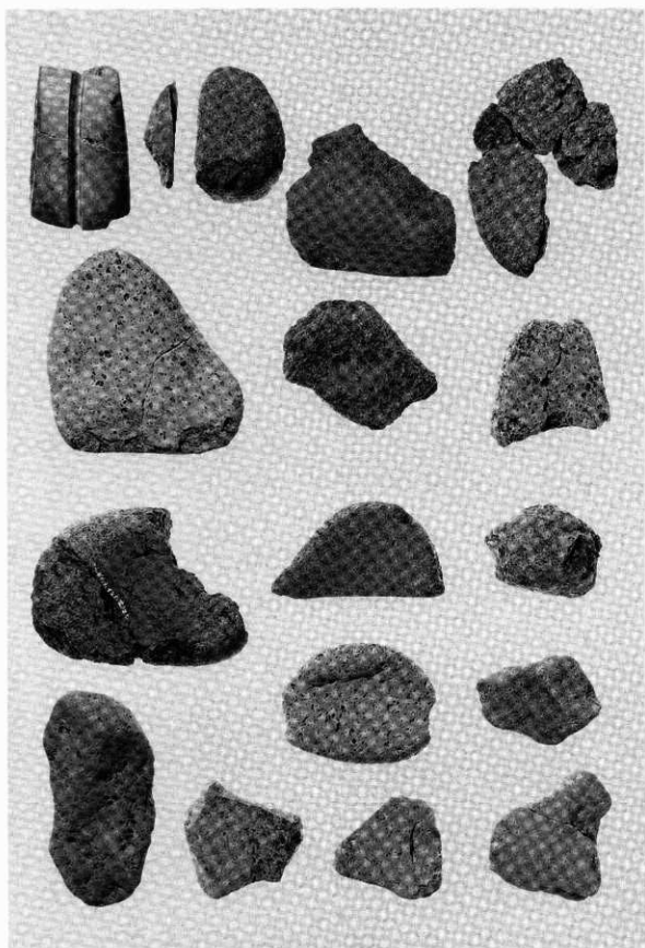
X-2の石器
