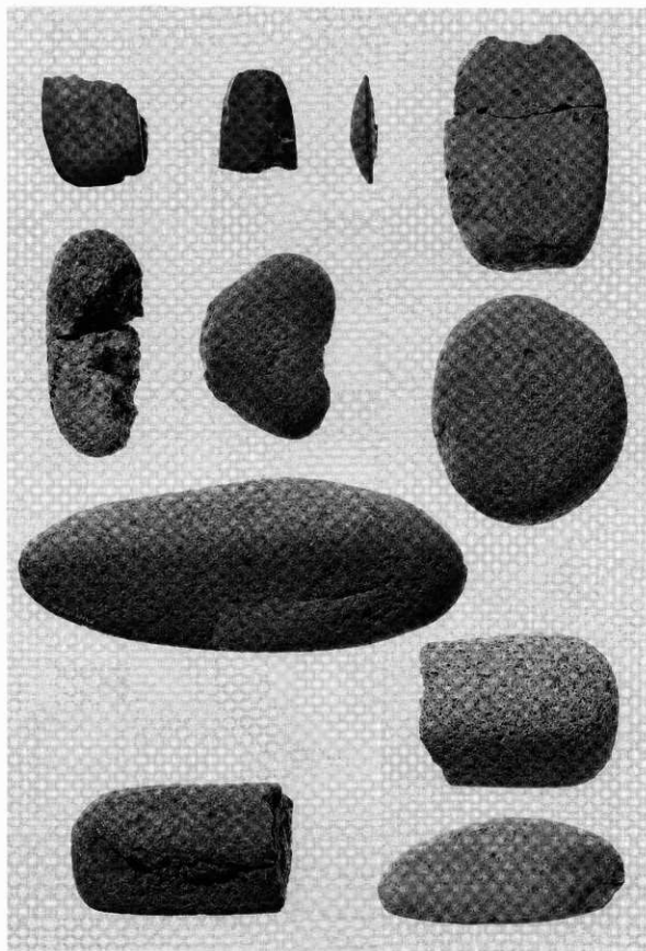
H-4の石器
