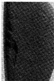
1 鹿状石器
