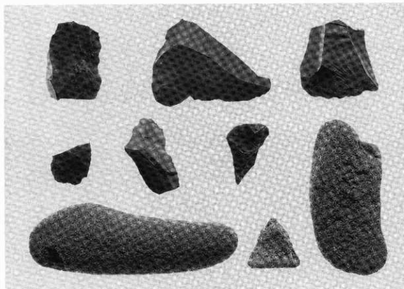
1 H-10の石器
