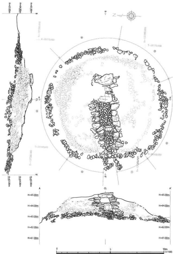
第16图 稻荷山1号墳第3重石積立面平面图
