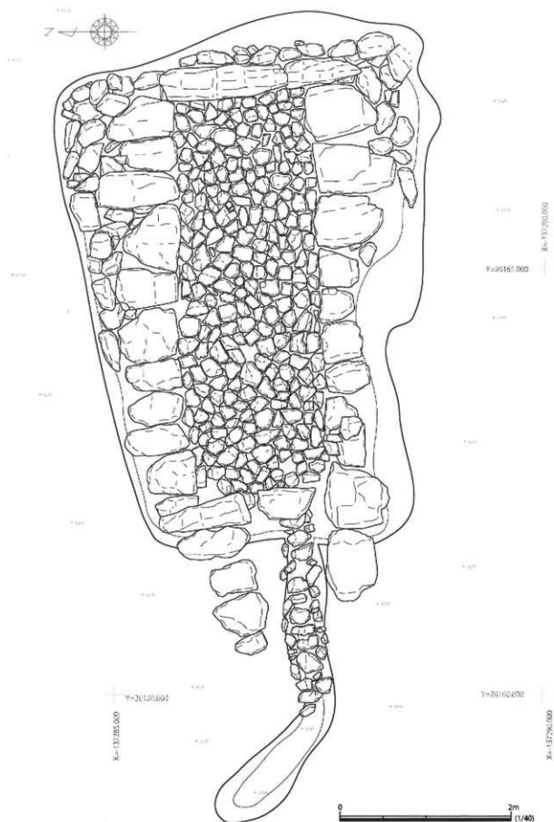
第24図 稻荷山1号墳基底石・敷石・暗渠排水溝図
