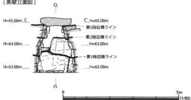
【奥壁立面図】
