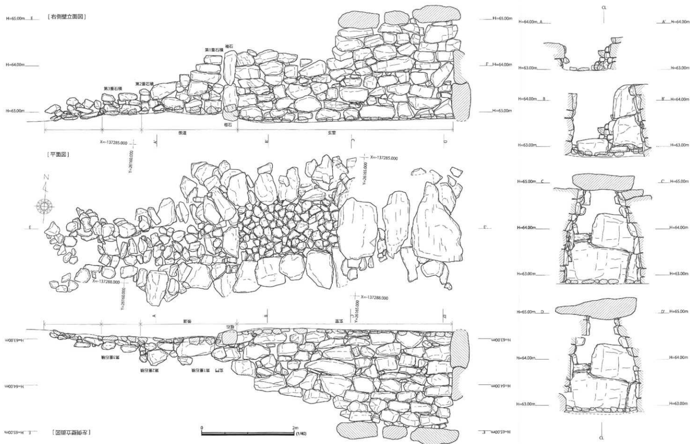
第21图 稻荷山1号墳石室立面平面图
