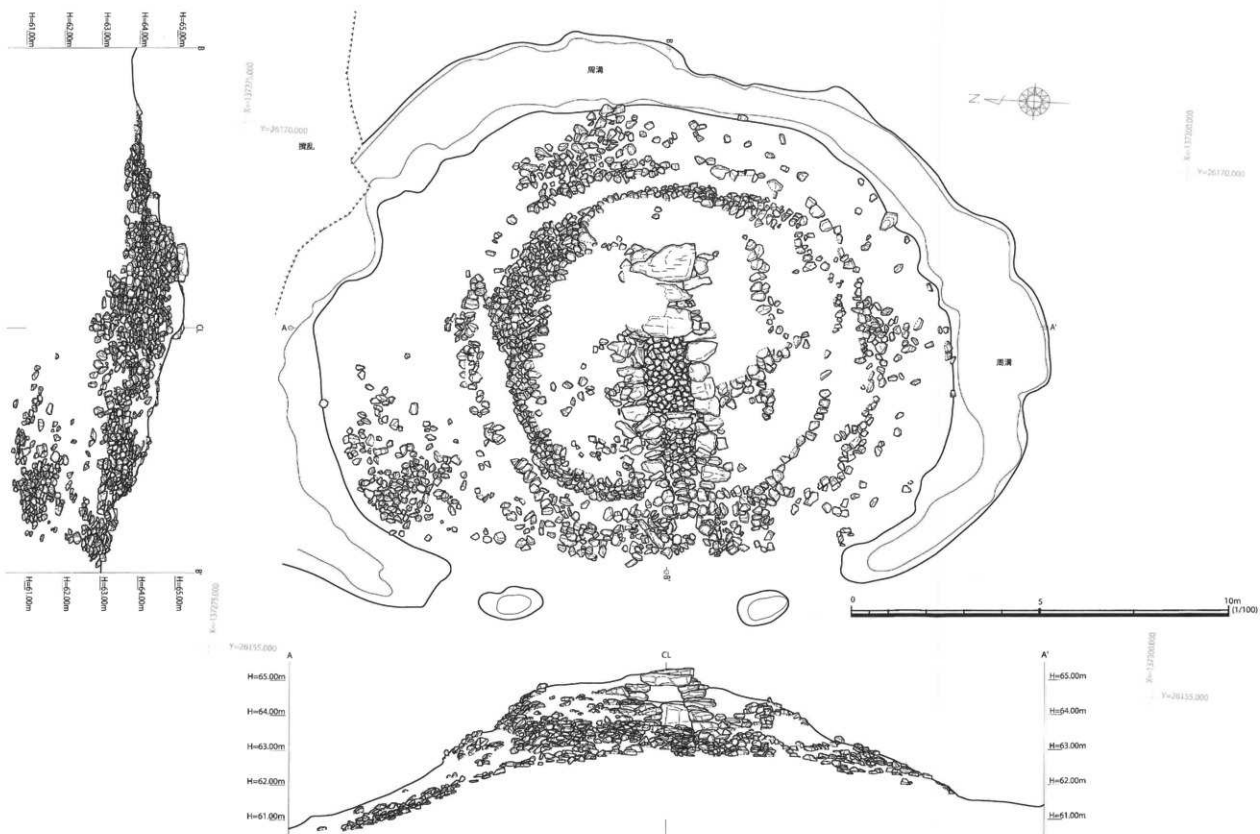
第12図 稻荷山1号墳立面平面図
