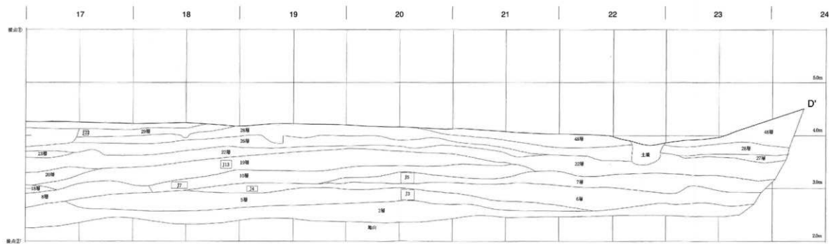
第15図 具層断面図一 3 (1/50)
