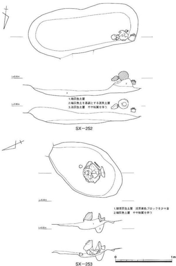
第59図 SX-252・253遺物出土状況図 (1/20)
