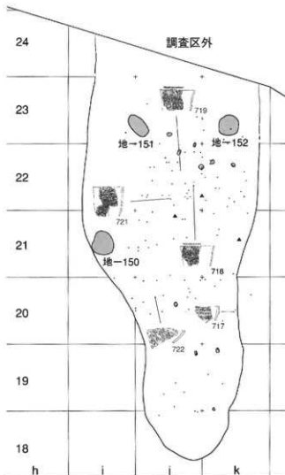
第38図 25層遺構・遺物分布図 (1/100)
