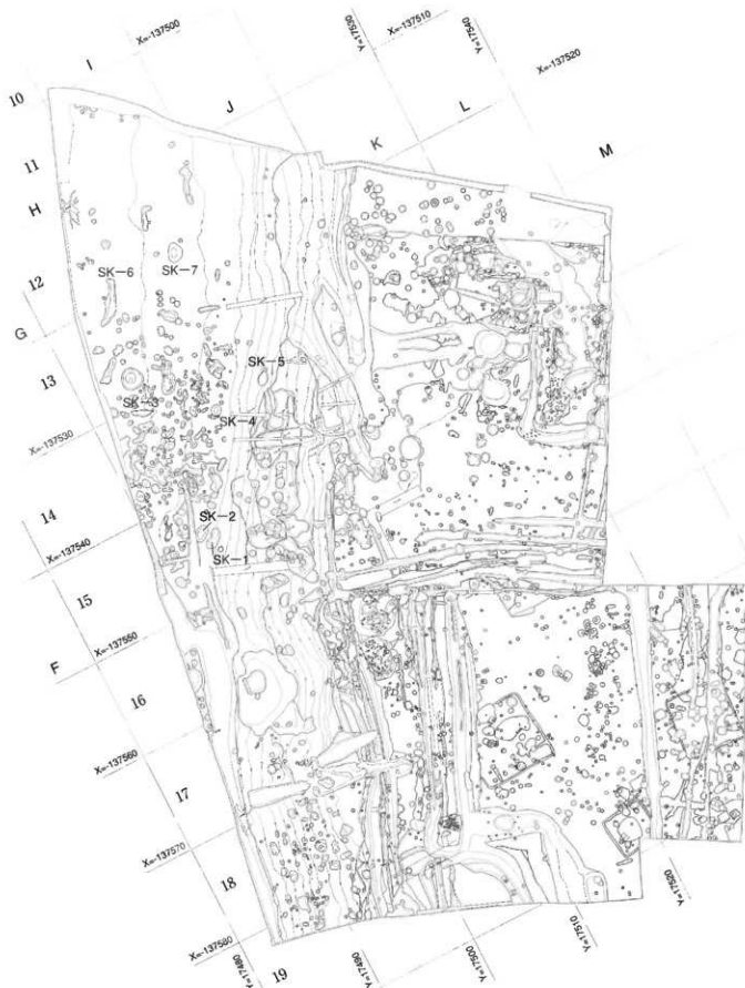
第7図 貝塚基盤（地山）測量図（1/400）
