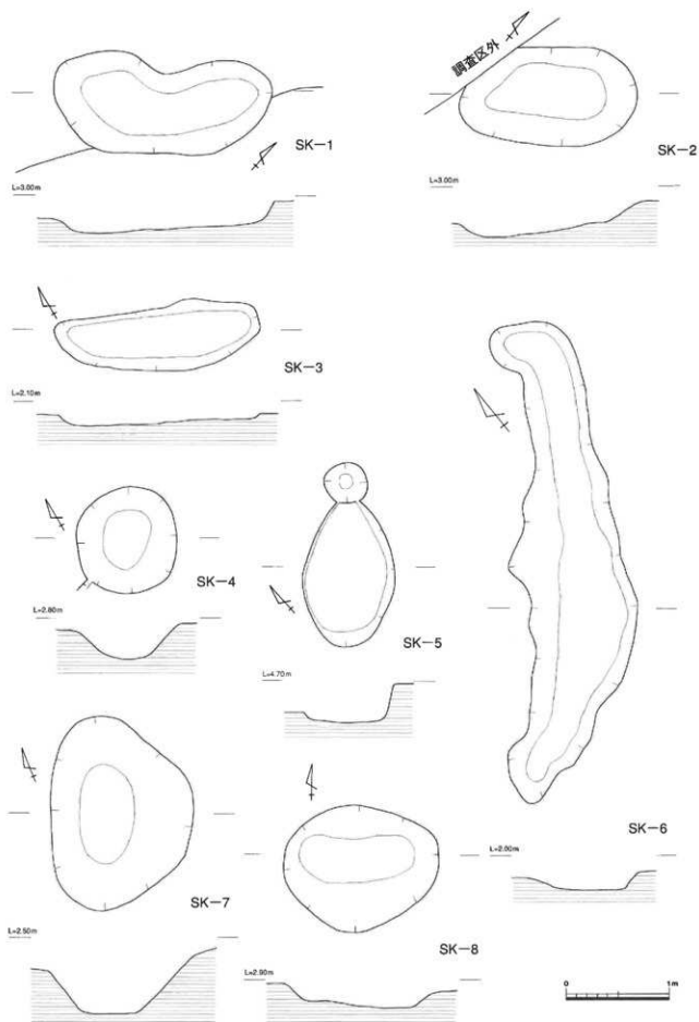
第56図 土壌実測図 (1/40)
