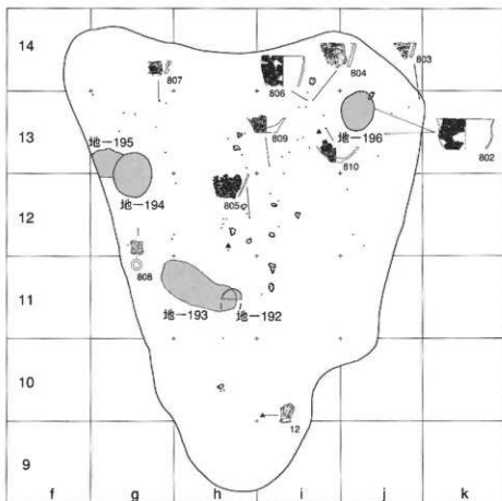
第50図 38層遺構・遺物分布図 (1/100)
