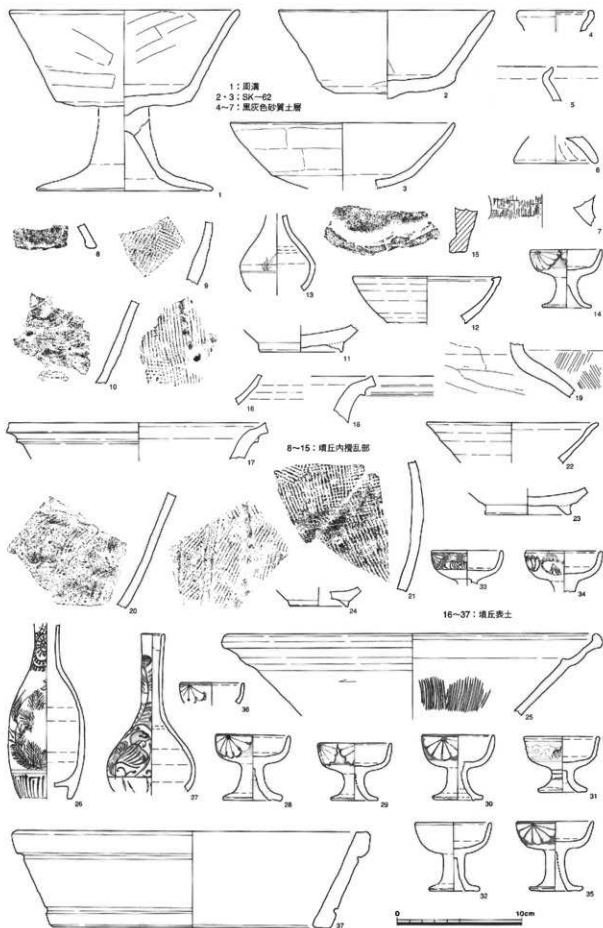
第34図 洗島1号墳出土遺物実測図-1 (1/3)
