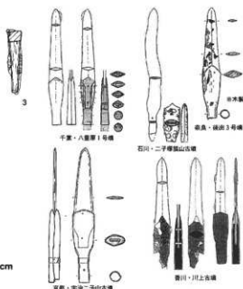
第36図 ヤリ類似例集成 (1/10)
