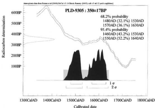
第38図 火葬墓炭化材の暦年較正図
