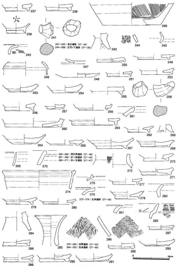
第25図 採集遺物実測図-6 (1/3)
