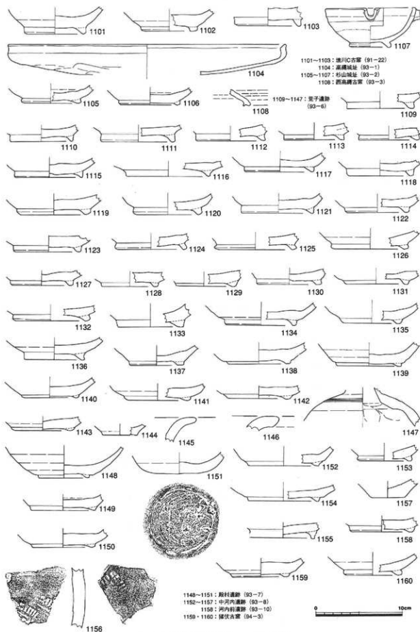
第46図 採集遺物実測図-27 (1/3)
