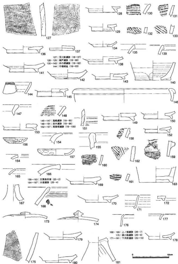
第23図 採集遺物実測図-4 (1/3)
