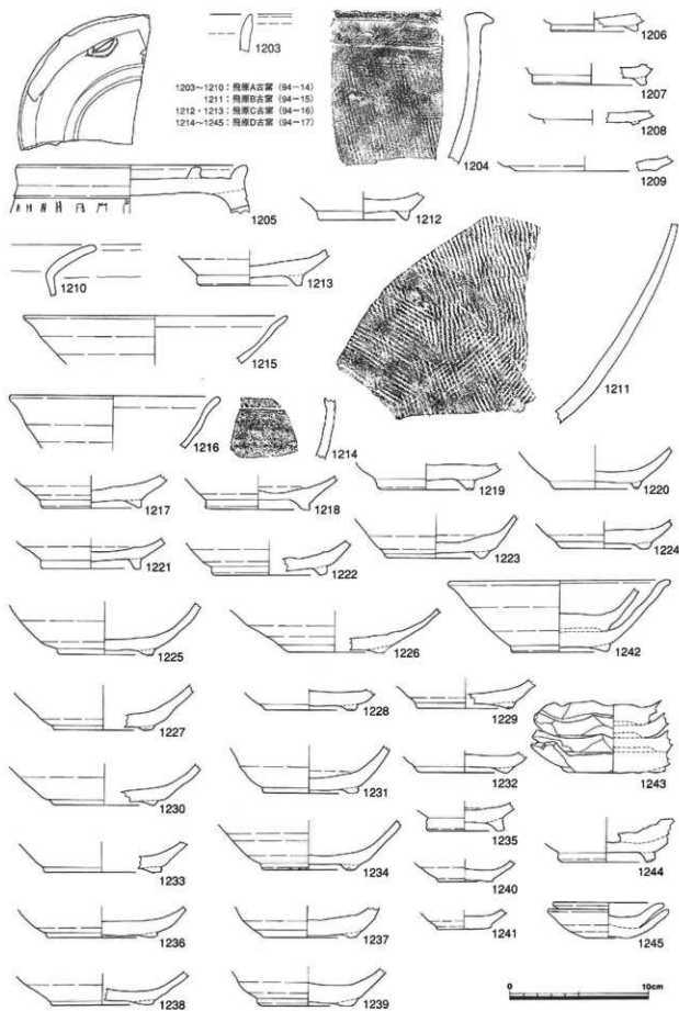
第48図 採集遺物実測図-29 (1/3)
