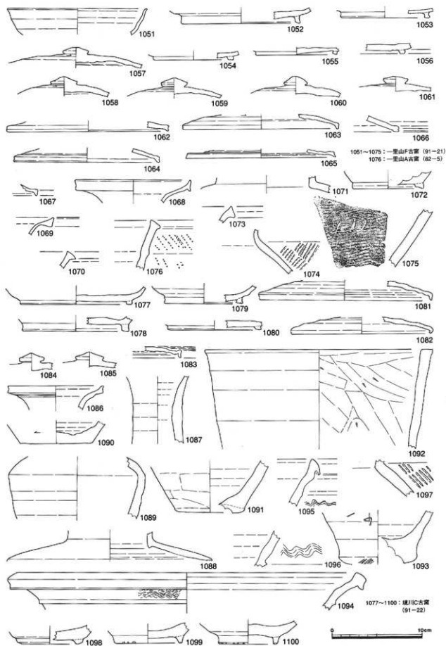
第45図 採集遺物実測図-26（1／3）
