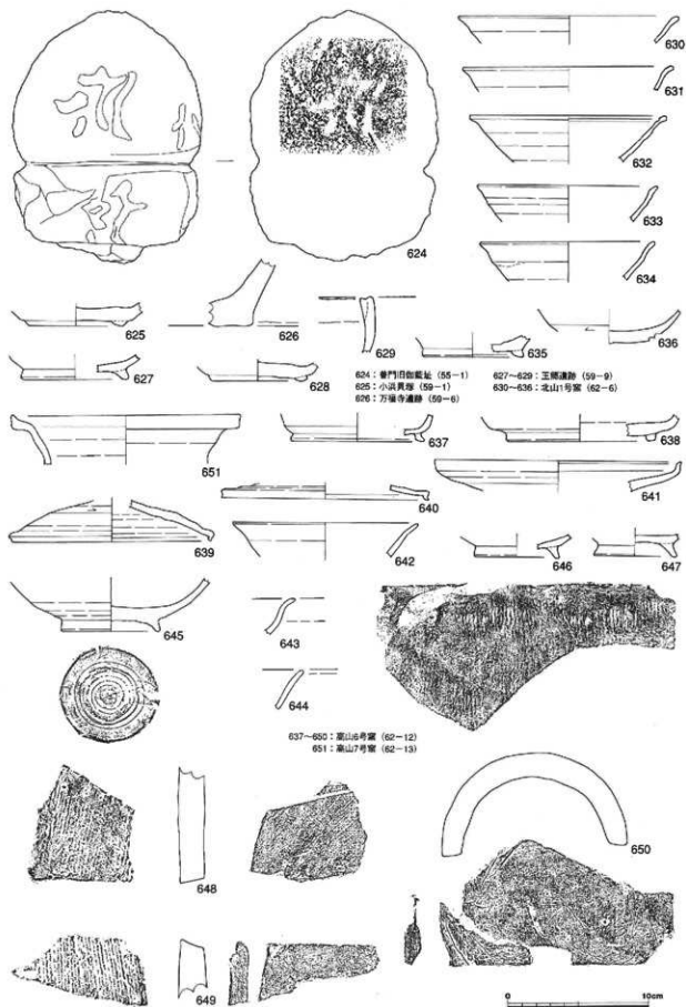
第35図 採集遺物実測図-16 (1/3)
