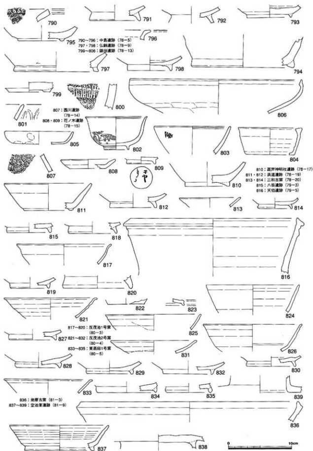
第39図 採集遺物実測図-20 (1/3)
