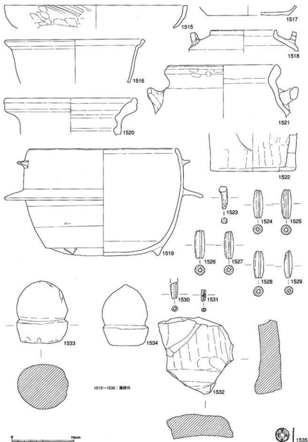
第55図 採集遺物実測図-36 (1/3)
