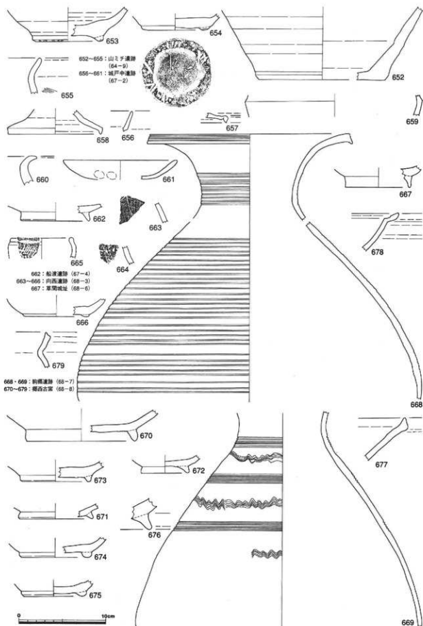
第36図 採集遺物実測図-17 (1/3)
