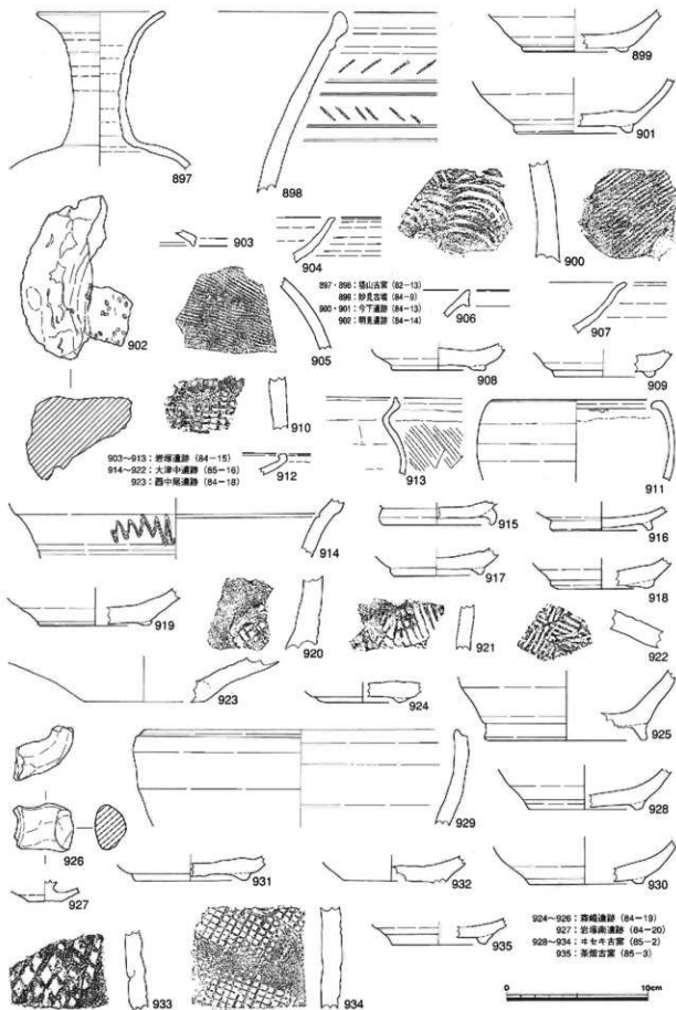
第41図 採集遺物実測図-22（1／3）
