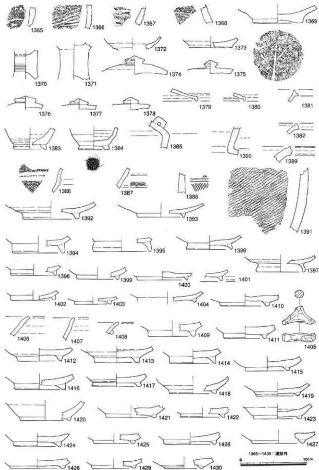
第52図 採集遺物実測図-33 (1/3)
