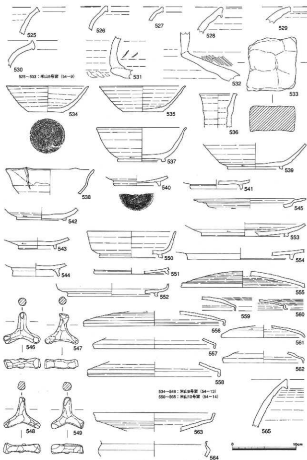
第32図 採集遺物実測図-13 (1/3)
