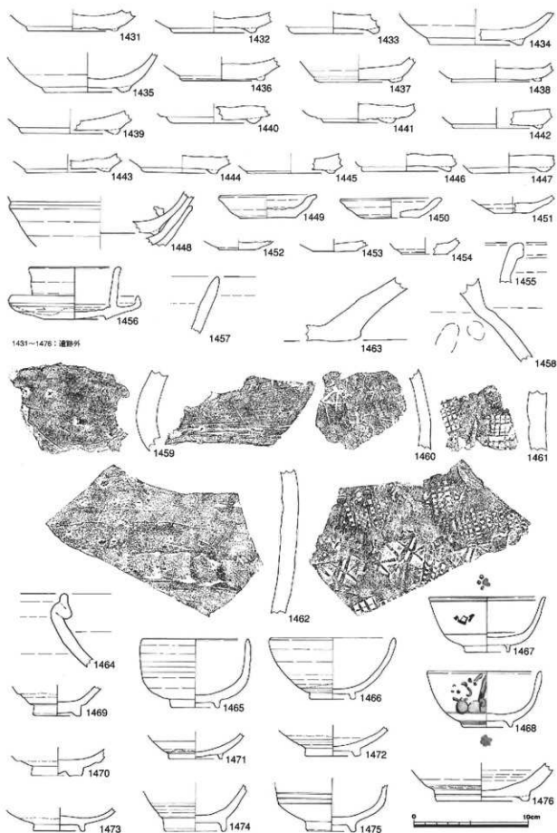
第53図 採集遺物実測図-35 (1/3)
