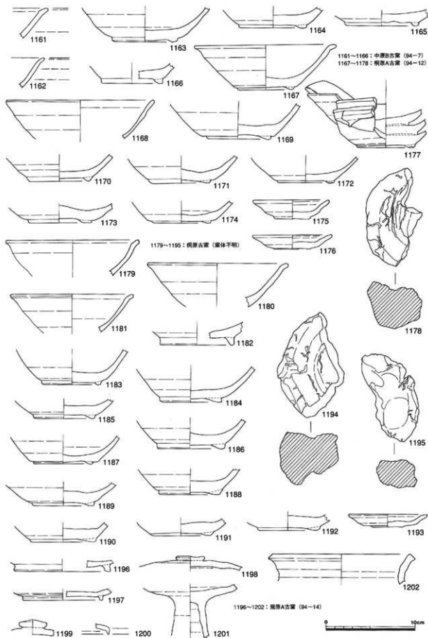
第47図 採集遺物実測図-28 (1/3)
