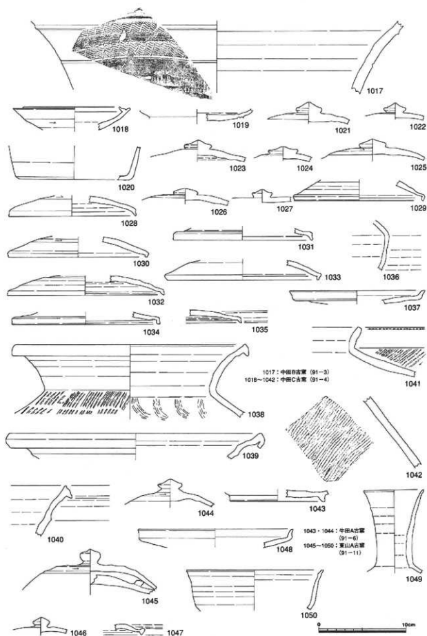
第44図 採集遺物実測図-25 (1/3)
