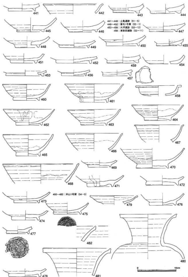
第30図 採集遺物実測図-11 (1/3)
