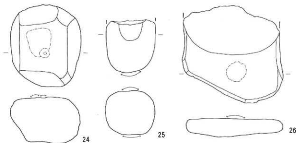
24・26: S Z - 1・東溝
