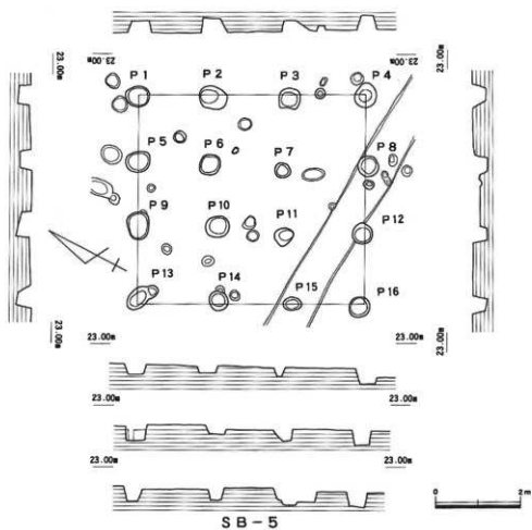
SB-4・5実測図 (1/100)
