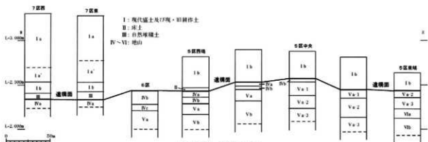
第5図 基本層序
