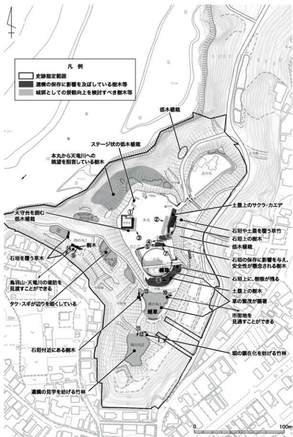
Fig.66 二侯城跡植栽現況図
