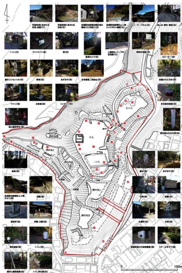
Fig.70 二俣城跡建築物・工作物等現況図
