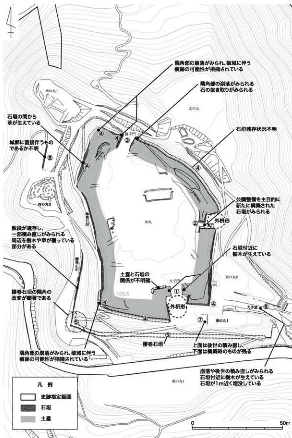
Fig.63 鳥羽山城跡石垣現況図
