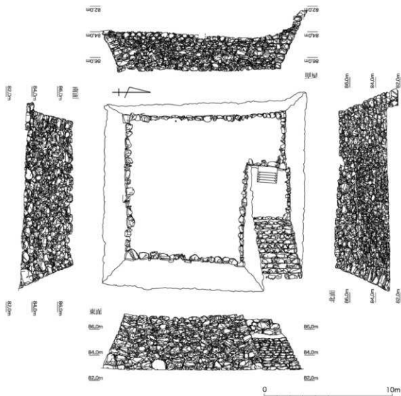
Fig.47 天守台の構造
