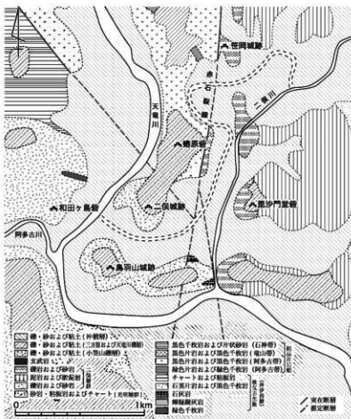
Fig.6 二保城跡及び鳥羽山城跡周辺の地質図
