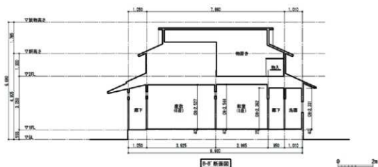
〔図 3-17〕 離れ断面図 (S=1:150)
