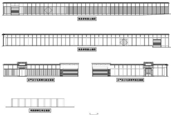
〔图 3-8〕 正門・高塀・南西部煉瓦塀立面図 (S=1:300)
