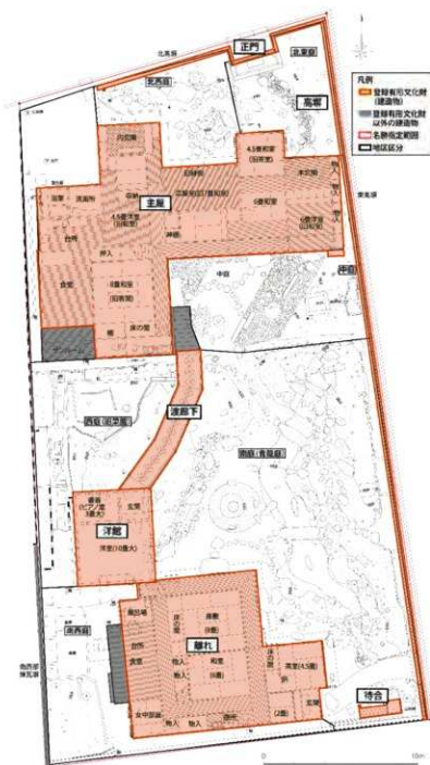
〔図 3-7〕 建造物配置図
