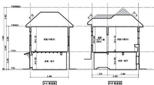
〔图 3-15〕 洋館立面図・断面図 (S=1:150)
