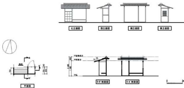
〔図 3-18〕 待合立面・断面図 (S=1:150)
