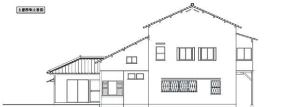
主屋東側立面図
