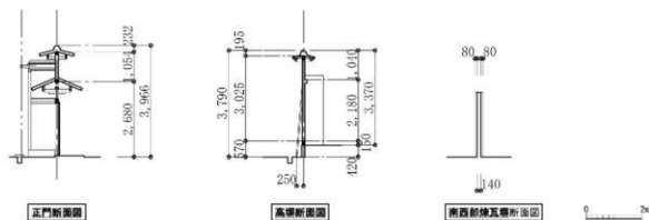
〔图 3-9〕 正門・高塀・南西部煉瓦塀断面図 (S=1:150)
