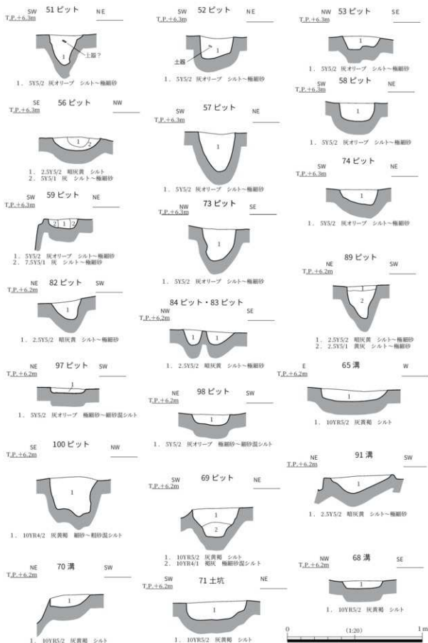
図 15 1区第4面遺構断面図(2)
