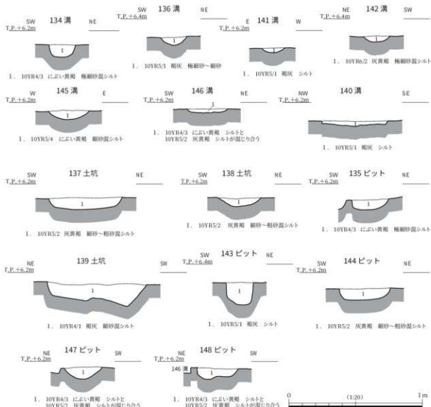
図 17 2 区第 2 面遺構断面図
