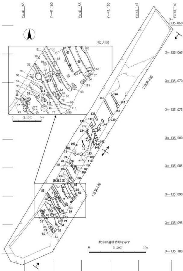
図 13 1区第4面・2区第2面平面図
