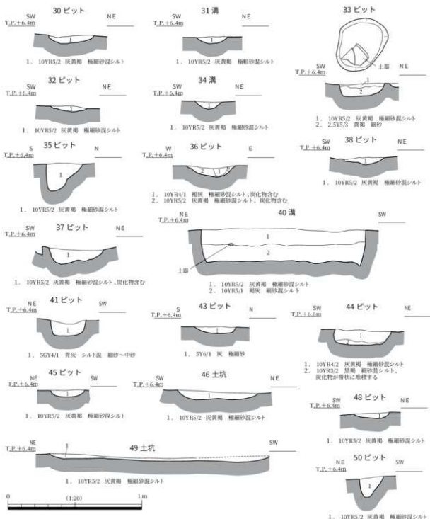
図 11 1区第3面遺構断面図
