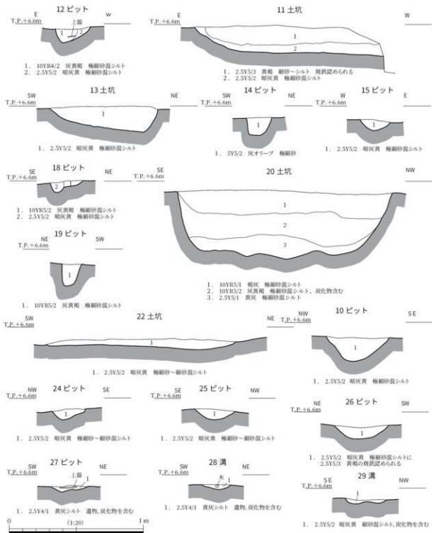
図9 1区第2面遺構断面図
