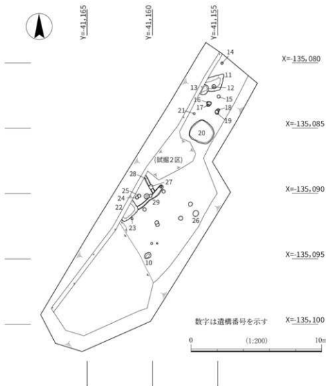
図8 1区第2面平面図
