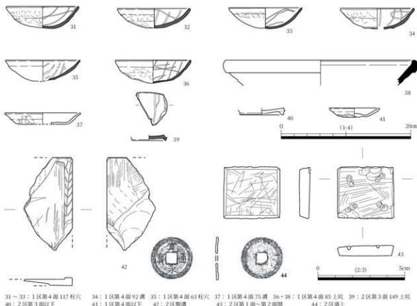
図 22 1区・2区出土遺物実測図(2)
