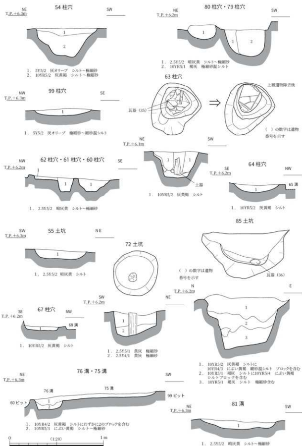
図 14 1区第4面遺構断面図(1)
