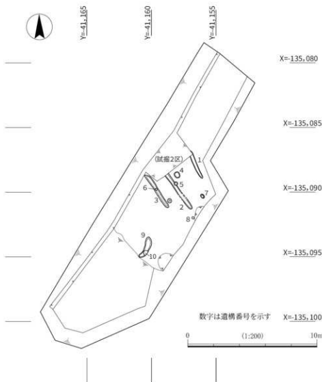
図6 1区第1面平面図
