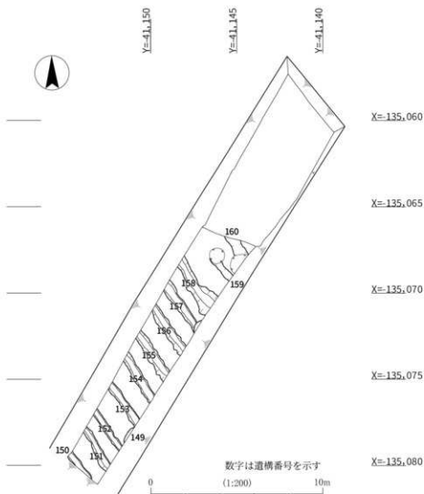
図 18 2区第3面平面図 150・151・152 溝
