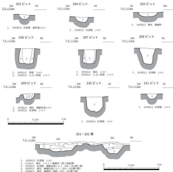
図 25 4区第2面遺構断面図
