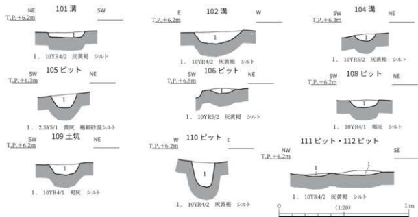
図 16 1区第4面遺構断面図(3)
