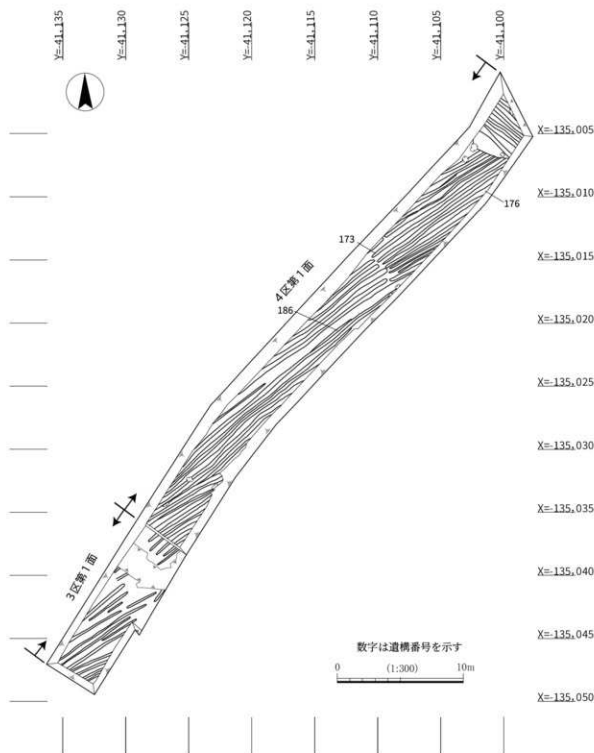
図23 3区第1面・4区第1面平面図
