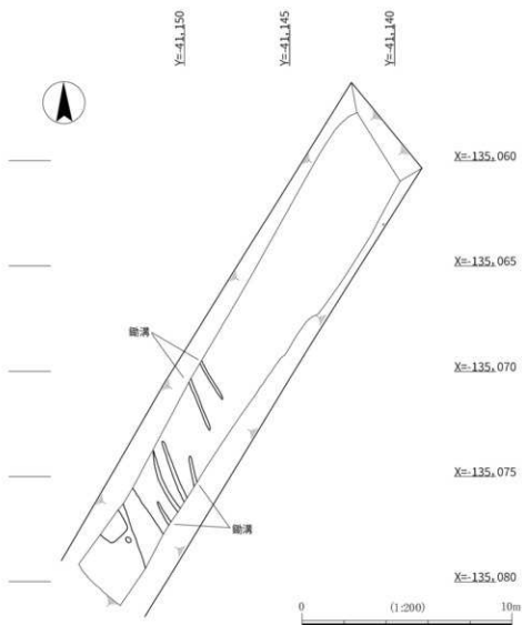
図 20 2区第4面平面図
