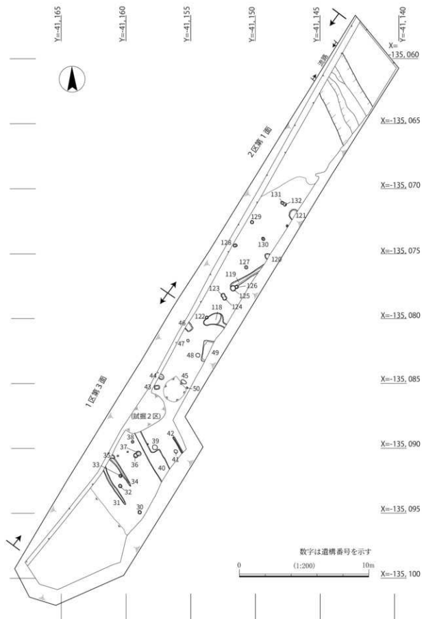
図 10 1区第3面・2区第1面平面図
