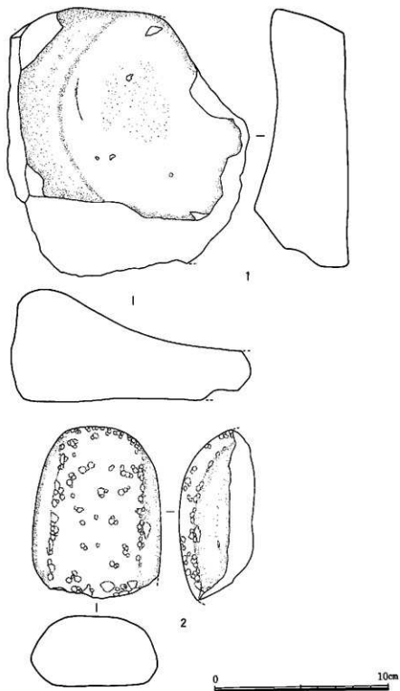
図3 並里遺物散布地採集の石皿(1)、すり石(2)
