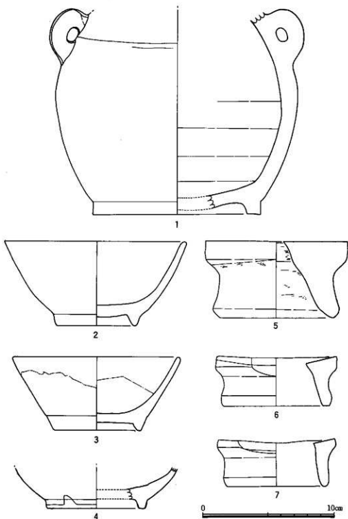
図9 屋敷窯跡採集の陶器(1~4)・窯道具(5~7)
