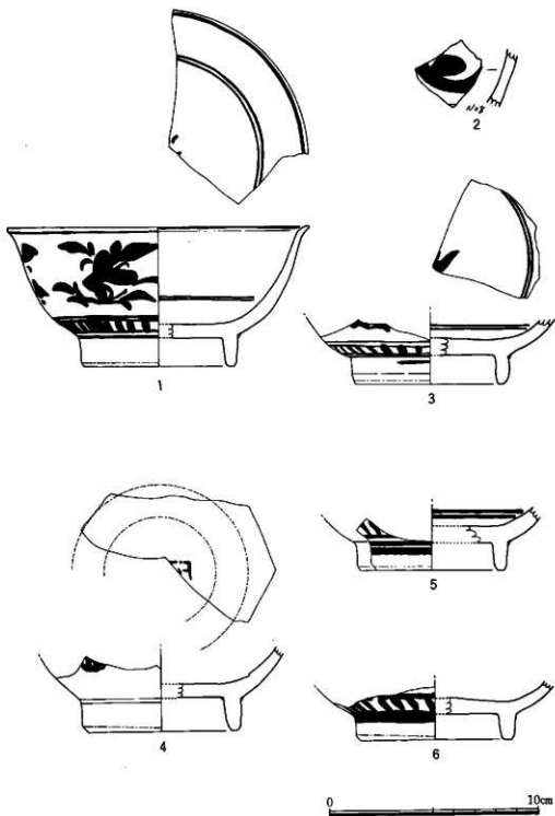
図4 大川原遺物散布地(1~3)、トゥムスズ御嶽遺跡(4~6) 採集の染付
