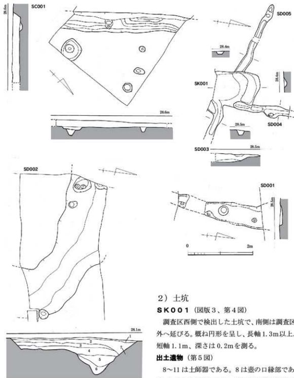
第4図 遺構実測図 (1/60)
