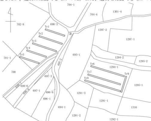
全体図 (1 : 1,000)
