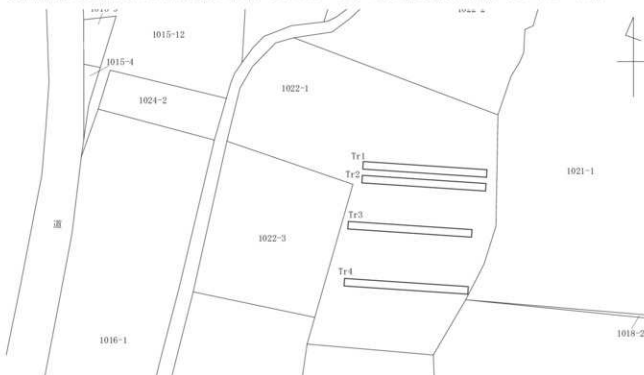
全体図 (1 : 500)
