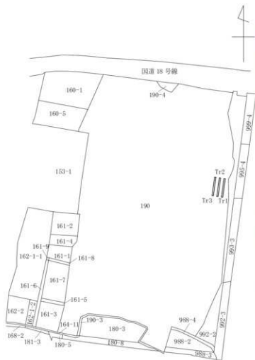
全体図 (1 : 2,000)
