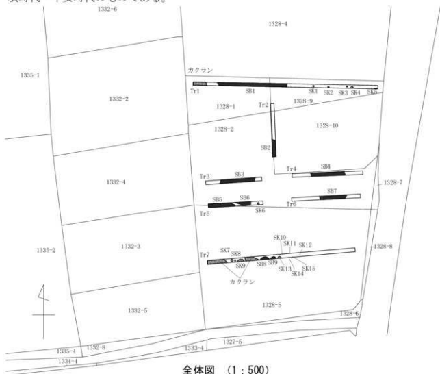
全体図 (1 : 500)
