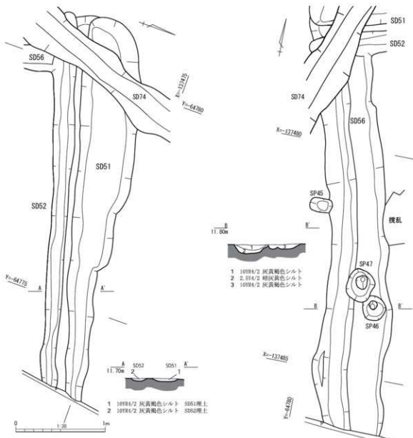
Fig. 37 SD51・52・56 平面・断面図 (S-1/30)
