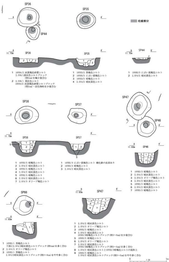
Fig. 33 小穴群各遺構平面・断面図 (S=1/30)
