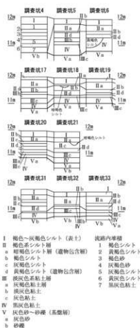
Fig. 8 土層柱状図 (S=1/100)
