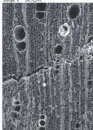
横断面 0.1 mm
