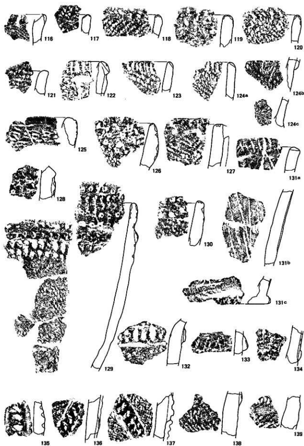
図VI-48 土器(8)
