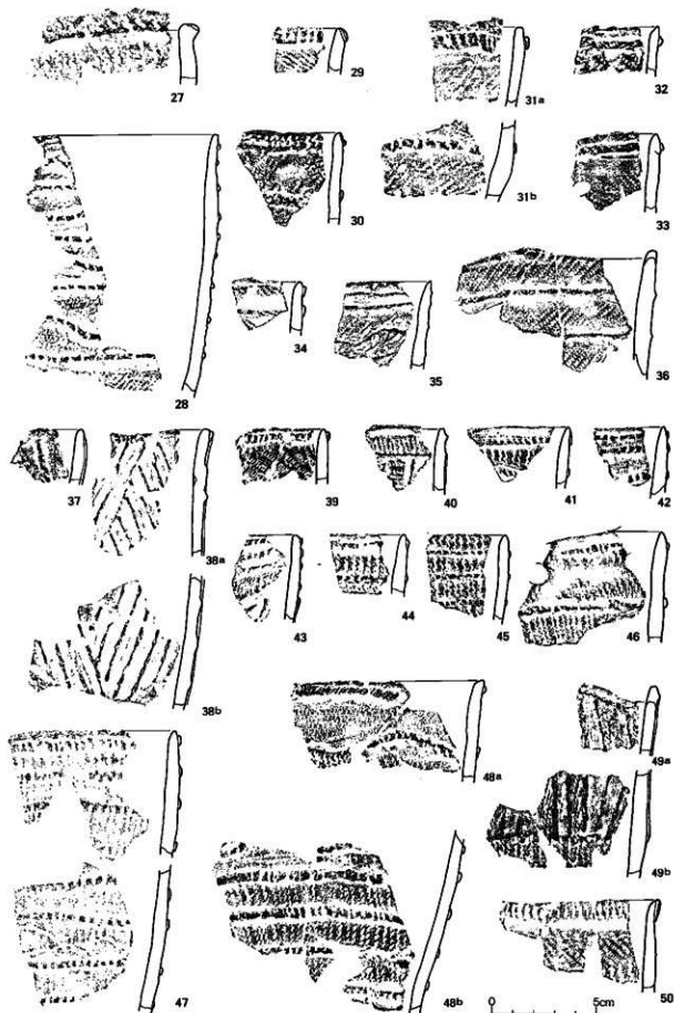
圖 VI-44 土器(4)
