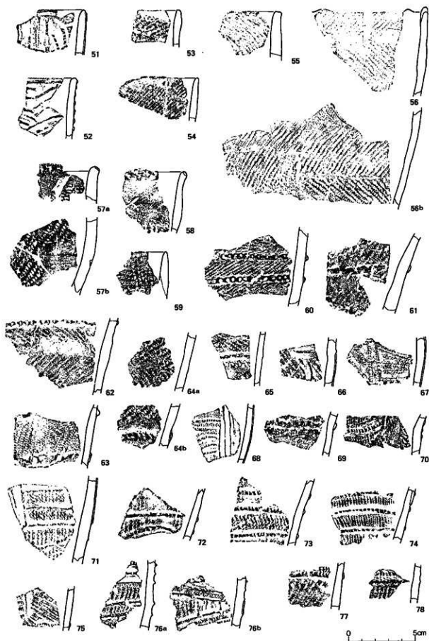
圖VI-45 土器(5)
