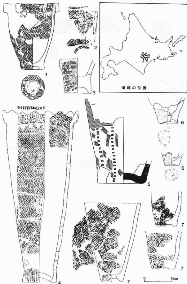
図1 あげ底の土器(1)と遺跡の位置
