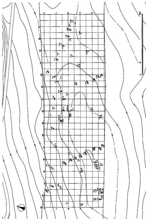
図VI-6 遺構の位置
