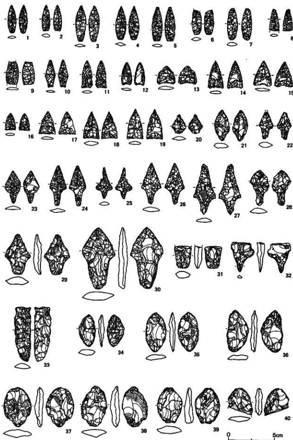
図VI-52 石器(1)
