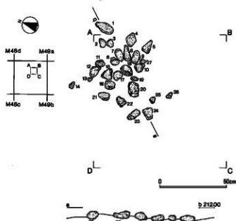
図IV-9 礫集中S-2
