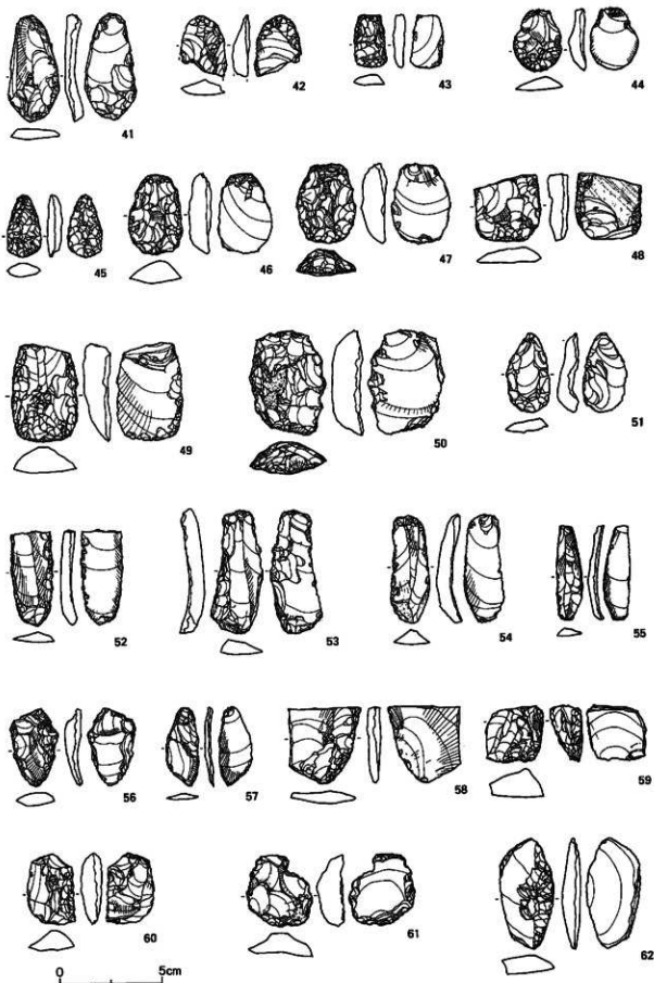
图 VI-53 石器(2)
