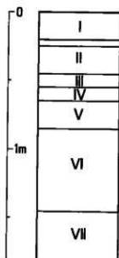
図IV-5 土層柱状図
