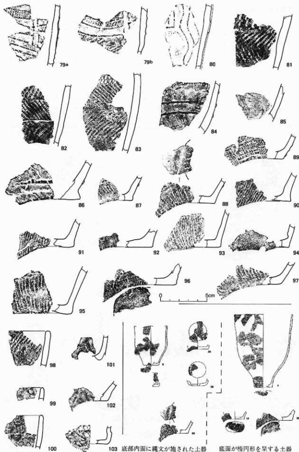
図VI-46 土器(6)
