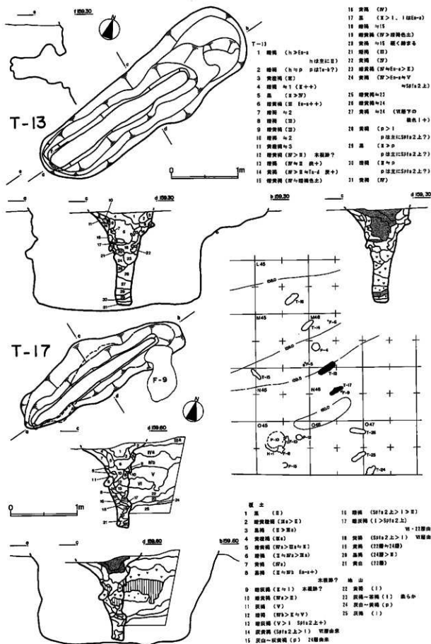
図VI-21 T-13・T-17
