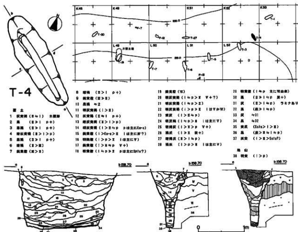
図VI-32 T-4
