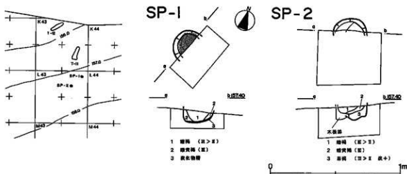
図VI-16 SP-1・SP-2
