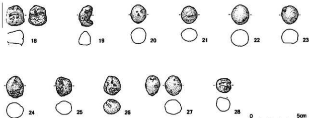
図VI-10 P-4の遺物
