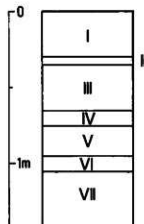
図V-4 土層柱状図
