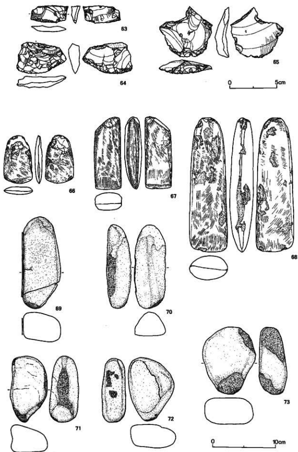
図VI-54 石器(3)
