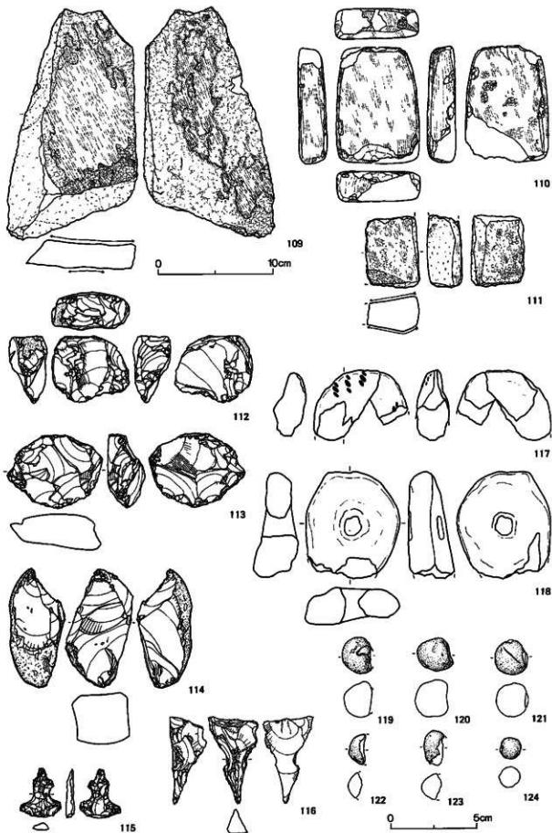
圖VI-59 石器(8)
