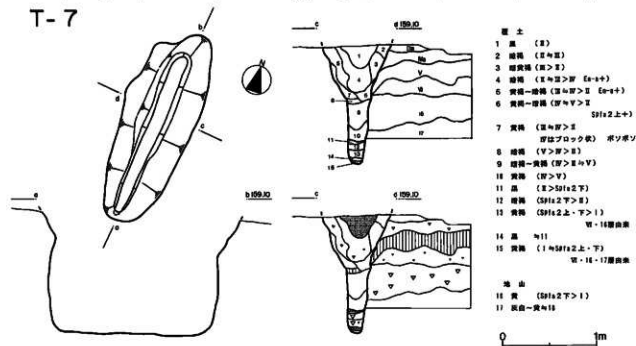
図VI-34 T-6・T-7
