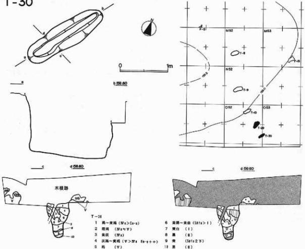
図VI-26 T-29・T-30
