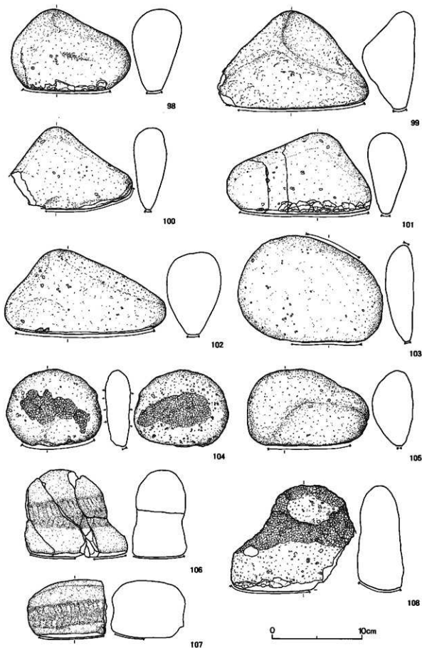
図VI-58 石器(7)
