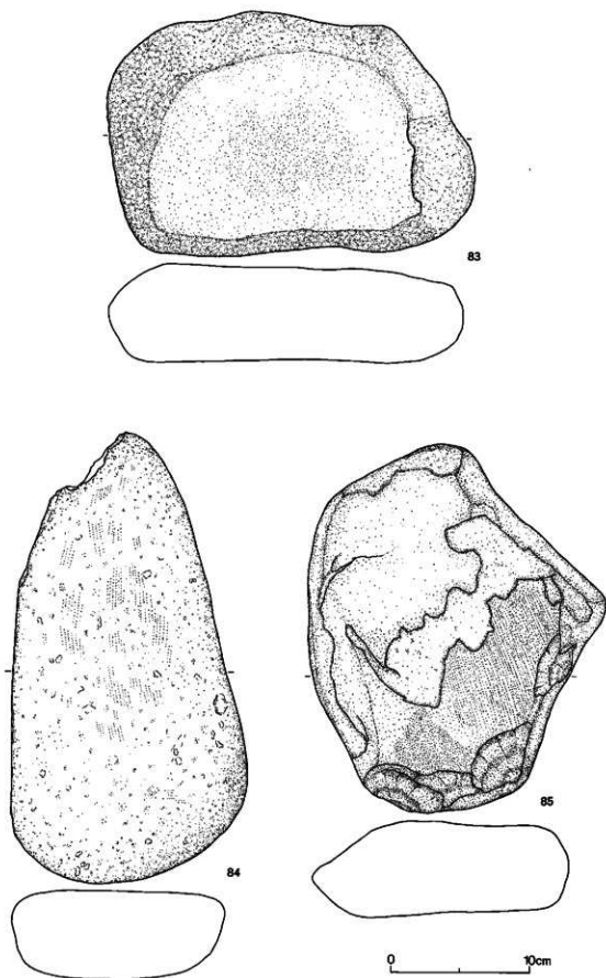
図VI-56 石器(5)
