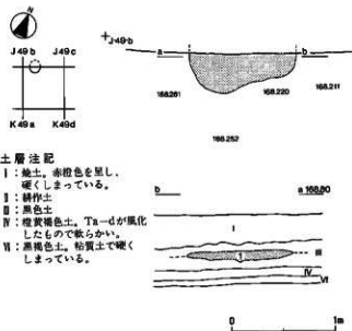
図V-5 焼土 F-1
