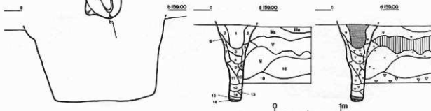
図VI-33 T-3・T-5
