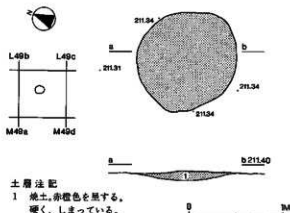
図IV-6 焼土 F-1
