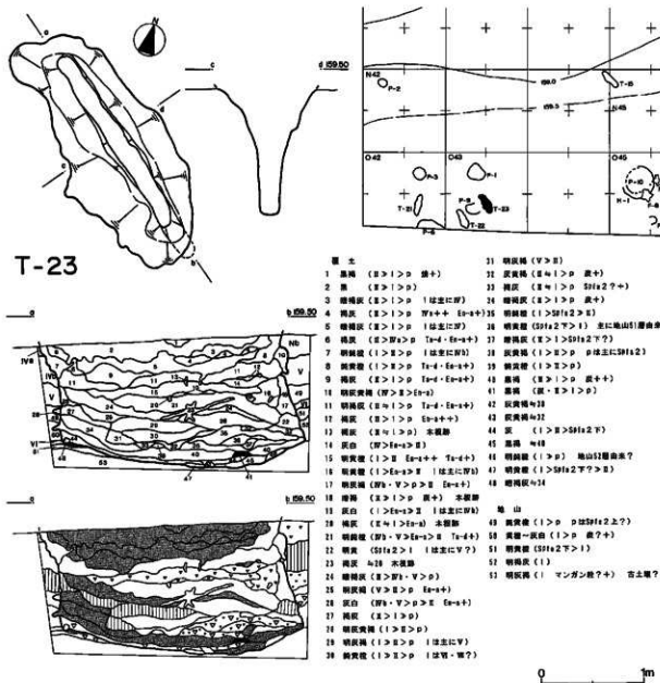
図VI-31・T-23
