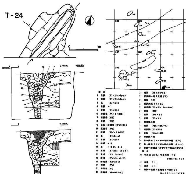
図VI-23 T-24
