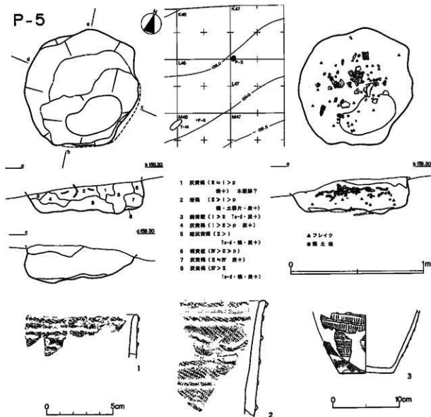
図VI-11 P-5と遺物
