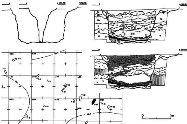
图 VI-29 · T-28
