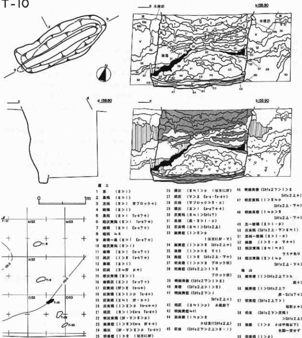
図VI-25 T-10
