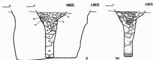
図VI-20 T-16・T-14
