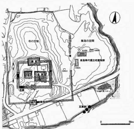
第6図 海会寺の伽藍地と寺院地
