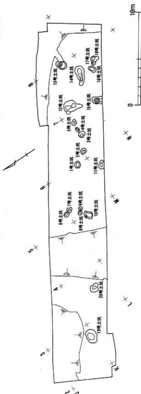
第6図 2区全体図
