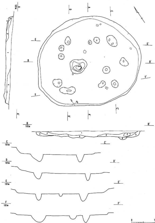
第 12 图 3 区第 2 号住居跡 实测图
