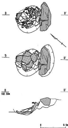
第 11 図 3 区第 1 号住居跡 炉実測図
