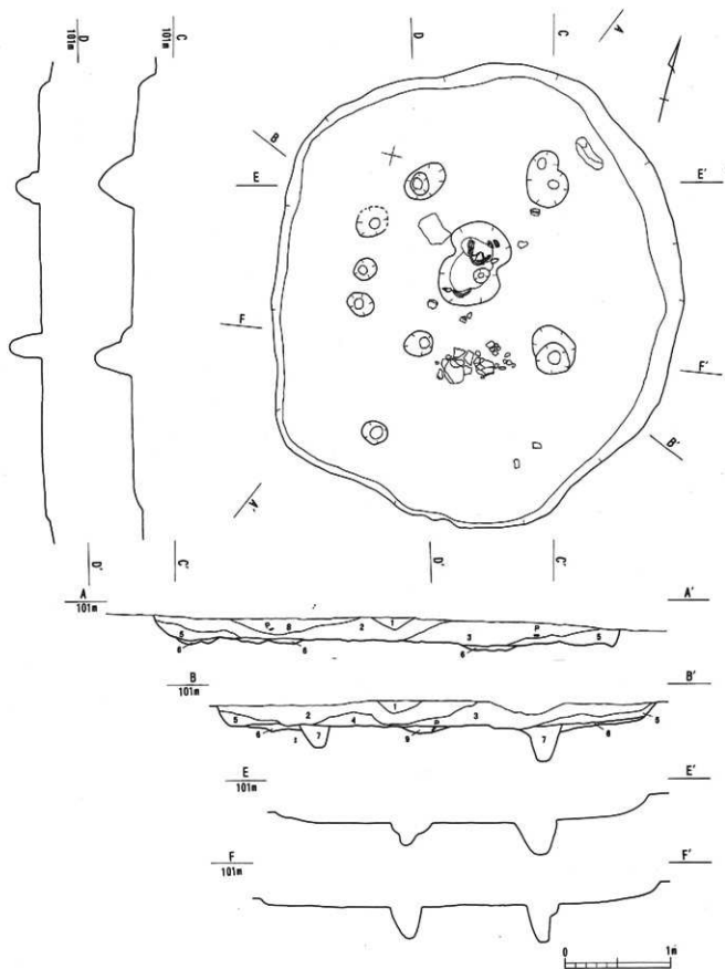
第13图 3区第3号住居跡 实测图
