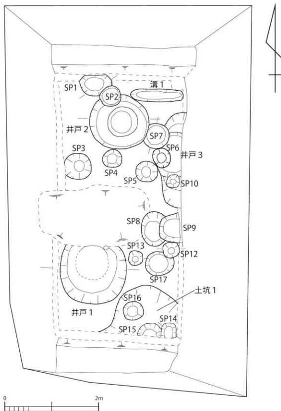
第5図 調査区平面図 (1:40)
