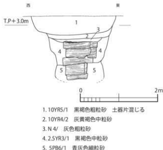
第11図 井戸2 断面図（1：50）
