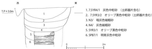
第6図 井戸1断面図 (1:50)
