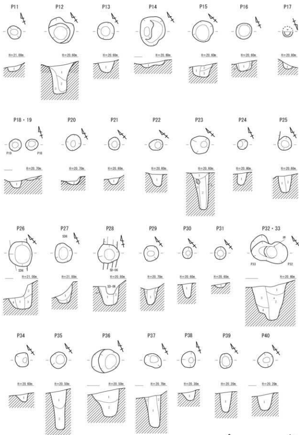
第9图 P-11~40实测图(S=1:30)
