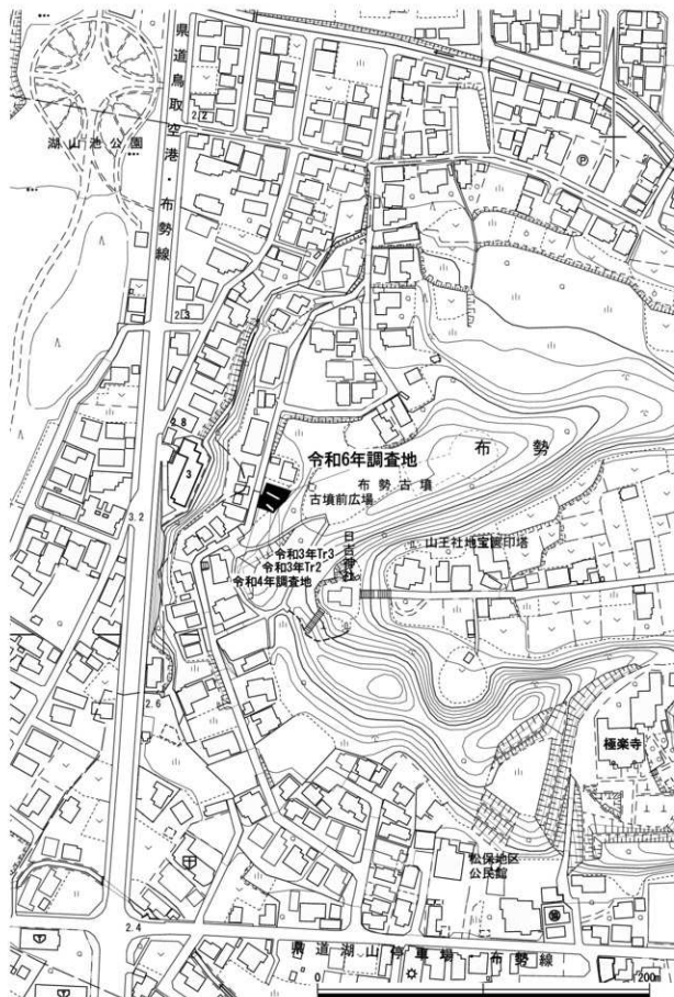
第1図 布勢遺跡調査地位置図(S=1 : 2,500)
