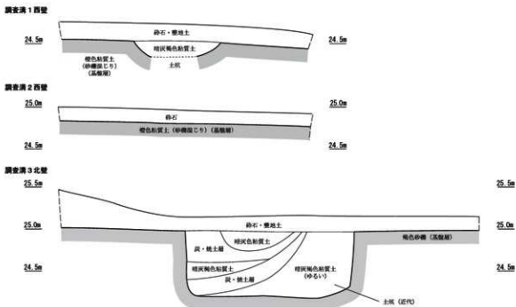
土層柱状図 (S=1/40)
