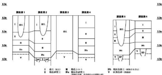
第2図 14次調査土層柱状図
