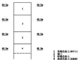
土層柱状図 (S=1/40)
