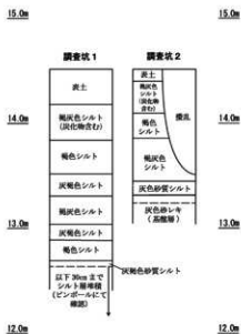
土層柱狀圖 (S=1/40)
