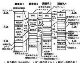
土層柱状図 (S=1/80)
