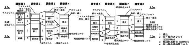
土層柱状図 (S=1/80)
