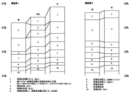
土層柱状図 (S=1/40)
