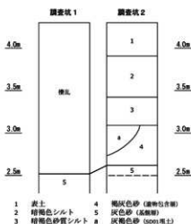
土層柱状図 (S=1/40)
