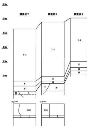
土層柱状図 (S=1/40)
