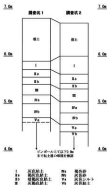
土層柱状図 (S=1/40)
