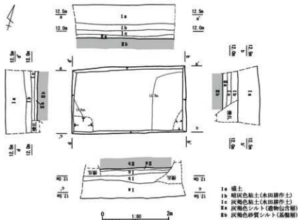
第18図 C区平面図及び土層断面図
