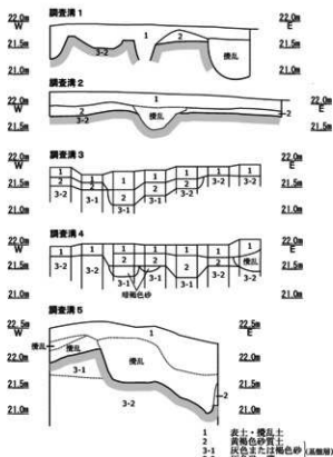
土層柱状図 (S=1/80)
