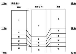
土層柱状図 (S=1/40)
