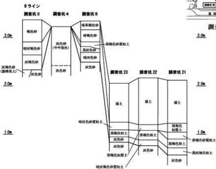
土層柱状図 (S=1/40)
