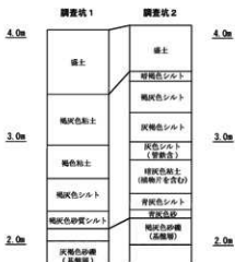
土層柱状図 (S=1/40)
