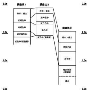
土層柱状図 (S=1/40)
