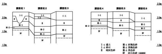
土層柱状図 (S=1/40)
