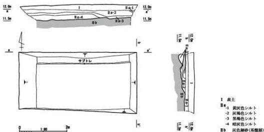
第16図 A区平面図及び土層断面図
