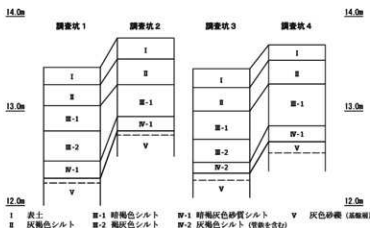
土層柱状図 (S=1/40)
