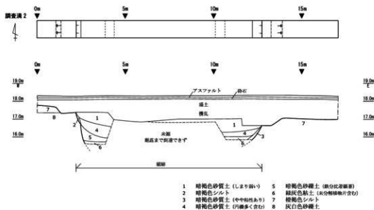
土層断面図 (S=1/150)
