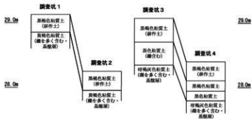
土層柱狀圖 (S=1/40)
