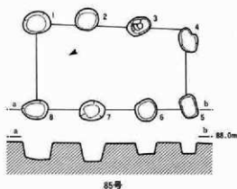
AII④ (長辺柱穴 4 本)
