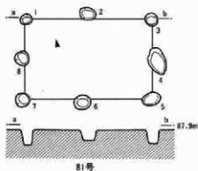
BII (長辺柱穴 3 本)
