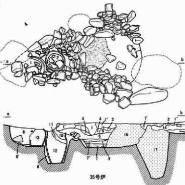
35号炉 炉体1
