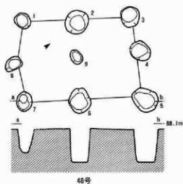
(長辺柱穴 3 本・東柱有)
