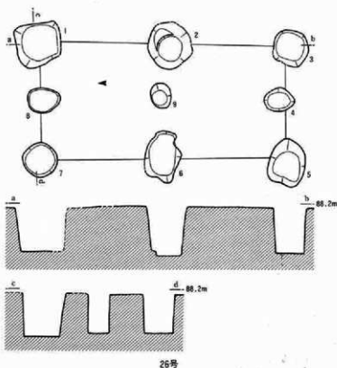
(長辺柱穴 3 本・束柱有)
