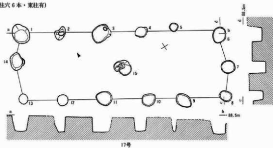
BN⑧ (長辺柱穴6本・東柱有)
