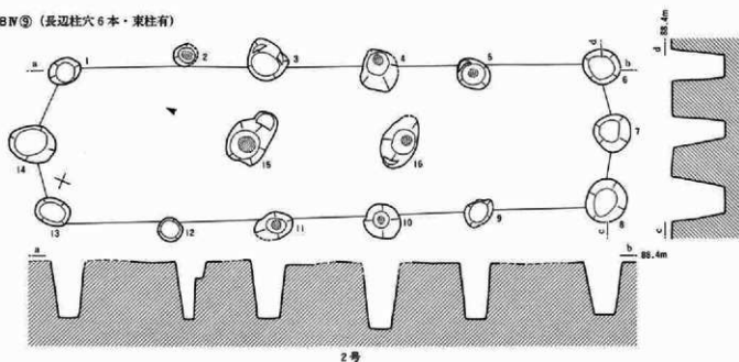
(長辺柱8本・束柱有)
