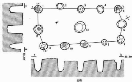
BIV⑦ (長辺柱穴5本・東柱有)
