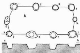
(長辺柱穴4本・東柱有)
