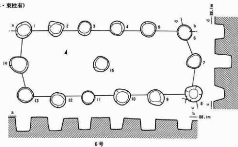
(長辺柱穴6本・東柱有)
