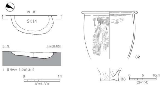
第44図 SK14 測量図・出土遺物実測図
