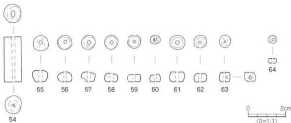
第51図 1号石室出土遺物実測図(2)
