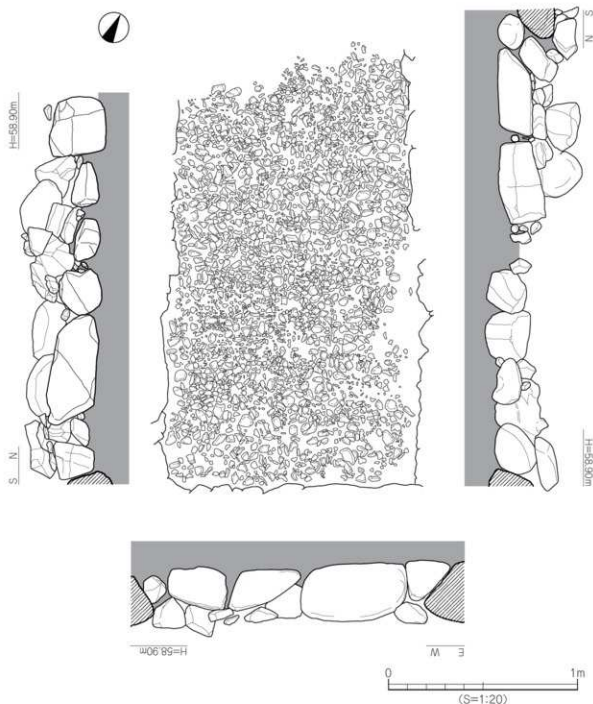
第 55 図 2 号石室展開図
