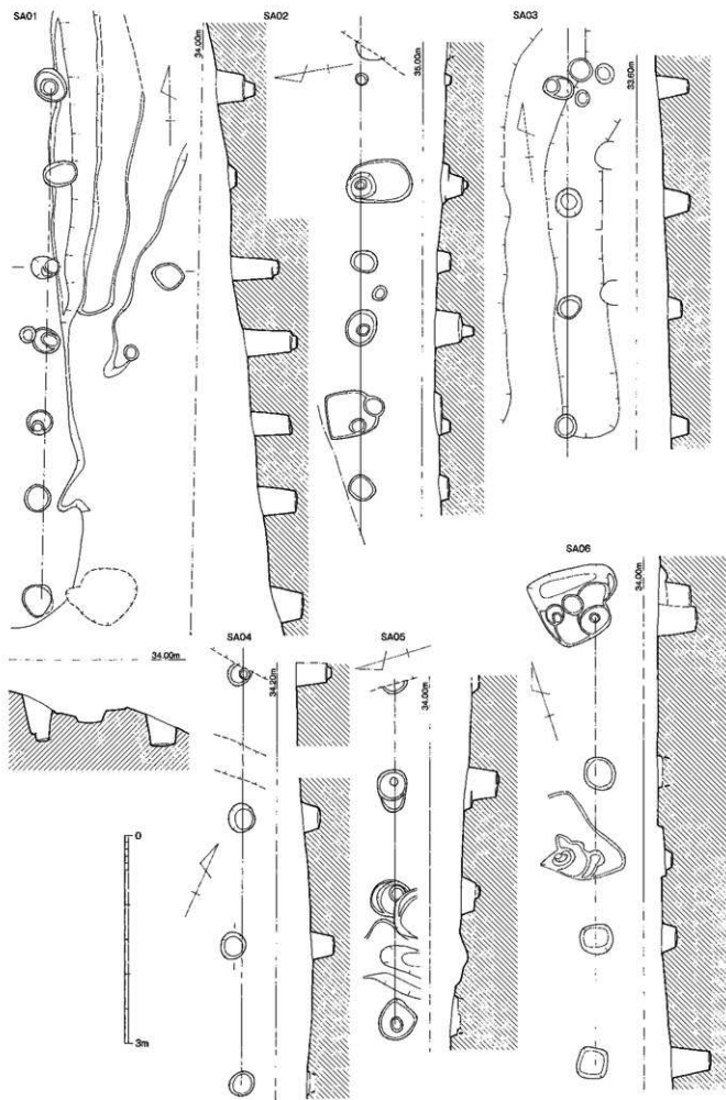
第 16 图 欄 SA01 ~ 06 実測図 (1/60)
