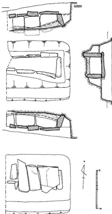
第5图 第3号石棺墓实测图
