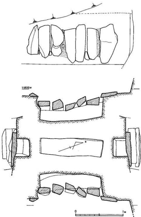
第7圖 第5号石室土塚墓実測図
