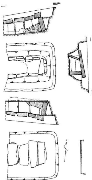
第4図 第2号石棺墓実測図
