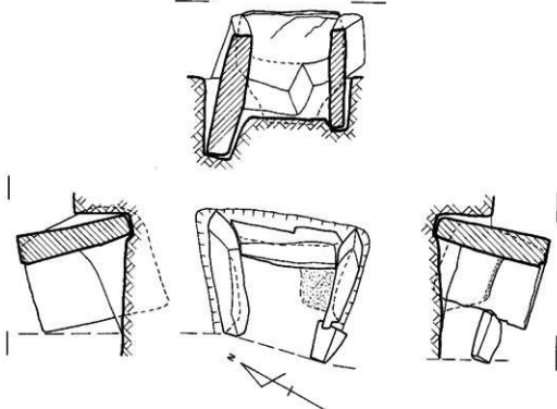
第3図 第1号石棺墓実測図
