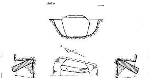
第8図 第6号石棺墓実測図
