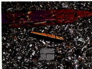
1. 試料番号1: カミングトン閃石含有黒雲母角閃石安山岩 (平成17年度 遺物番号35 台帳番号221 石皿)
