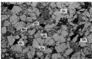
9. 試料番号 9 て-93 4 磨石兼融石 中粒砂岩
