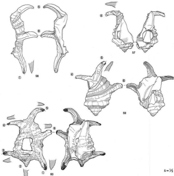
第7図 IV層出土の貝製品(2)
