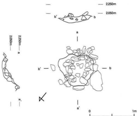
3号集石炉遺構実測図
