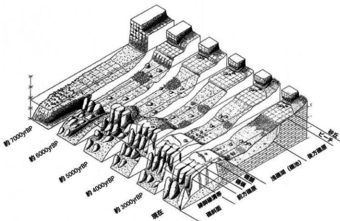
琉球列島における完新世サンゴ礁の形成過程模式図 (米倉ほか, 2001)
