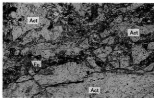
6. 試料番号6 ちー95 III 敲石 緑廉石-アクチノ閃石緑色岩
