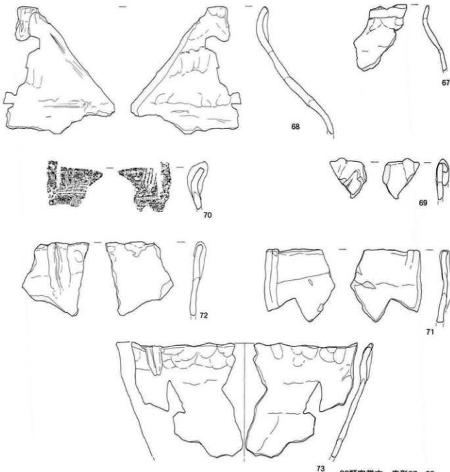
20類突帯文 壺形67・68 突帯文 深鉢形・甕形69~73
