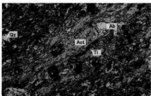
2. 試料番号2 さー100 II 半磨製石斧 緑康石-アクチノ閃石緑色片岩
