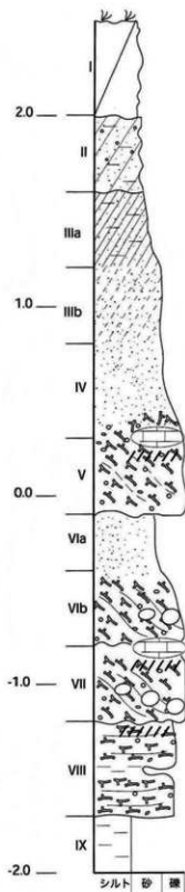
大堂原貝塚における堆積層の模式柱状図
