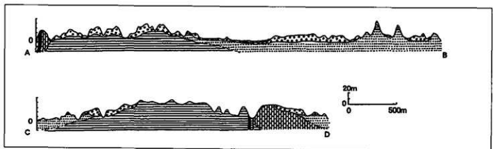
屋我地島地質断面図 (神谷厚昭)
