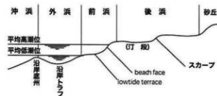
砂浜海岸の縦断形（松田ほか編（1981）に加筆）
