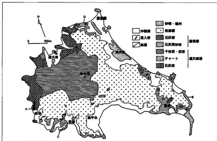
屋我地島の地質図（神谷厚昭）
