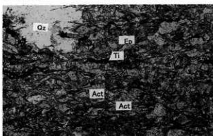
10. 試料番号 10 て-93 4 磨石 緑黒石-アクチノ閃石緑色片岩
