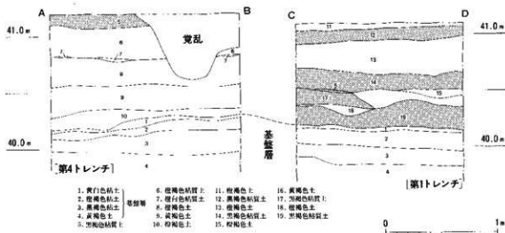
第7図 第1・4トレンチ墳丘断面実測図 (1/30)
