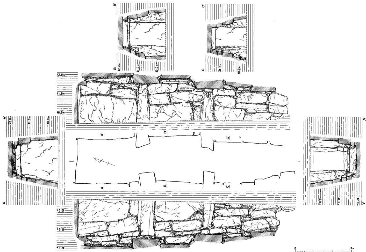
第10图 伊方古墳石室実測図 (1/60)
