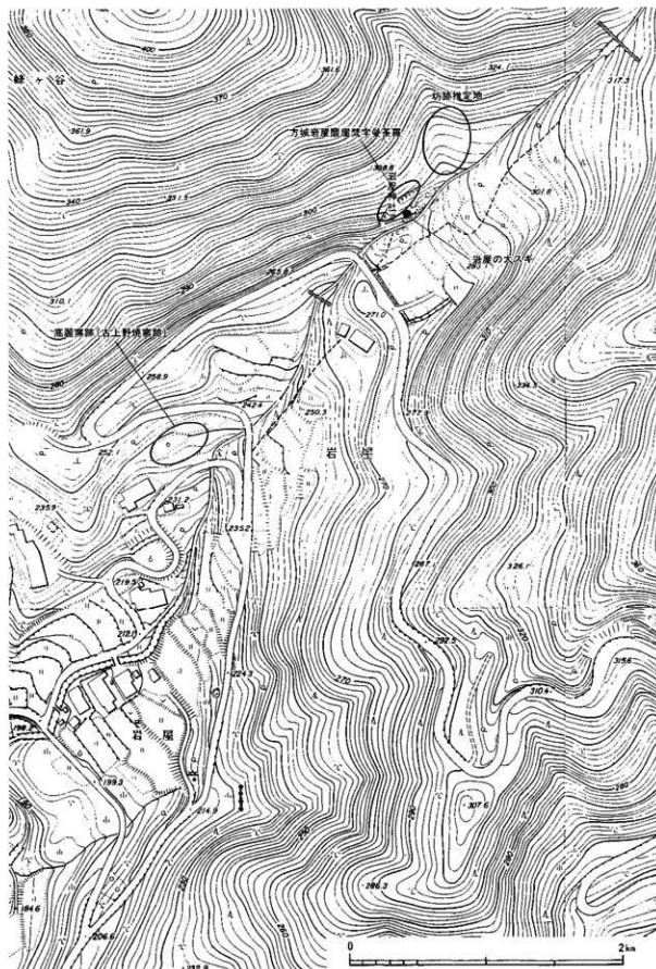
第11図 方城岩屋跡麓麓字受茶羅岡辺地形図 (1/2,000)
