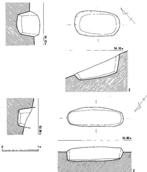
第17図 2・3号土壇墓実測図 (1/30)
