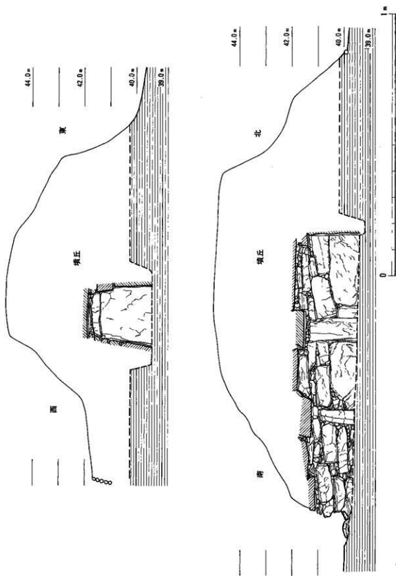
第6图 伊方古墳墳丘断面图 (1/100)
