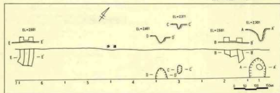
図-7 遺構実測図
