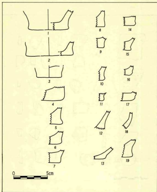
图-9 土器实测图・底部
