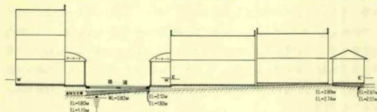
図-3 W-W'・E-E'断面図
