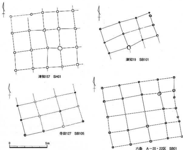
第31図 市内既往遺跡の関連独立柱建物 平面プラン (1/160) [出典:本書および各報告書から]
