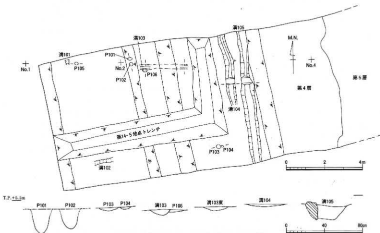
第8図 第1遺構面 平面図（1/100）、遺構断面図（1/20）
