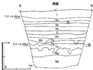
第7図 深掘トレンチ 土層断面図 (1/40)
