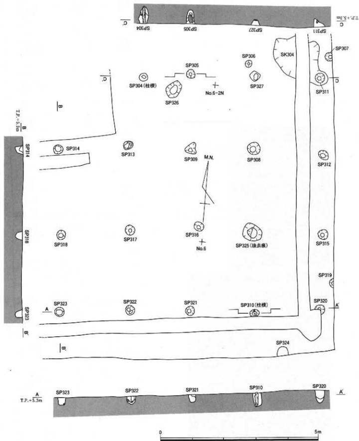
第24図 第3遺構面 獨立柱建物 (1/60)
