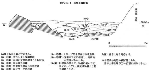
第7図 セクションベルト1土層断面図 1/50
