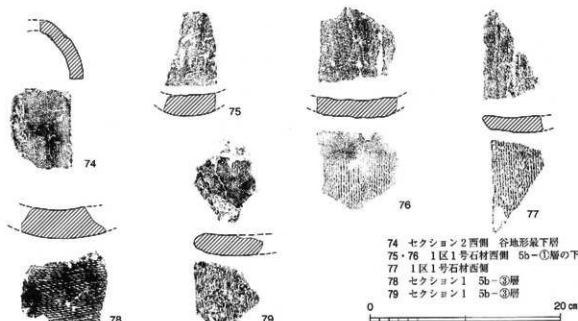
第18図 包含層出土瓦実測図 1/4
