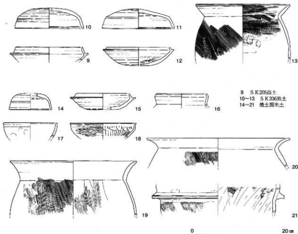
第15図 遺構面2出土遺物実測図 1/4
